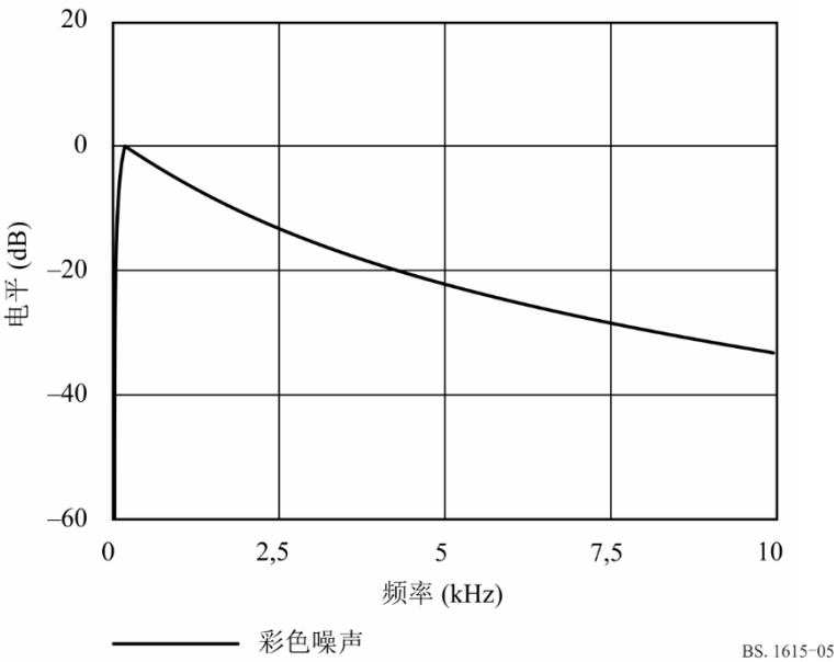
图 5 噪声整形滤波器的特性
