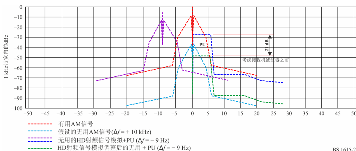
受IBOC混合信号模拟+ PU（-9 kHz）干扰的有用调幅信号
