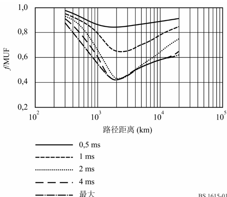
图 1 多径延迟时间
