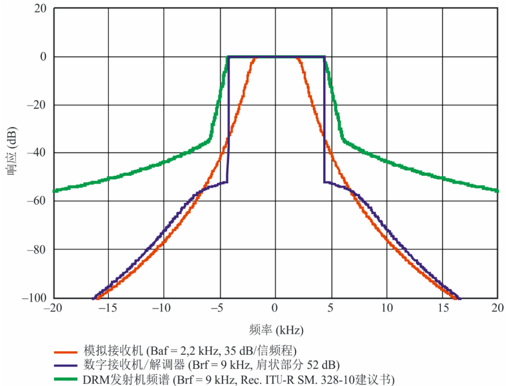
图 16 2001年的频谱掩模
