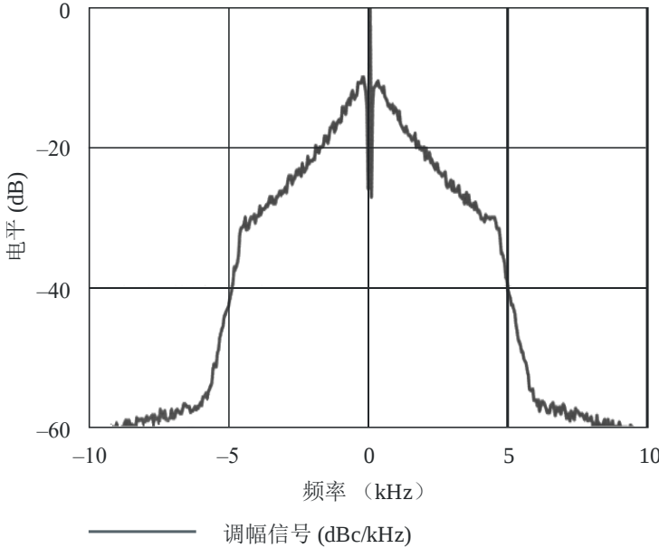
图 8 与有色噪声调制的调幅信号
