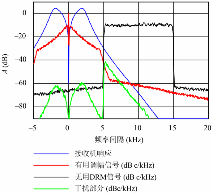
图 10b DRM信号干扰调幅信号
