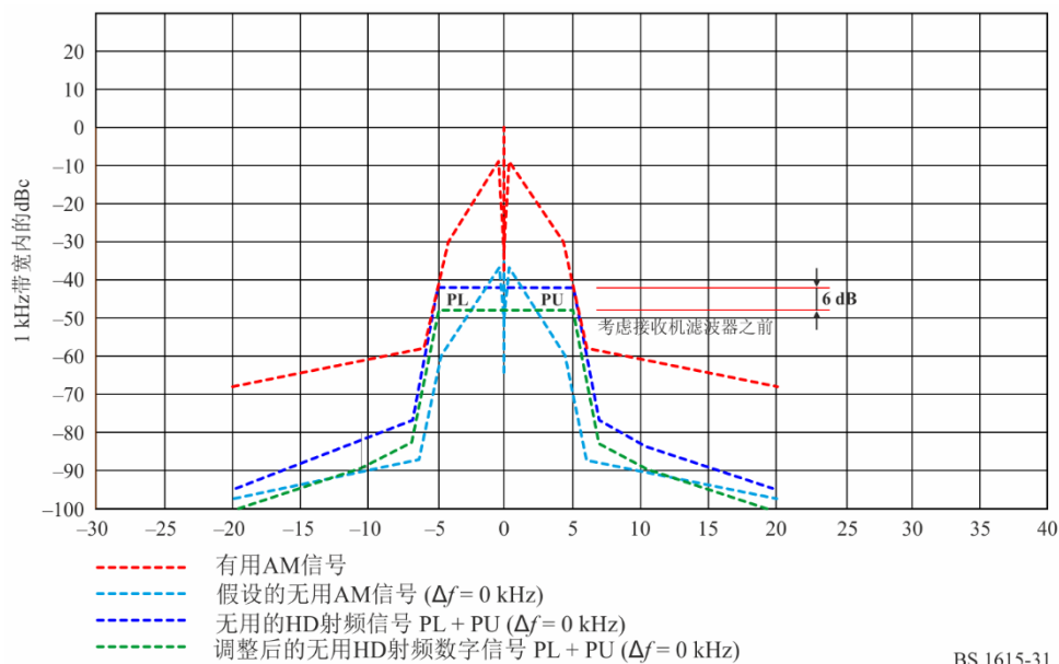
受10 kHz带宽IBOC数字信号干扰的有用调幅信号（0 kHz）
