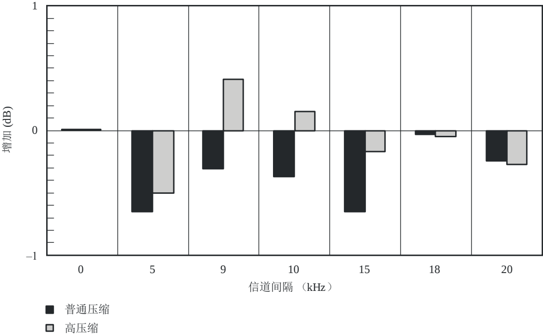
图 15 调幅干扰调幅的射频保护比的计算误差
