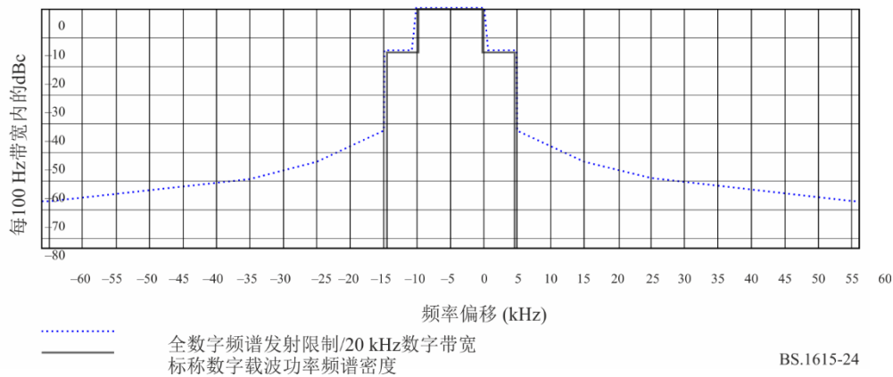
IBOC混合信号频谱和数字信号发射掩膜 – 模式MA3，使用20 kHz带宽
