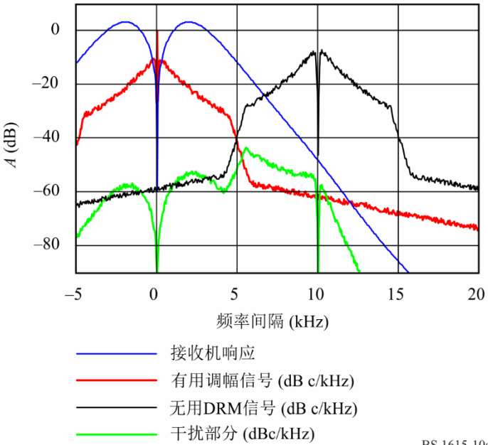
图 10a 调幅信号干扰调幅信号
