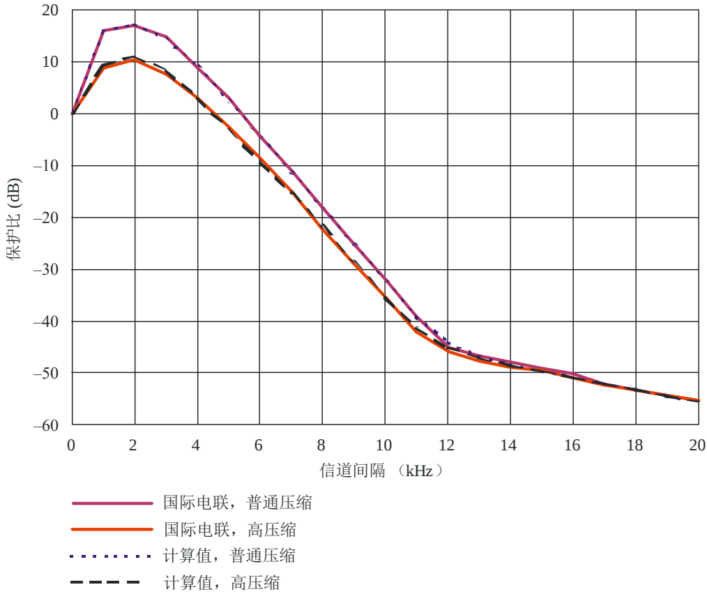
图 14 调幅干扰调幅的相对射频保护比
