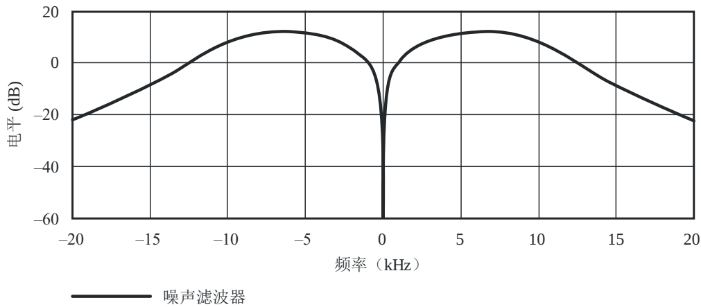
噪声滤波器的信号整形
