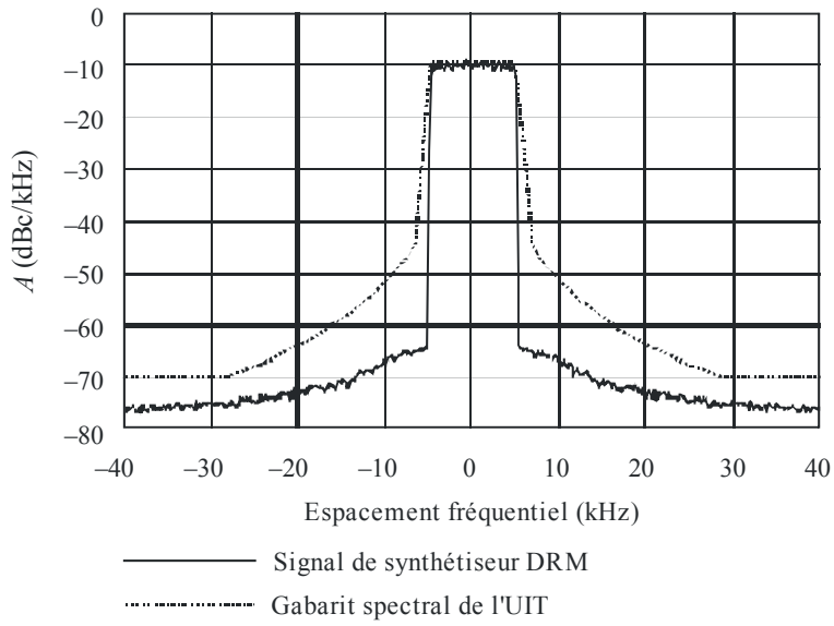
Signal de synthétiseur DRM (MAQ-64, 9 kHz) et gabarit spectral de l'UIT
