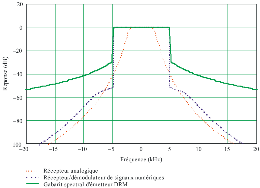
Gabarit spectral de la Recommandation UIT-R BS.1615
