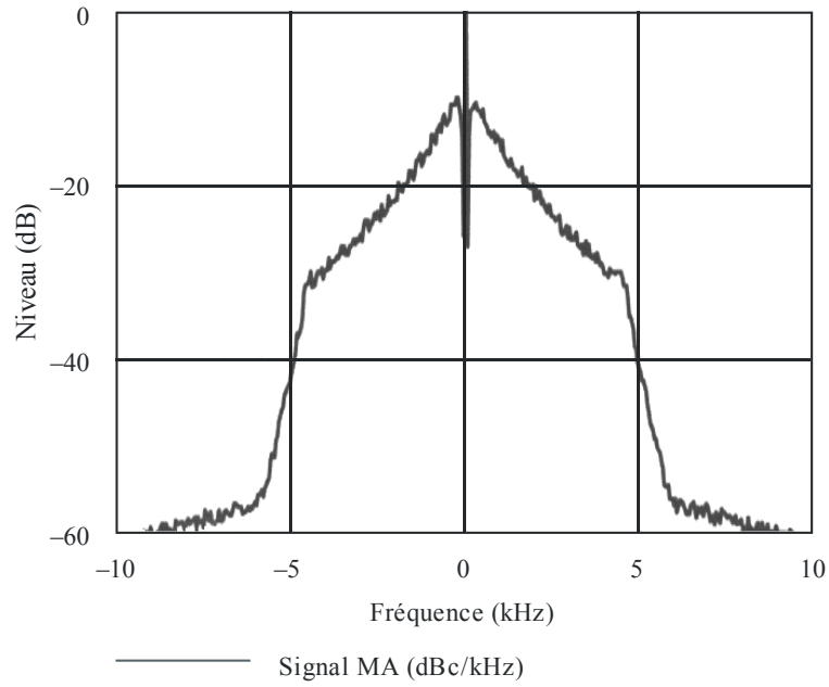
FIGURE 8 Signal MA modulé avec du bruit coloré
