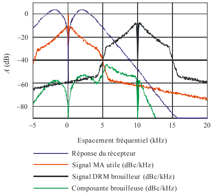
Signal MA brouillé par un autre signal MA
