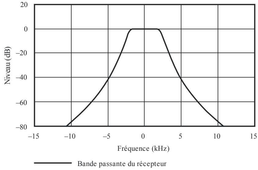
Courbe de sélectivité d'un récepteur MA moderne
