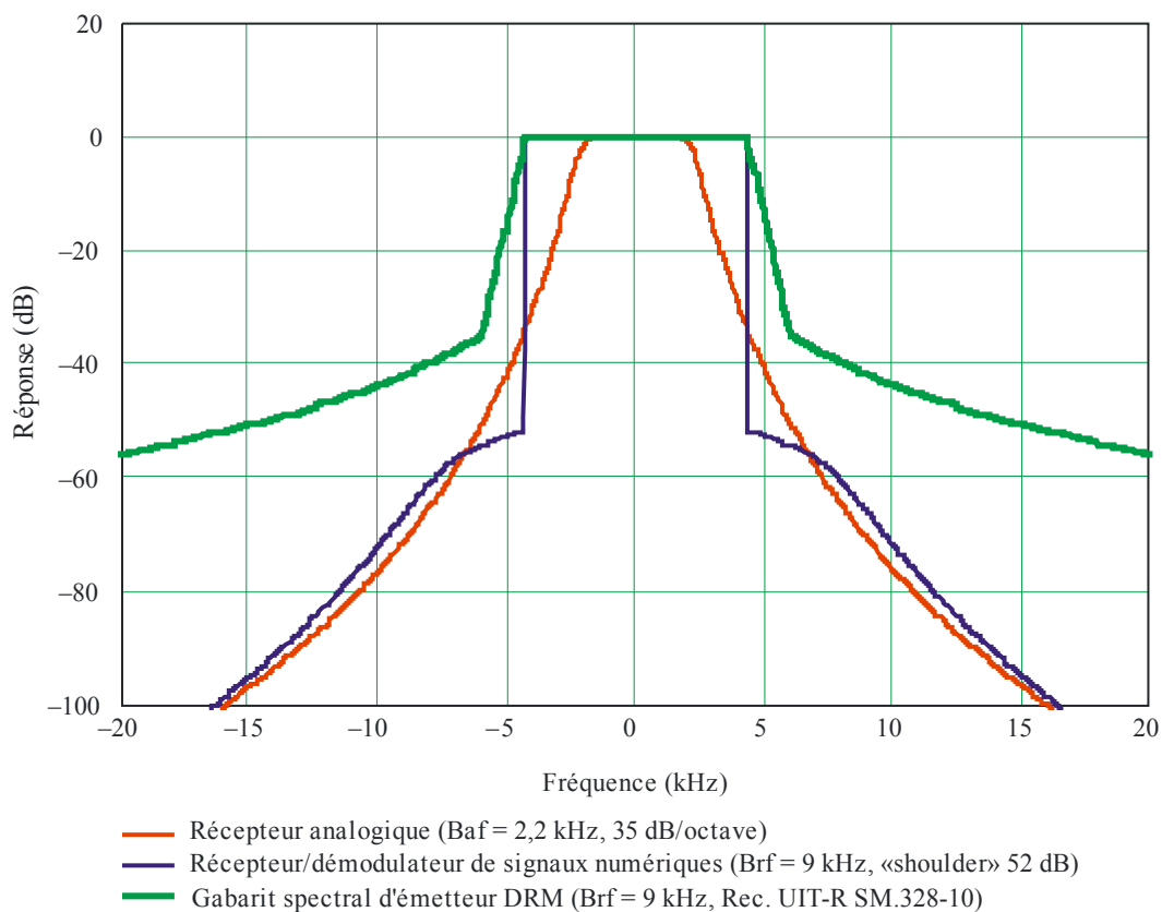
FIGURE 16 Gabarit spectral en 2001
