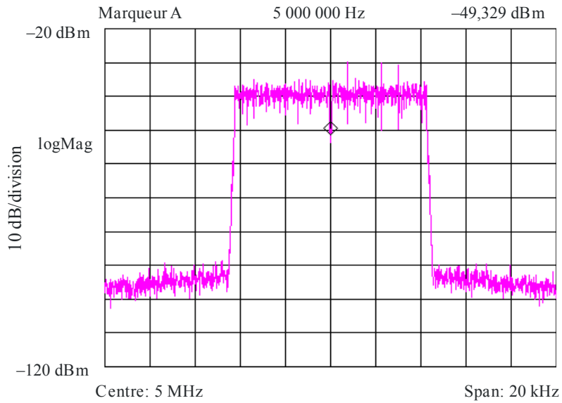
FIGURE 9a Signal de synthétiseur DRM (MAQ-64, 9 kHz)
