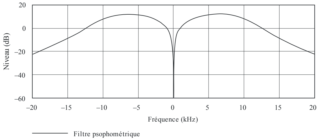
Conformation du signal par un filtre psophométrique
