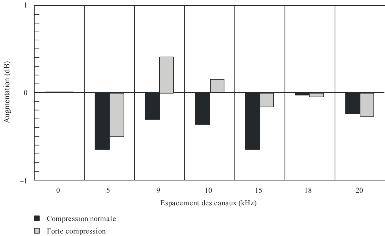
FIGURE 15 Erreur de calcul des rapports de protection RF dans le cas de signaux MA brouillés par d'autres signaux MA
