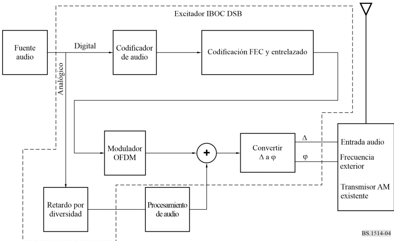
Diagrama de bloques del transmisor del sistema IBOC DSB híbrido en ondas hectométricas
