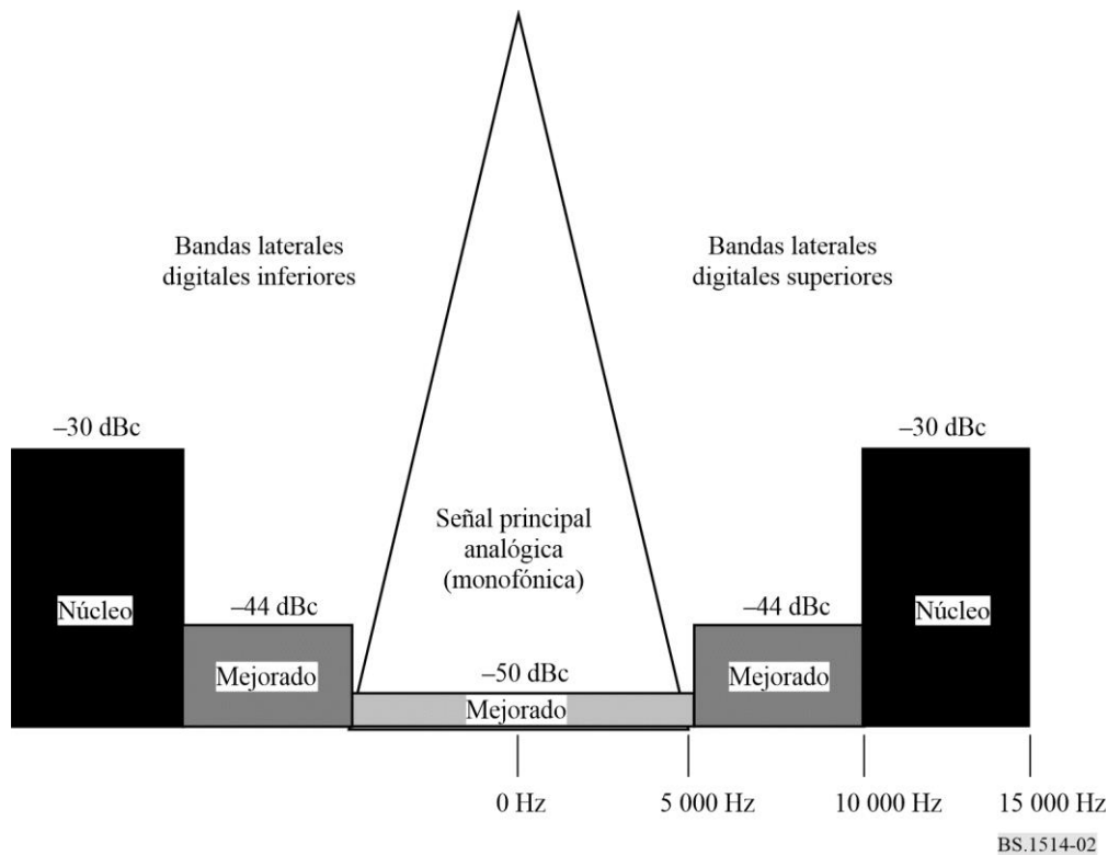
FIGURA 2 Densidad espectral de potencia del sistema IBOC DSB híbrido en ondas hectométricas
