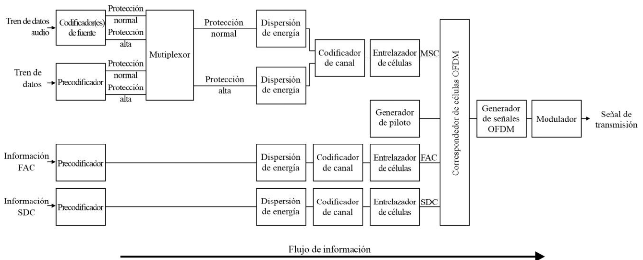
Diagrama de bloques de entrada al transmisor
