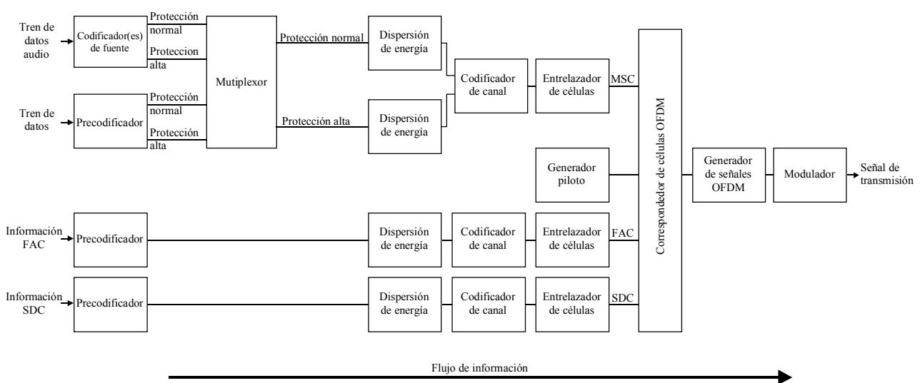
Diagrama de bloques de entrada al transmisor
