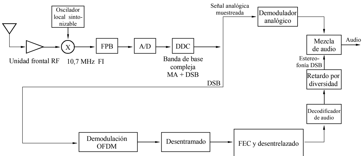
Diagrama de bloques del receptor típico IBOC híbrido en ondas hectométricas
