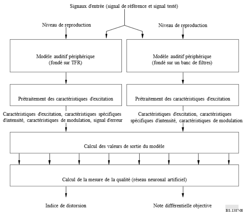
Diagramme générique du système de mesure
