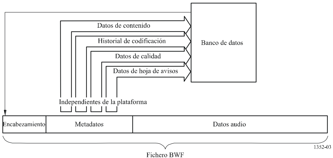
FIGURA 3 Servidor de archivo de recepción para estación de datos de fichero BWF
