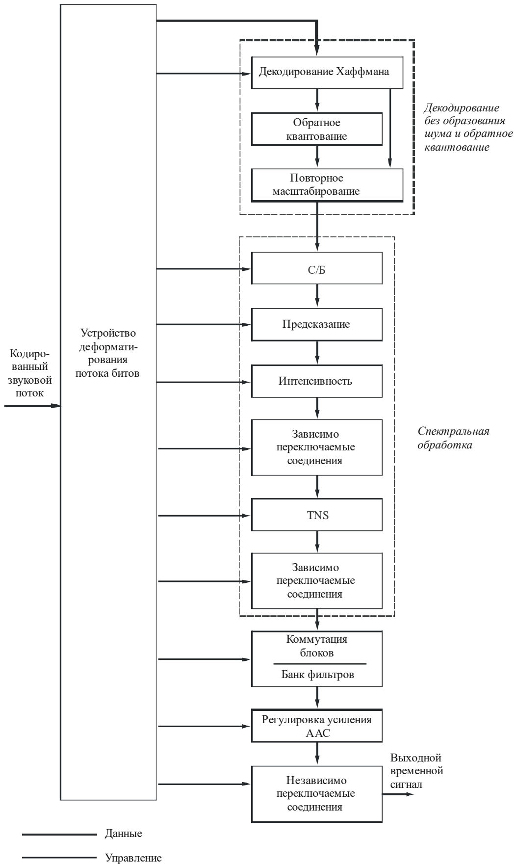
РИСУНОК 6 Функциональная схема декодера AAC MPEG-2
