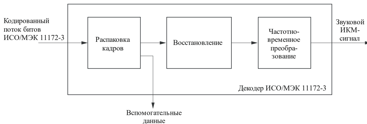
РИСУНОК 4 Блок-схема декодера
