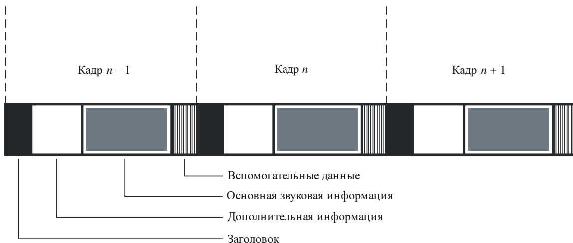
Формат цифрового потока уровня II ИСО/МЭК 11172-3
