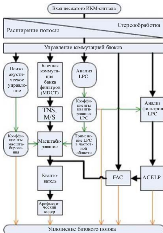
Блок-схема кодера USAC MPEG-D
