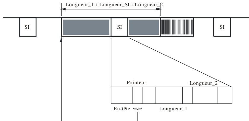
FIGURE 3 Format du train binaire de Couche III ISO/CEI 11172-3
