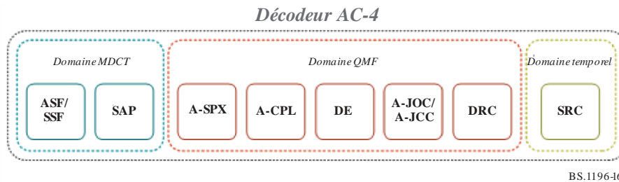
FIGURE 16 Outils de décodage
