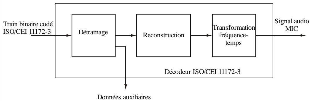
Schéma fonctionnel du décodeur
