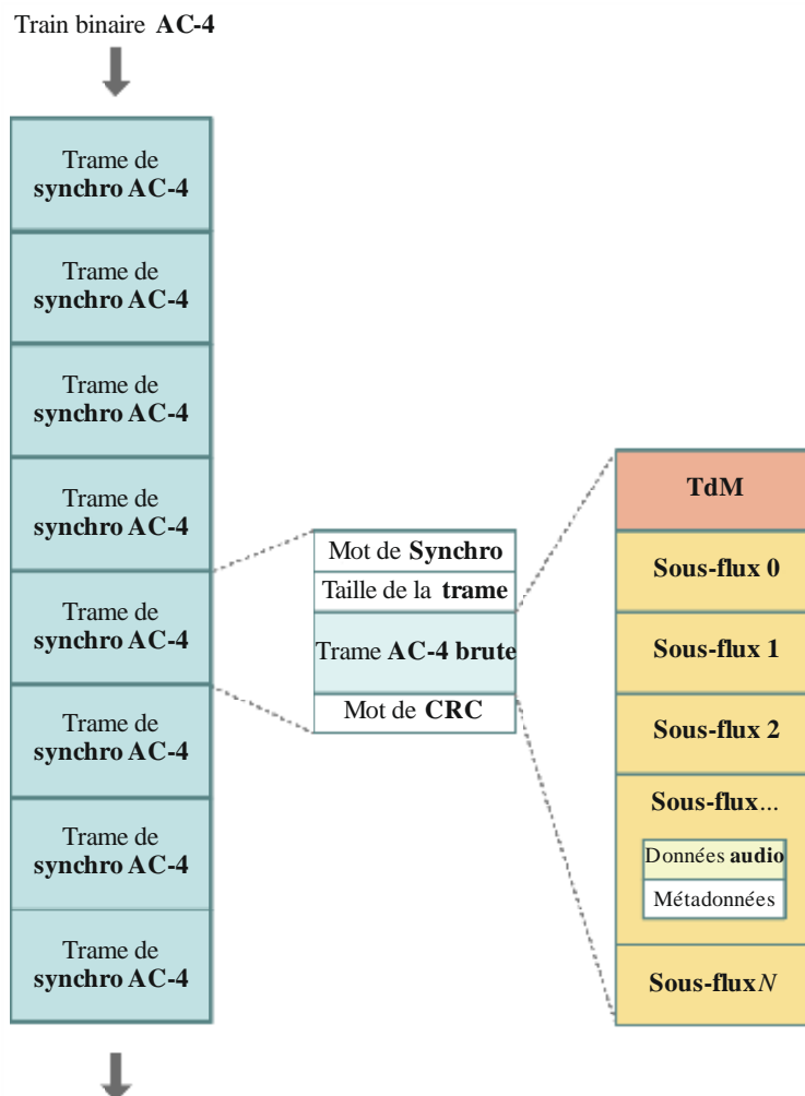
FIGURE 14 Syntaxe du train binaire de haut niveau
