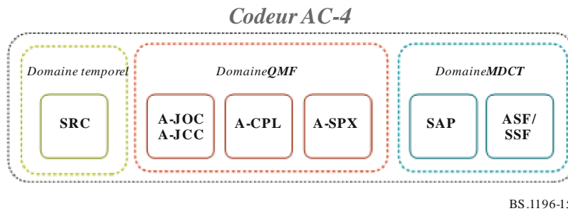
FIGURE 15 Outils de codage disponibles dans le système AC-4
