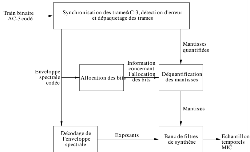
FIGURE 8 Décodeur AC-3
