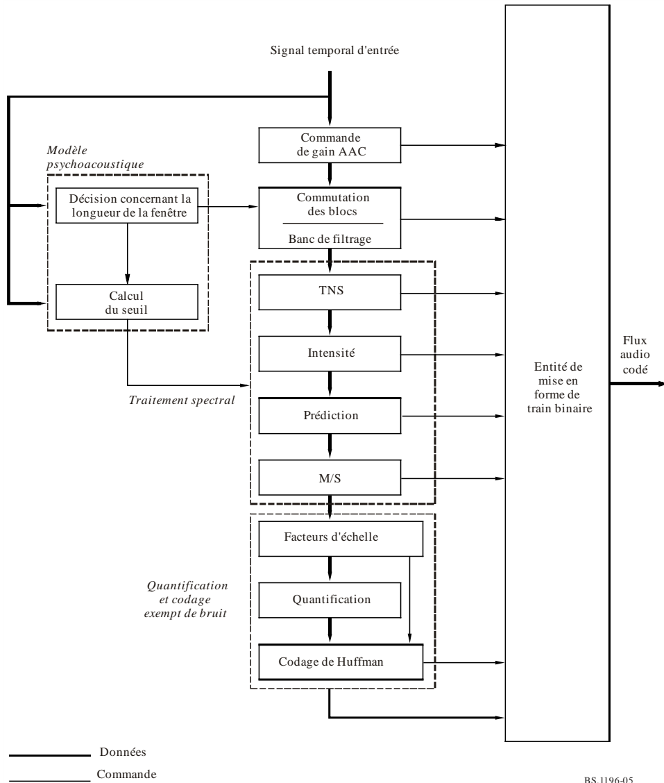
FIGURE 5 Schéma fonctionnel d'un codeur MPEG-2 AAC
