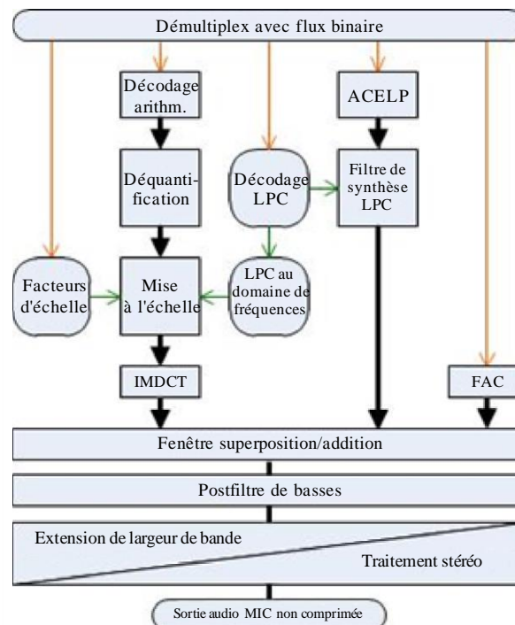
FIGURE 13 Schéma fonctionnel d'un décodeur MPEG-D USAC
