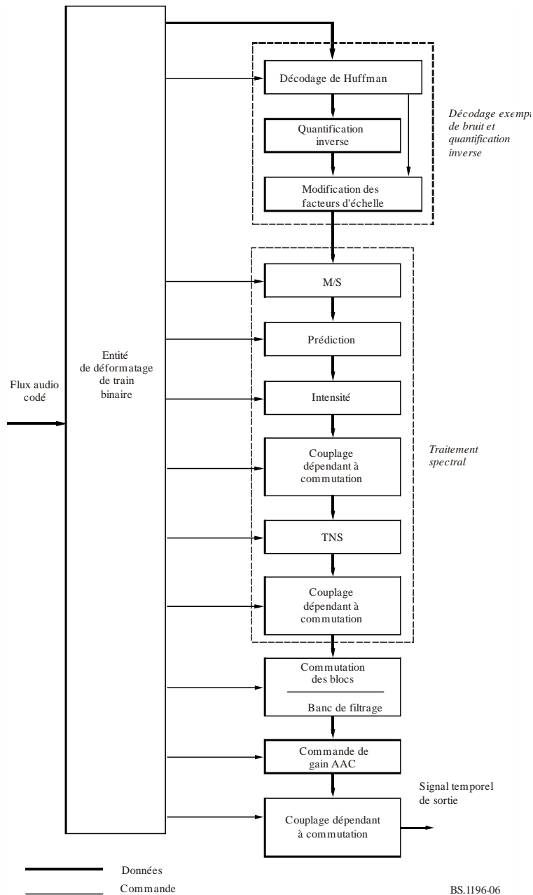
Schéma fonctionnel d'un décodeur MPEG-2 AAC
