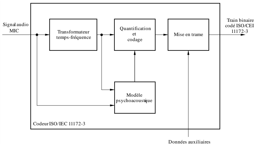
Schéma fonctionnel d'un codeur type
