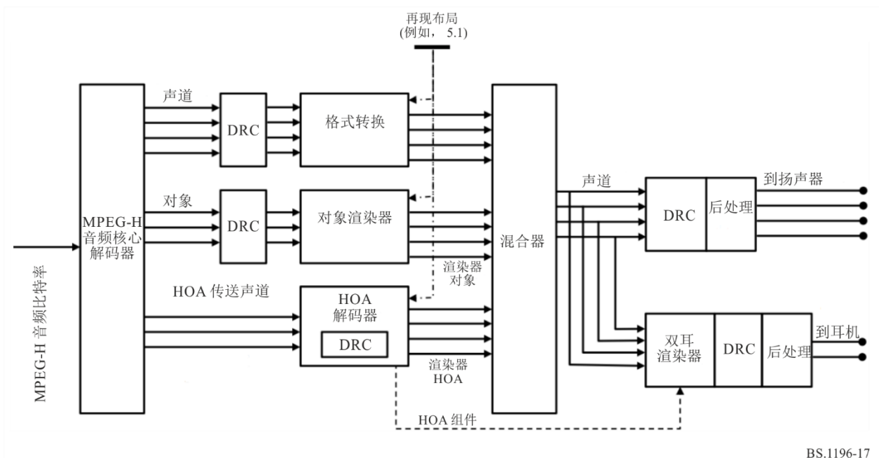
低复杂度型MPEG-H 3D音频解码器体系结构的顶层方框图
