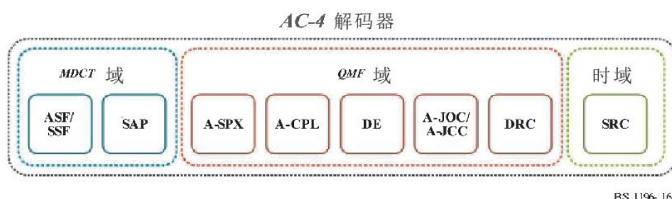
图16 解码工具
