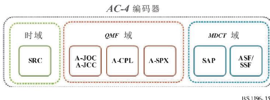
图15 AC-4系统中可用的编码工具
