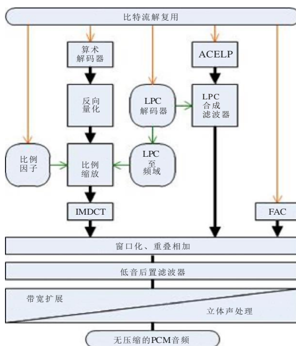
MPEG-D USAC解码器的方框图
