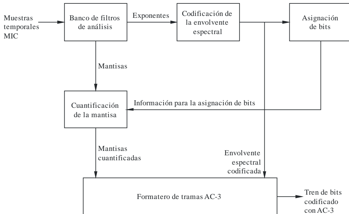
FIGURA 7 Codificador AC-3
