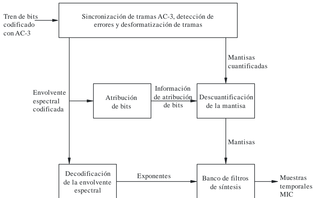
FIGURA 8 Decodificador AC-3
