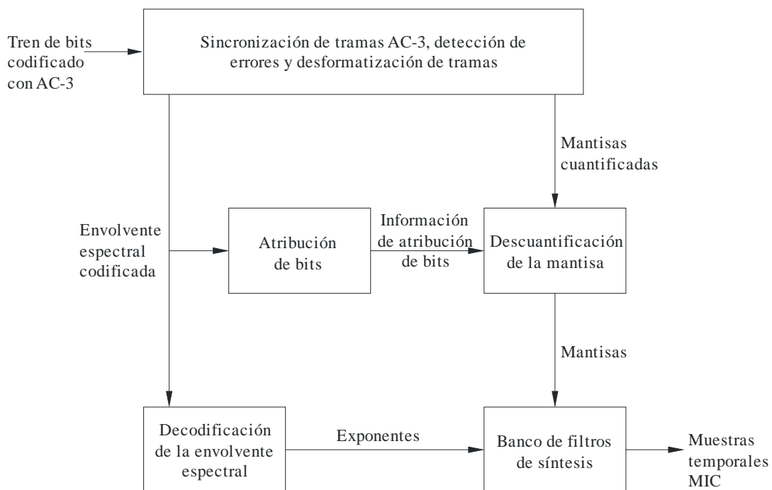
FIGURA 8 Decodificador AC-3
