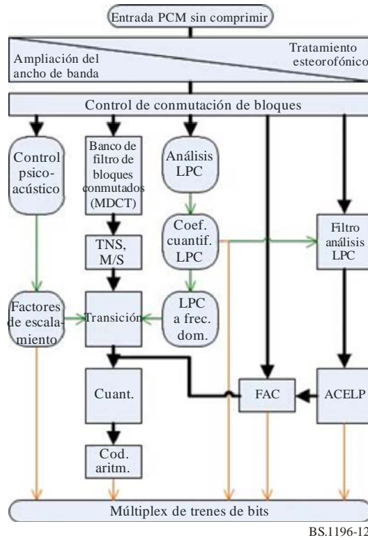
Diagrama de bloque del codificador MPEG-D USAC
