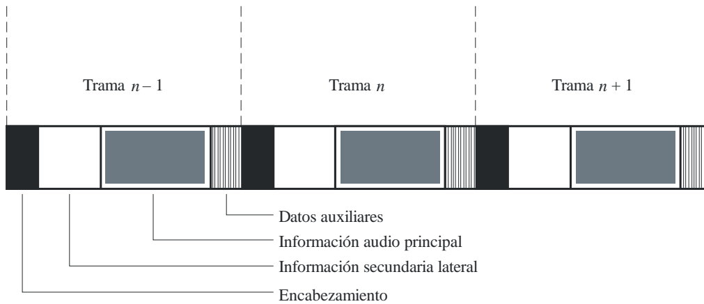
FIGURA 2 Formato del tren de bits ISO/CEI 11172-3 de Capa II
