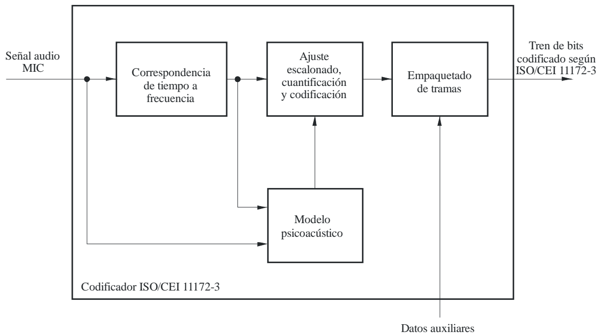
Esquema de bloques de un codificador típico
