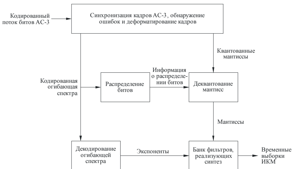
РИСУНОК 8 Декодер АС-3
