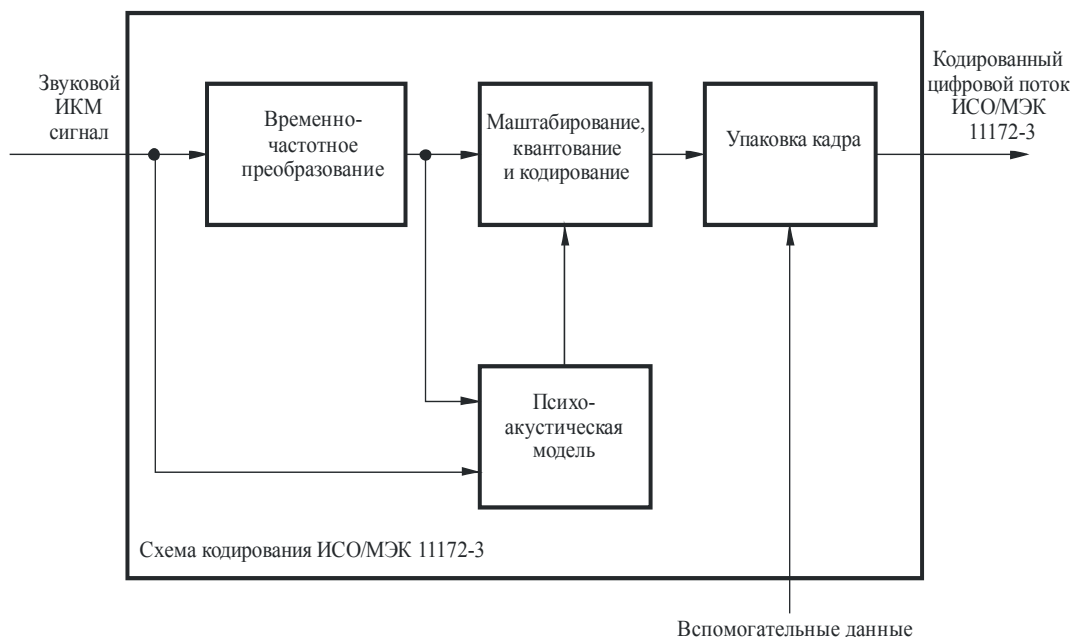
РИСУНОК 1 Блок-схема типового кодера
