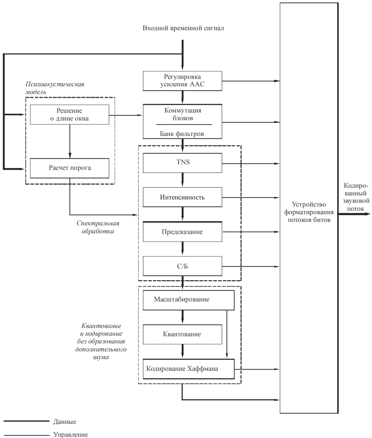
РИСУНОК 5 Функциональная схема кодера AAC MPEG-2
