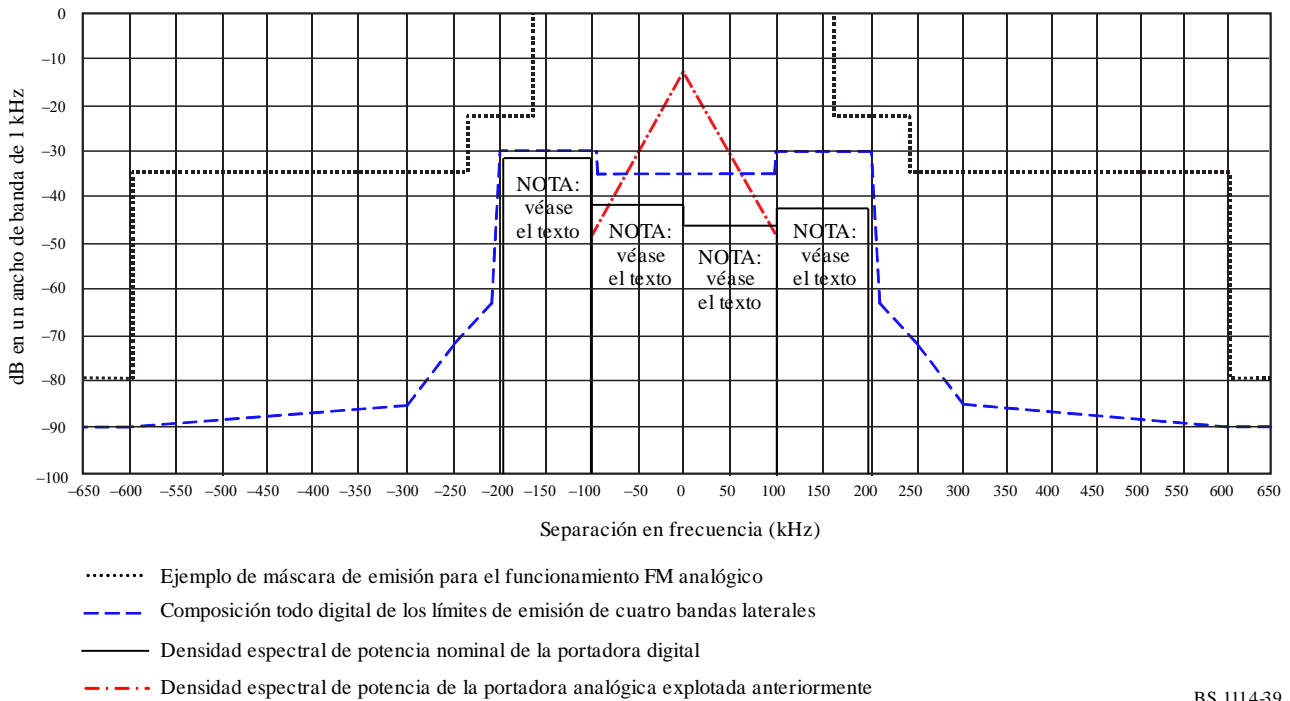
FIGURA 39 Límites de la emisión plenamente digital*
