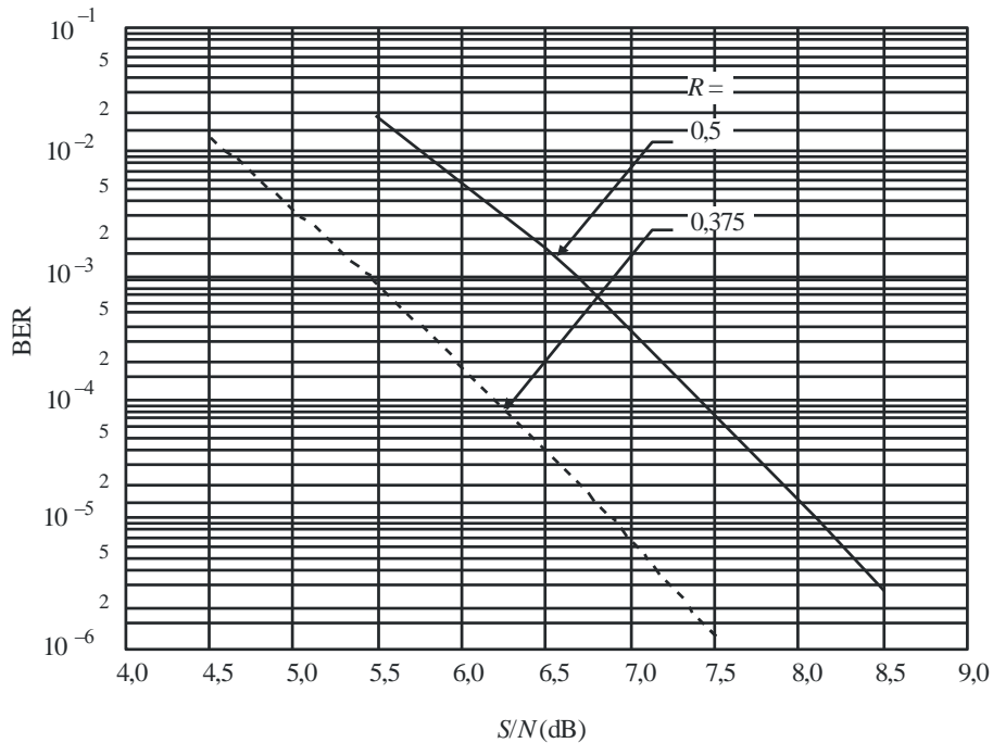
FIGURA 9 BER en función de la relación S/N para el Sistema A (Modo de transmisión II o III): canal gaussiano
