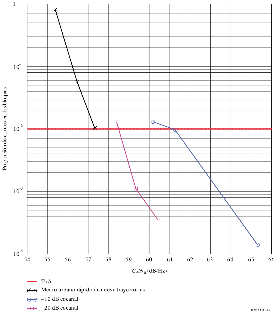
FIGURA 43 Resultados de la proporción de errores en los bloques de un sistema híbrido con una fuente de interferencia de diez canales de desvanecimiento independiente
