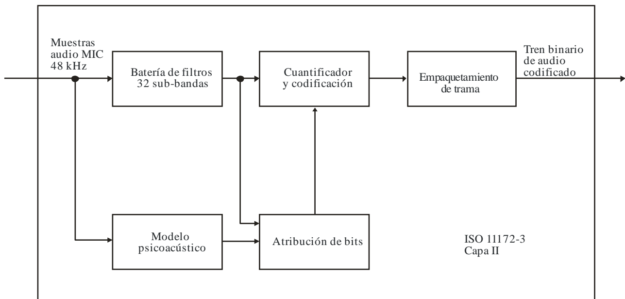
Diagrama de bloques del sistema básico del codificador de audio
