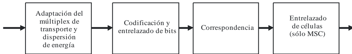
Diagrama de bloques funcional de la codificación y el entrelazado
