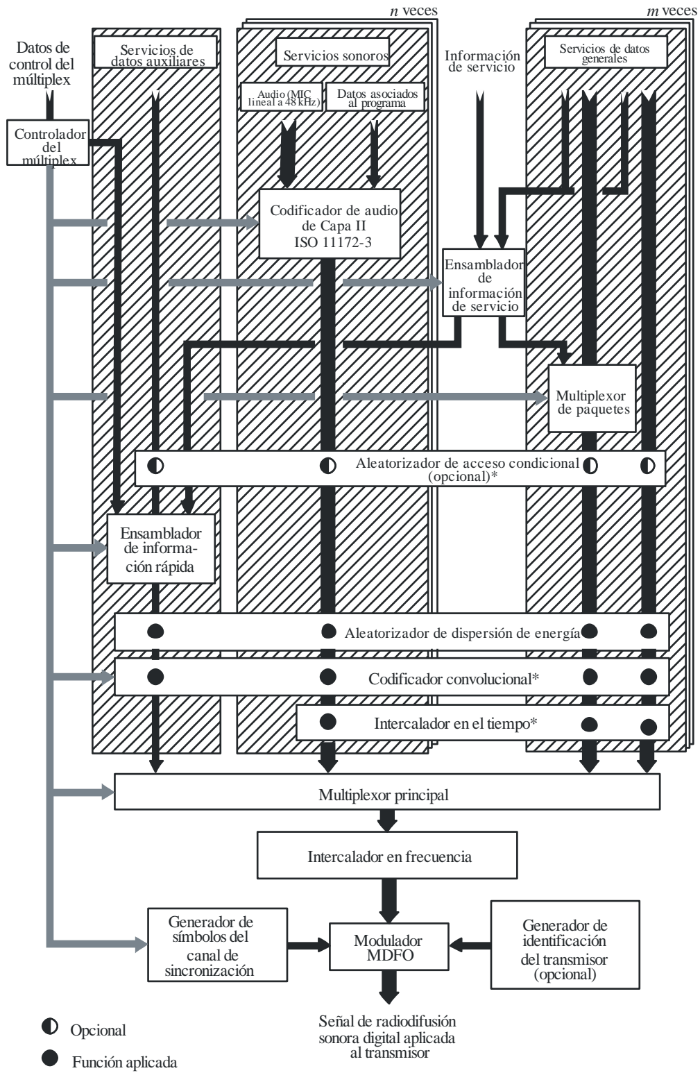
Diagrama conceptual de la parte de transmisión del Sistema A
