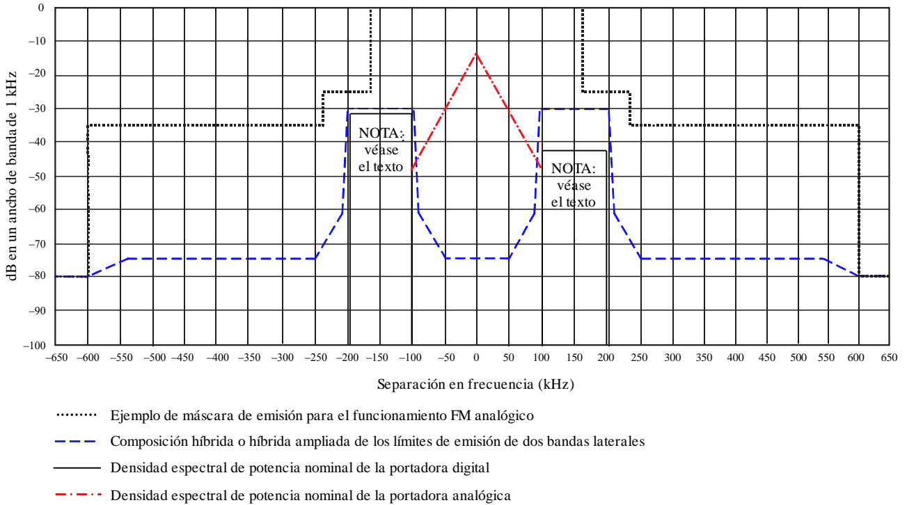
Límites de la emisión en modo híbrido IBOC*
