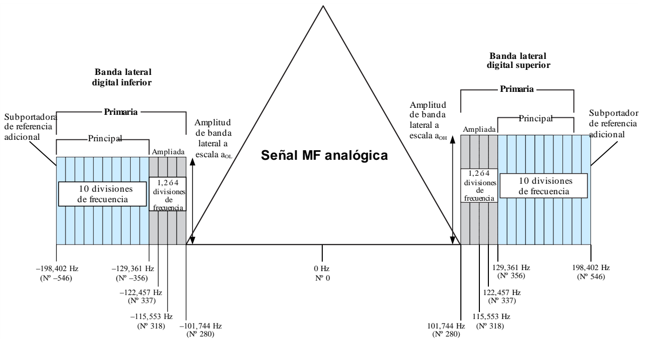
Espectro de la forma de onda híbrida ampliada – Modos de servicio MP2, MP3, MP11, MP12, MP5 y MP6
