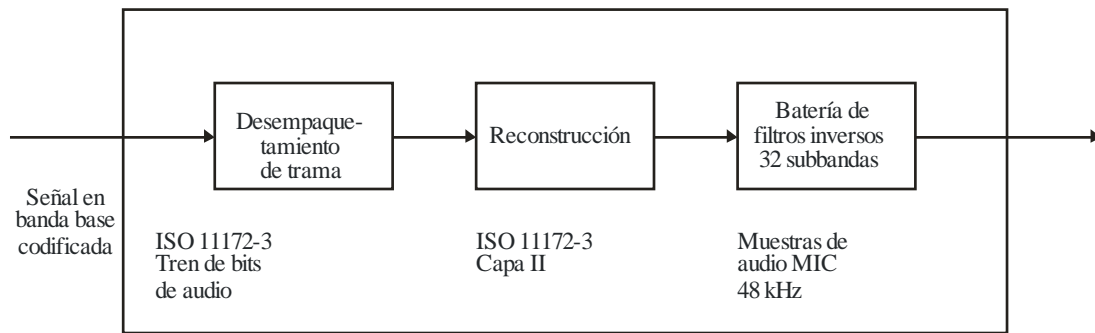
Diagrama de bloques del sistema básico del decodificador de audio
