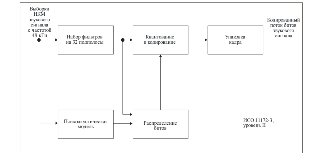
Блок-схема основного аудиокодера системы
