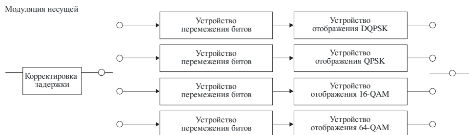
РИСУНОК 20 Конфигурация блока модуляции несущей
