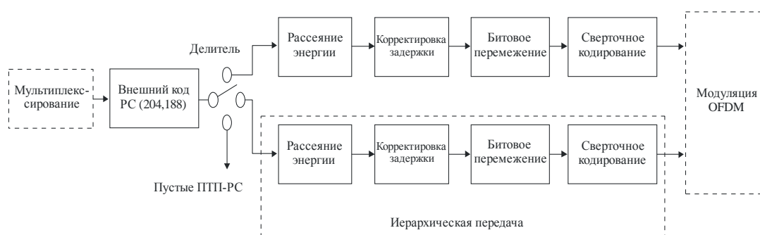
Схема кодирования канала
