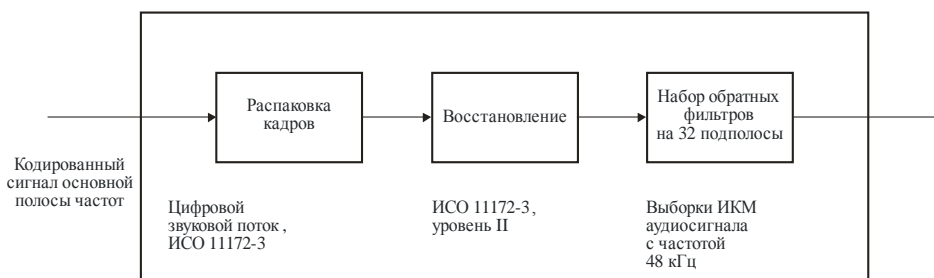
Блок-схема основного звукового декодера системы
