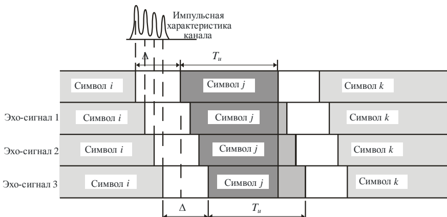
Усиливающее влияние эхо-сигналов
