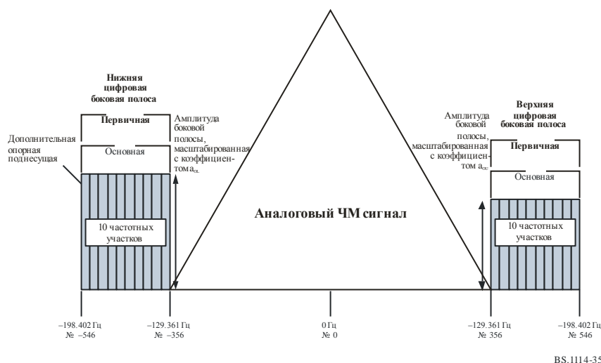
Спектр гибридной волны – режим обслуживания МР1
