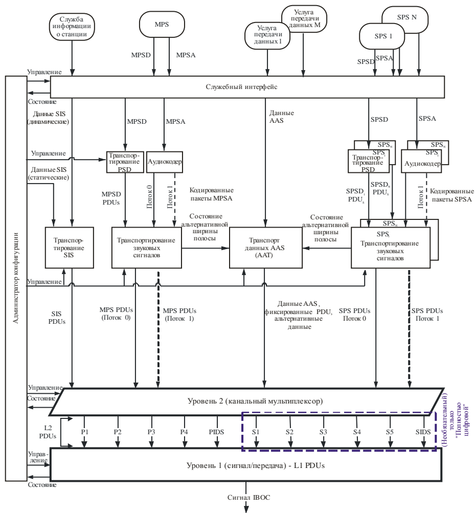
РИСУНОК 29 Блок-схема стека протокола ЧМ-системы ИВОС
