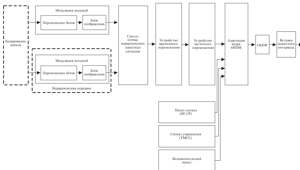
РИСУНОК 19 Блок-схема модуляции
