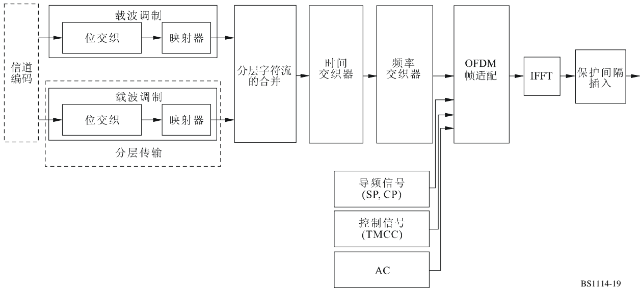
图 19 调制方框图
