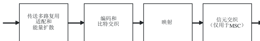
图 46 编码和交织功能框图
