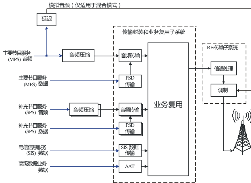
IBOC广播系统概述
