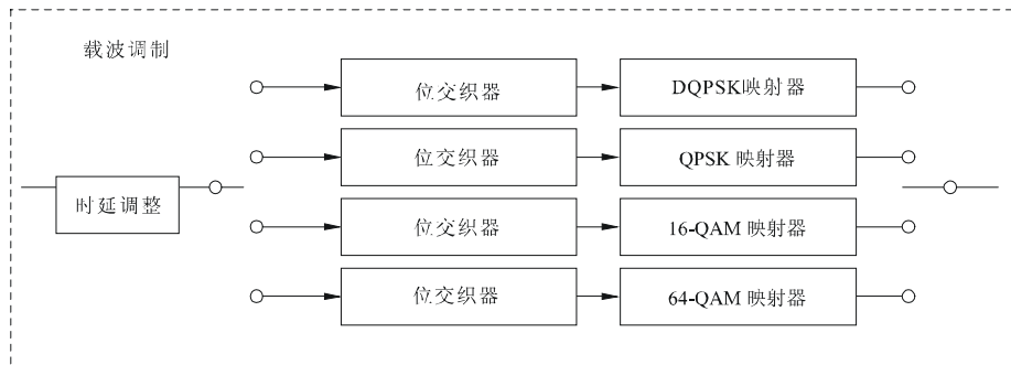
图 20 载波调制单元的配置
