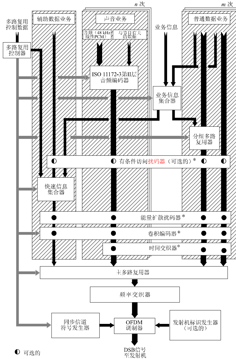
图1 系统A发送部分的概念图
