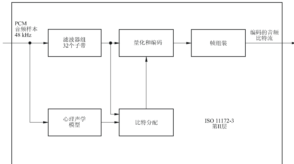
图2 基本的系统音频编码器框图
