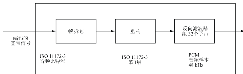
图3 基本的系统音频解码器框图
