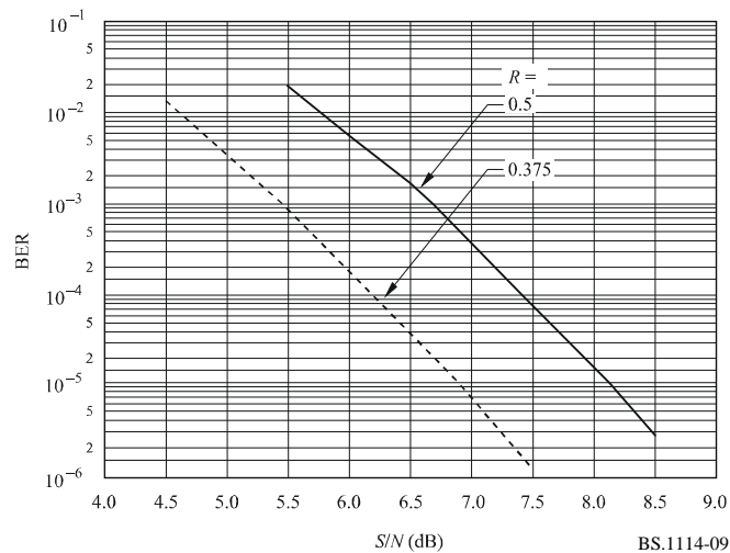
系统A的BER对比S/N (传输模式II或III)：高斯信道
