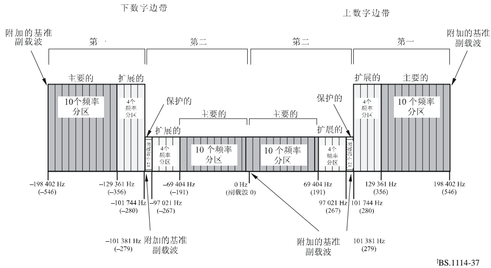
全数字波形的频谱 – 服务模式MP5、MP6和MP12、MS1到MS4
