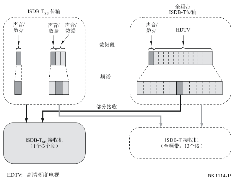
ISDB-T SB 和全频带ISDB-T传输概念和它的接收
