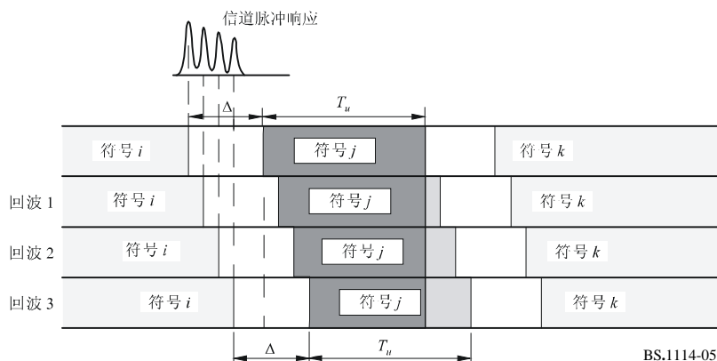
回波的积极作用
