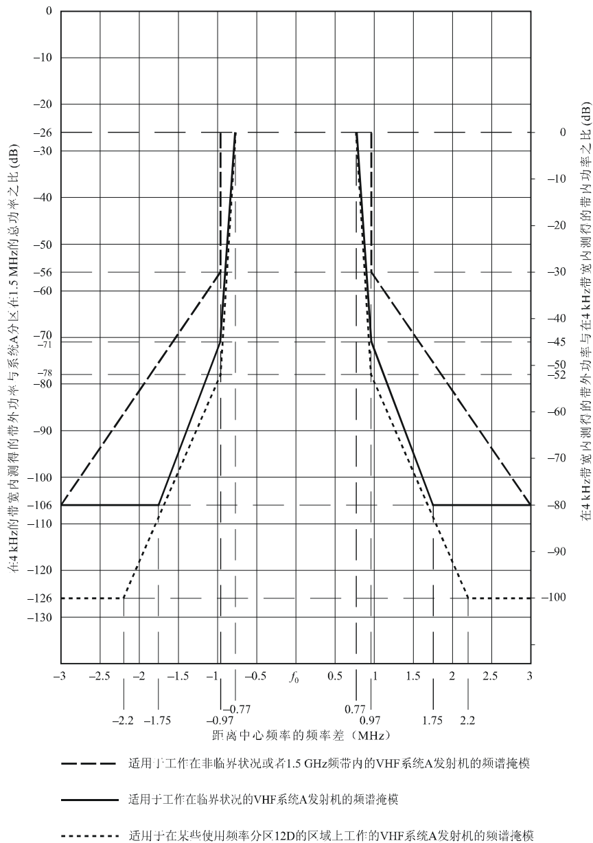
系统A传输信号的带外频谱掩模
