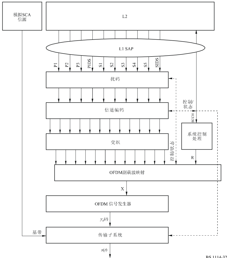
FM空中接口L1功能框图
