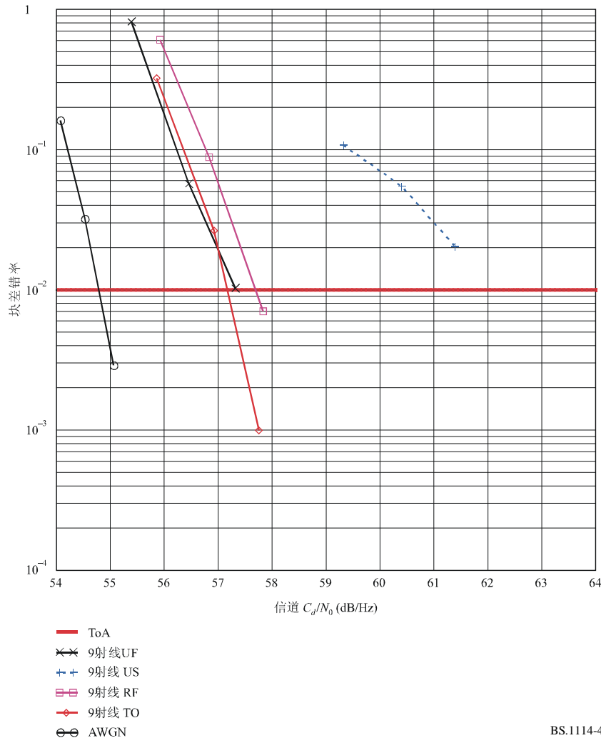
图 41 混合系统在不同类型的9射线衰落和加性高斯白噪声 (AWGN) 情况下的块错误率结果
