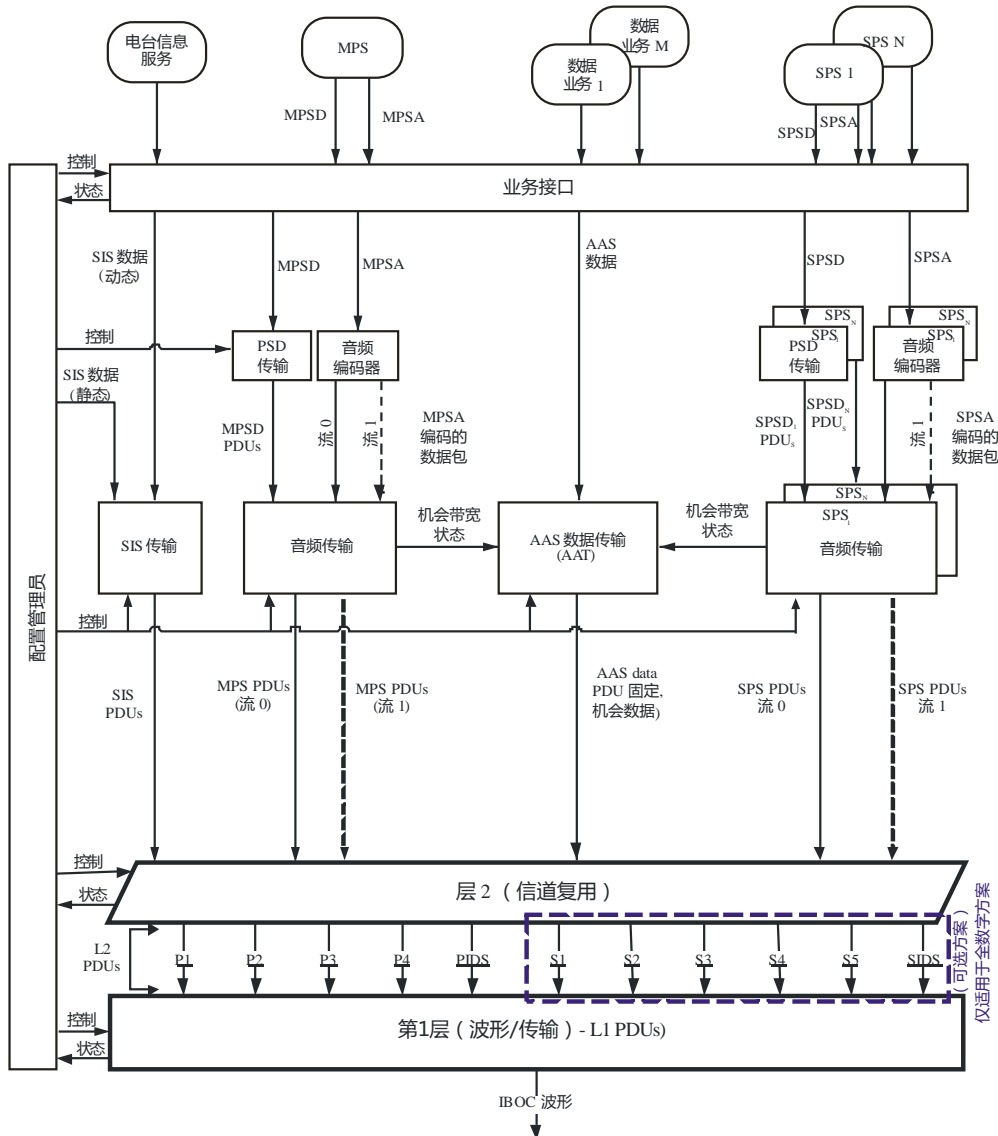
IBOC FM系统协议栈模块图
