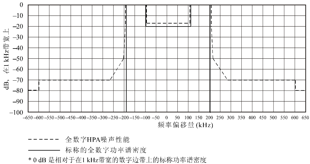
全数字发射限制
