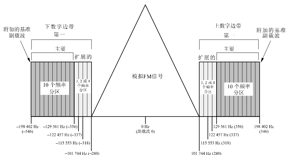
扩展的混合波形频谱 – 服务模式MP2、MP3、MP11、MP12、MP5和MP6
