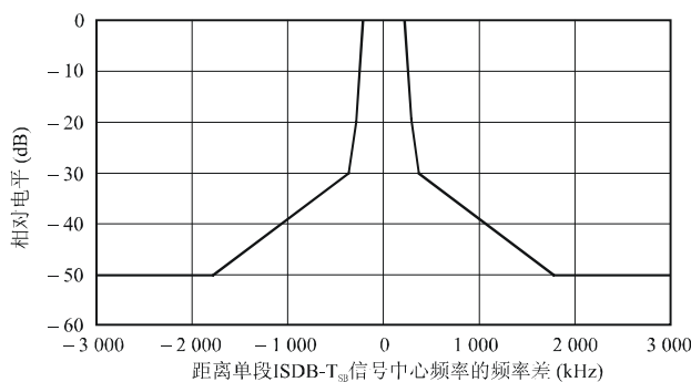
图 21 单段ISDB-TSB信号的频谱掩模 (段带宽=6/14 MHz)
