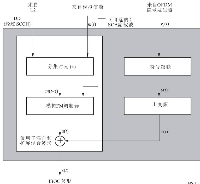
混合/扩展混合传输子系统功能框图
