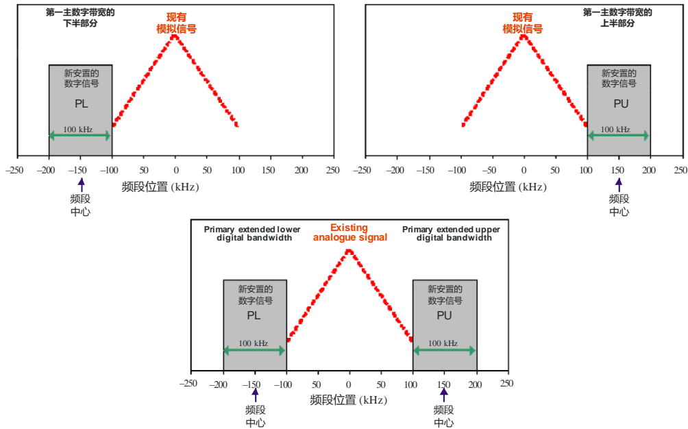
IBOC FM系统的扩展混合波形示例
