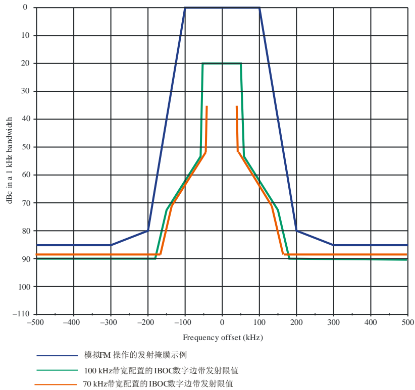
IBOC边带发射限值*
