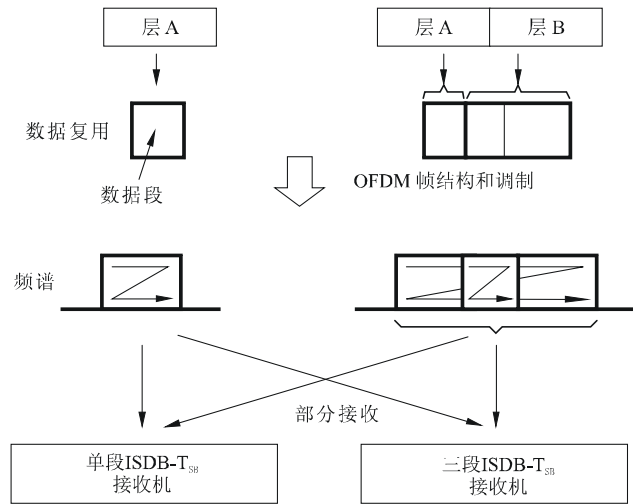
分层传输和部分接收举例图
