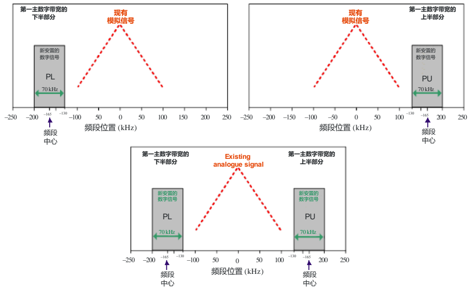
IBOC FM系统的主混合波形示例
