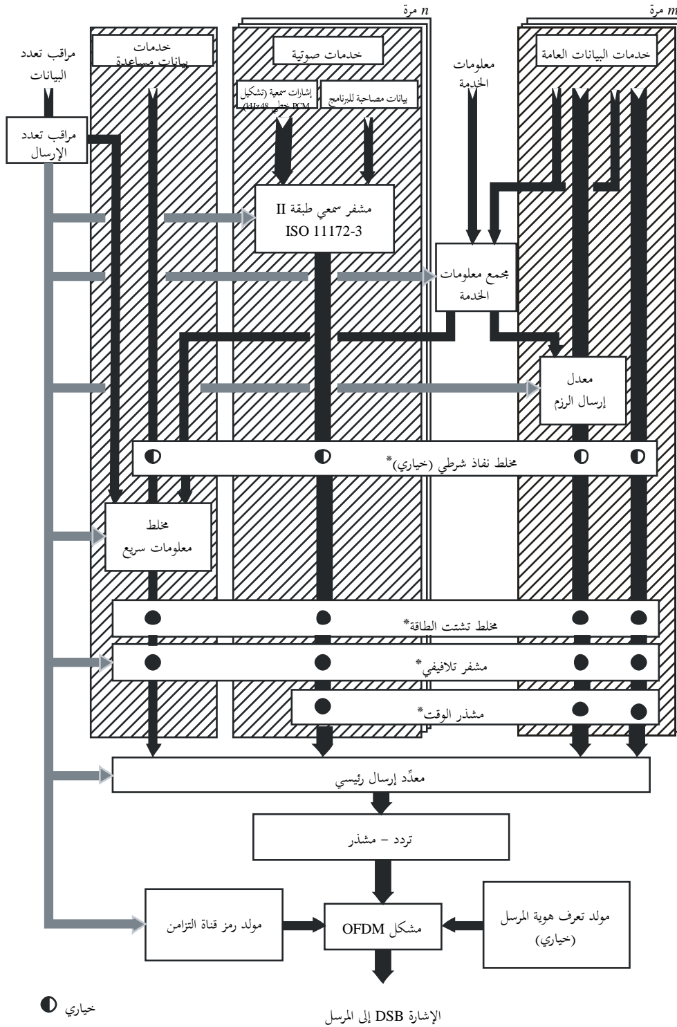
مخطط نظري لجزء الإرسال في النظام
