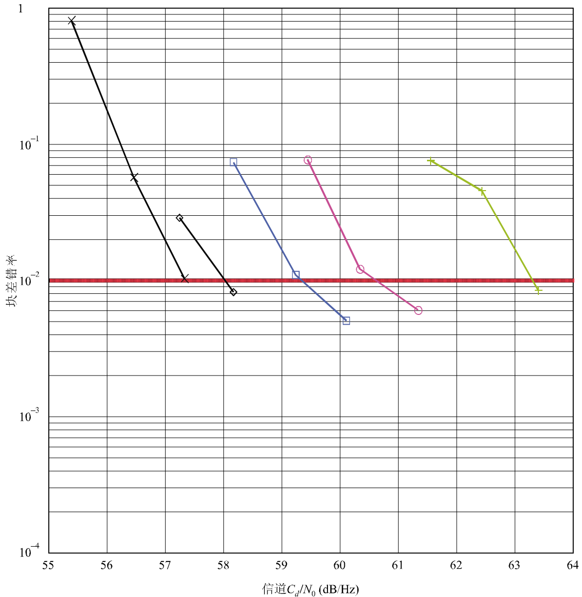
混合系统在9射线UF衰落和独立衰落的第一邻道 干扰情况下的块差错率结果
