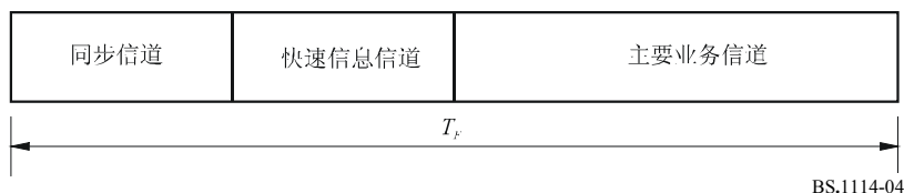
图4 多路复用帧结构
