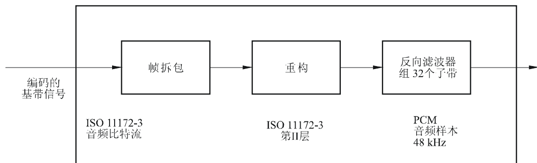
图3 基本的系统音频解码器框图
