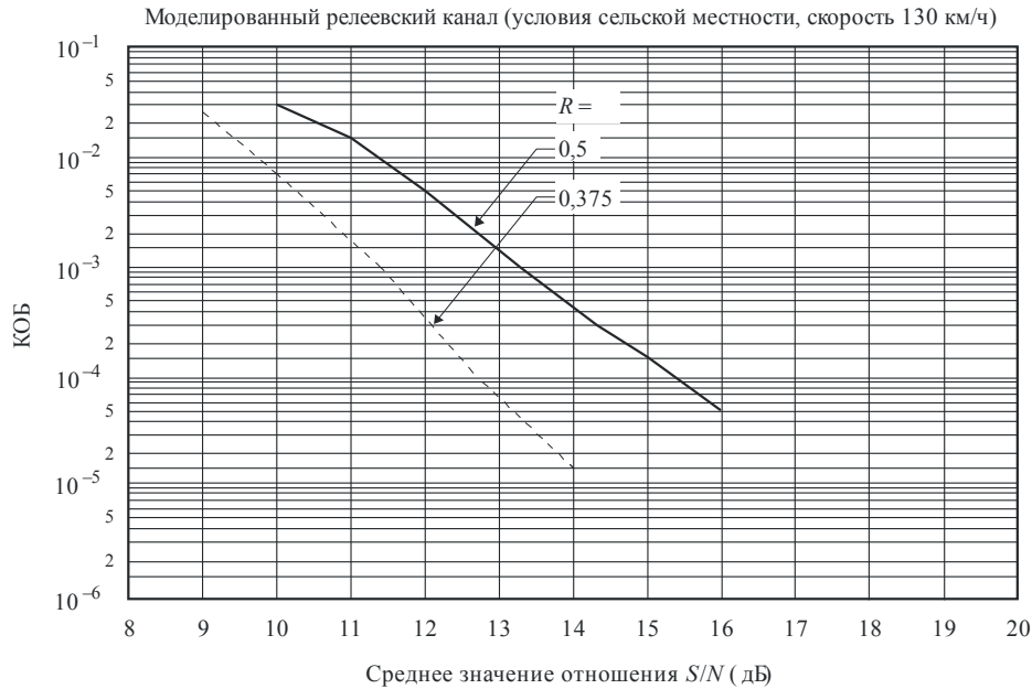
РИСУНОК 12 Зависимость КОБ от отношения S/N для Системы А (Передача в режиме I, 226 МГц)
