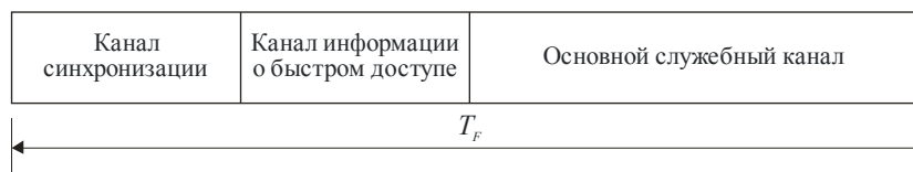
Структура цикла уплотненного сигнала
