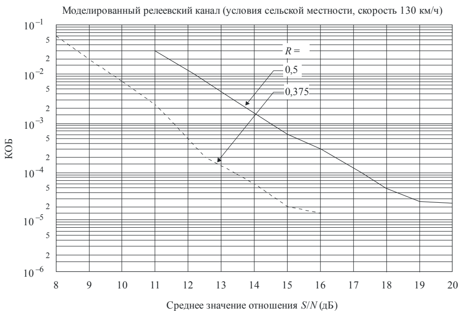
РИСУНОК 13 Зависимость КОБ от отношения S/N для Системы А (Передача в режиме II, 1480 МГц)
