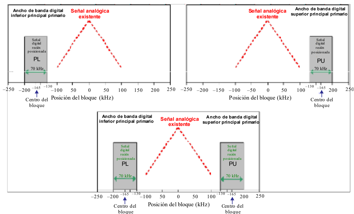
Ejemplos de forma de onda híbrida principal del sistema FM IBOC
