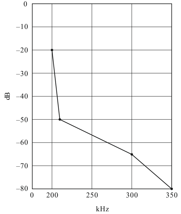
Curva espectral para el modo espectral C
