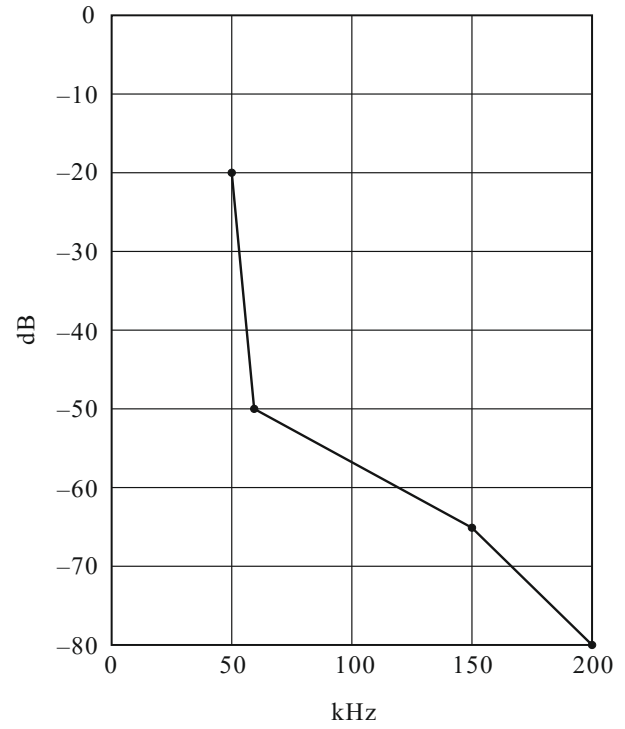
Curva espectral para el modo espectral A
