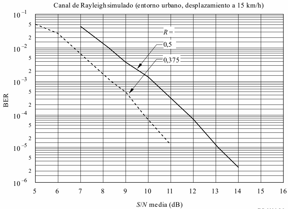
FIGURA 6 BER en función de la relación S/N para el Sistema A – (226 MHz)
