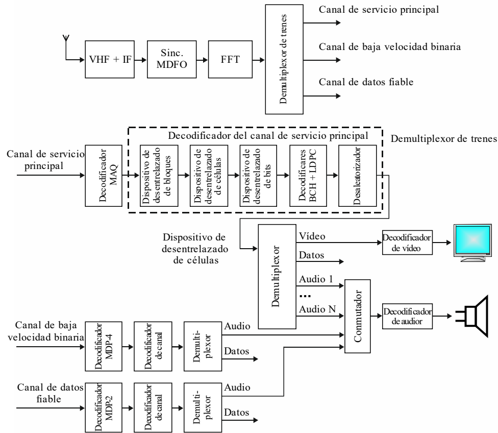
Diagrama de bloques funcionales de un receptor RAVIS
