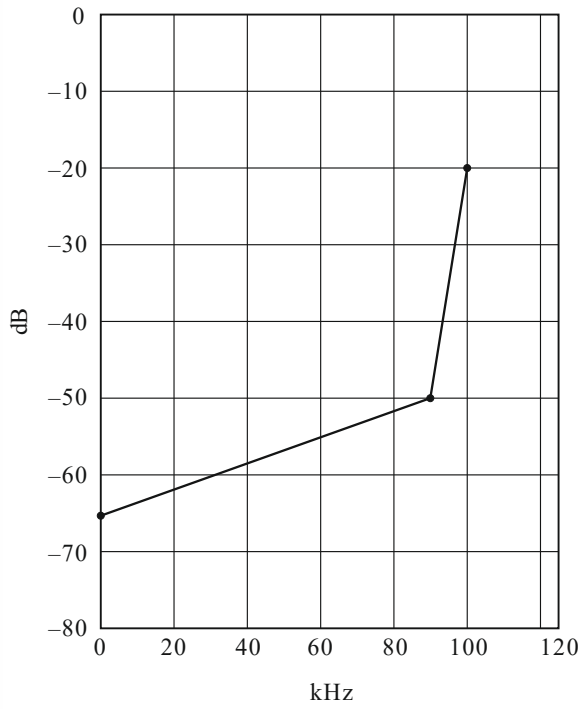
FIGURA 51 Curva espectral para el modo espectral E
