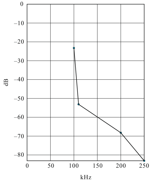
Curva espectral para el modo espectral B
