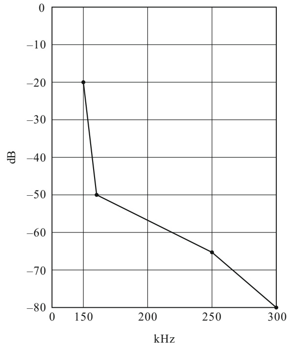
FIGURA 51 Curva espectral para el modo espectral E
