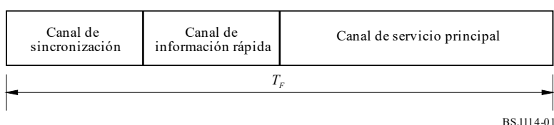
FIGURA 1 Estructura de la trama múltiplex
