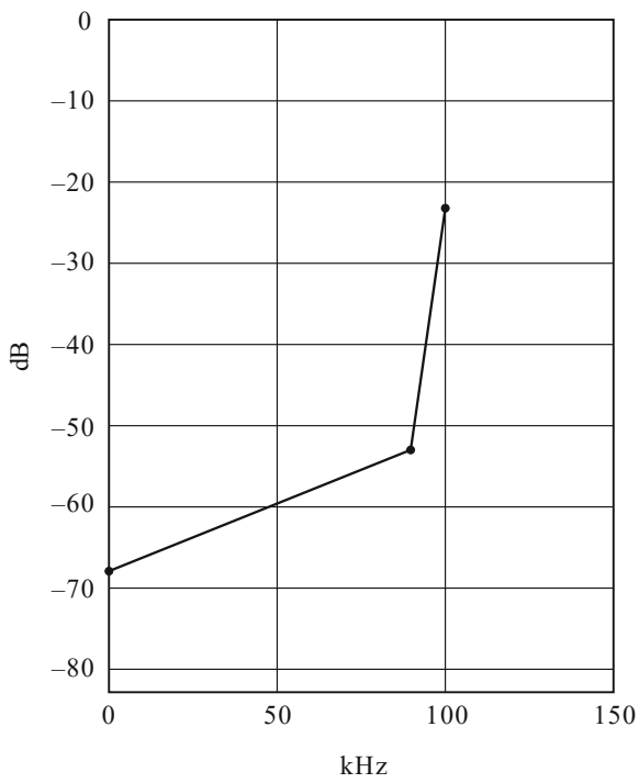
FIGURA 52 Curva espectral para el modo espectral F
