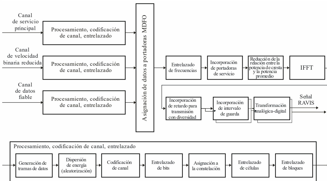
Diagrama de bloques funcionales de un transmisor RAVIS
