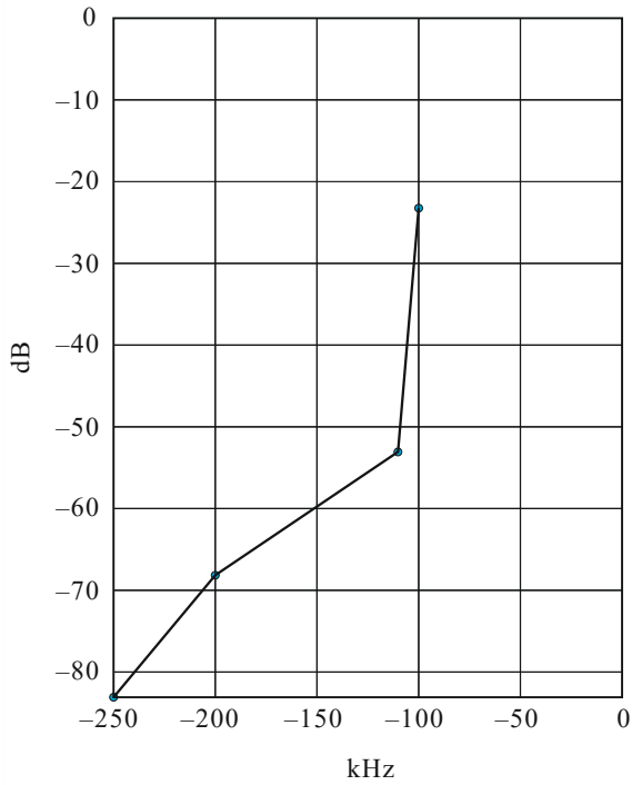
Curva espectral para el modo espectral B
