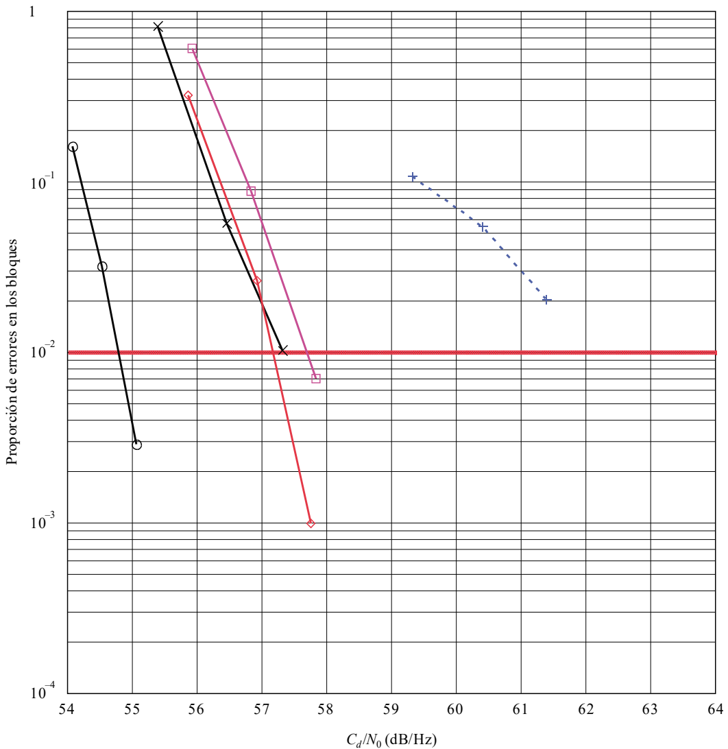
Resultados de la proporción de errores en los bloques del sistema híbrido ante diferentes tipos de desvanecimiento de nueve trayectorias y ruido gaussiano blanco aditivo (AWGN)
