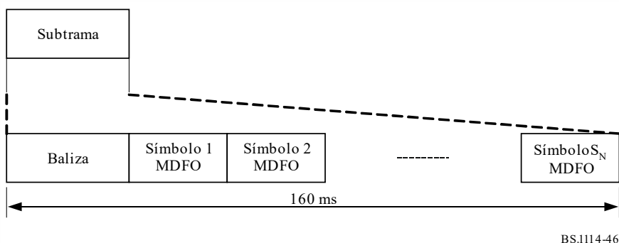
FIGURA 46 Estructura de una subtrama
