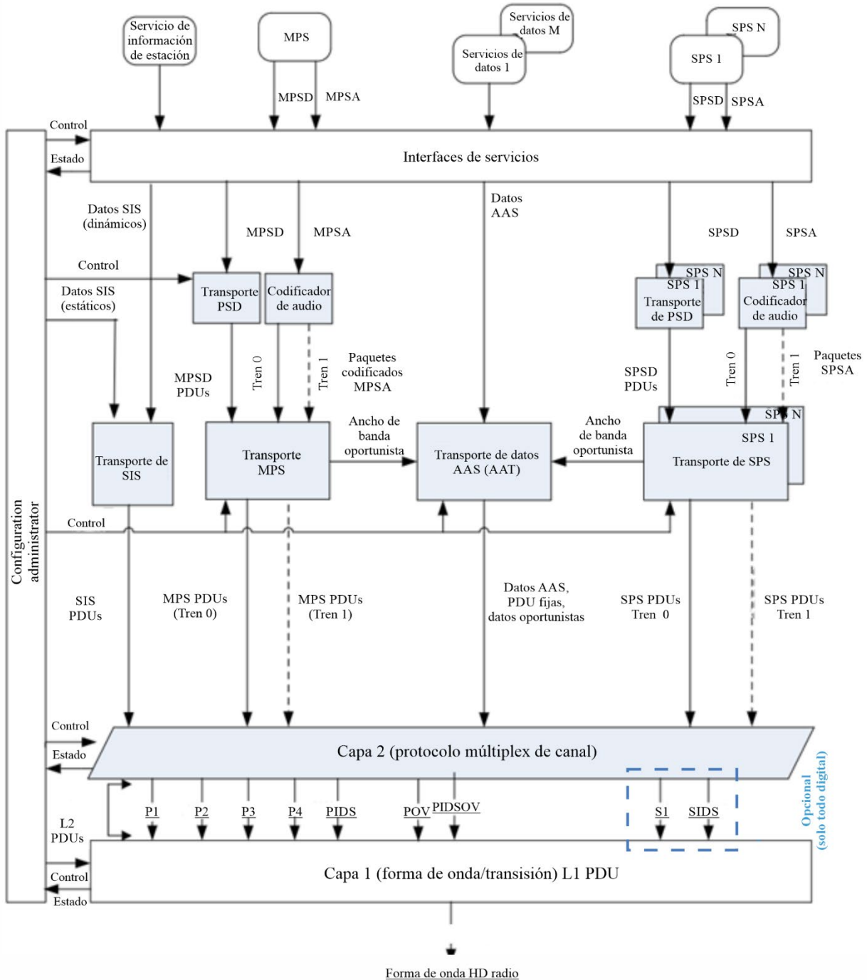
Diagrama de bloques de la pila de protocolo del sistema IBOC FM
