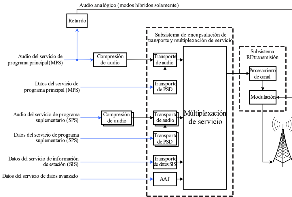
FIGURA 21 Esquema del sistema de radiodifusión IBOC
