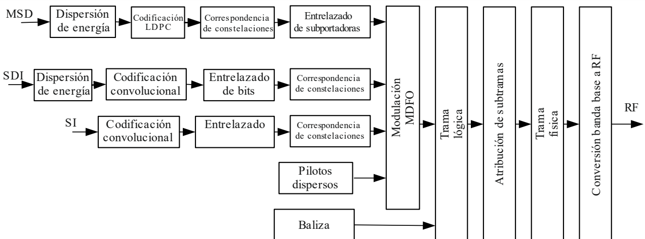
FIGURA 45 Diagrama de codificación y modulación del canal
