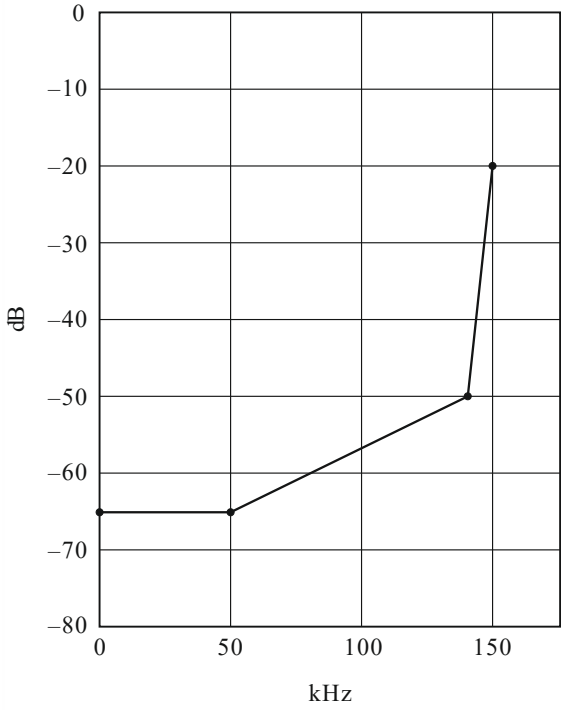
Curva espectral para el modo espectral C
