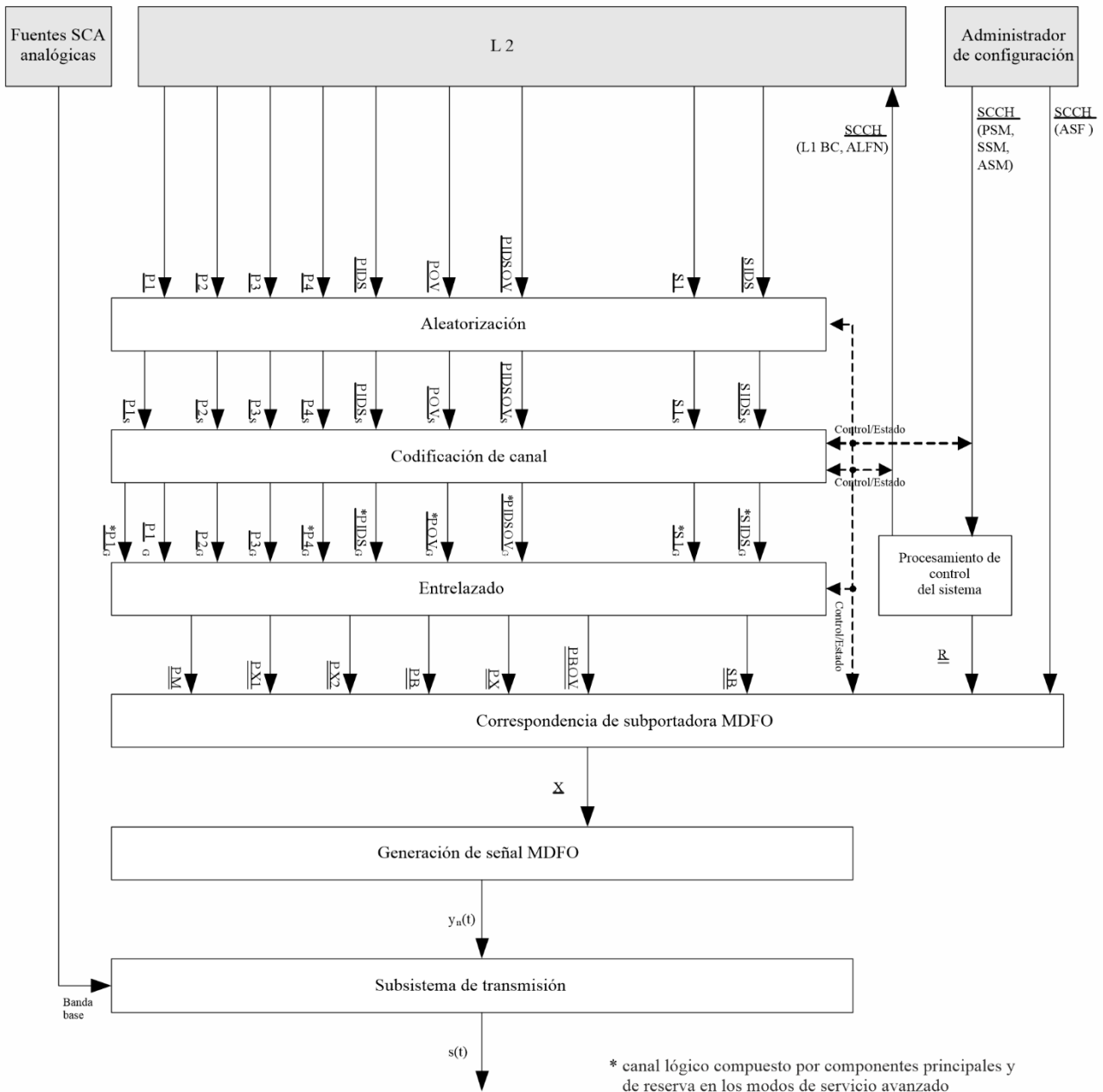
FIGURA 25 Diagrama de bloques funcional de L1 de la interfaz aérea de MF
