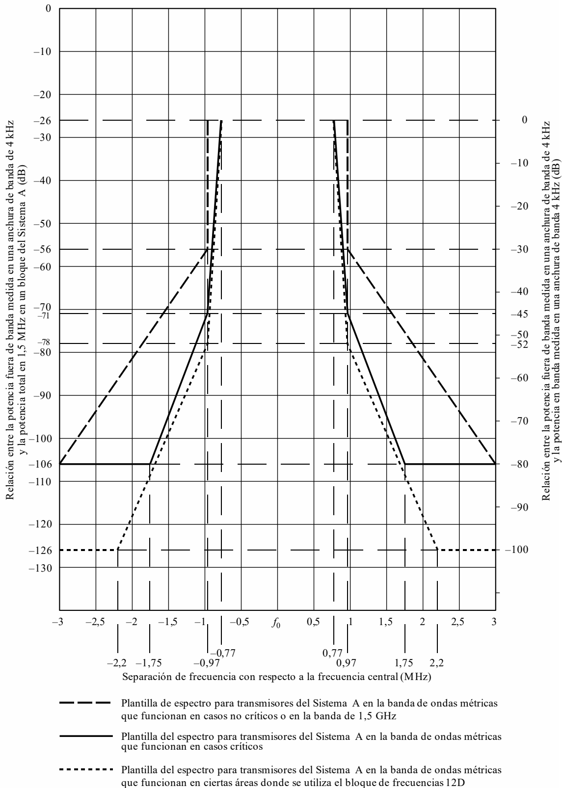
FIGURA 4 Plantillas del espectro fuera de banda para el Sistema A
