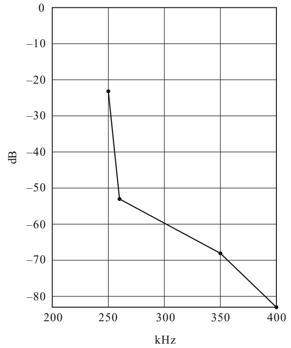
Curva espectral para el modo espectral D
