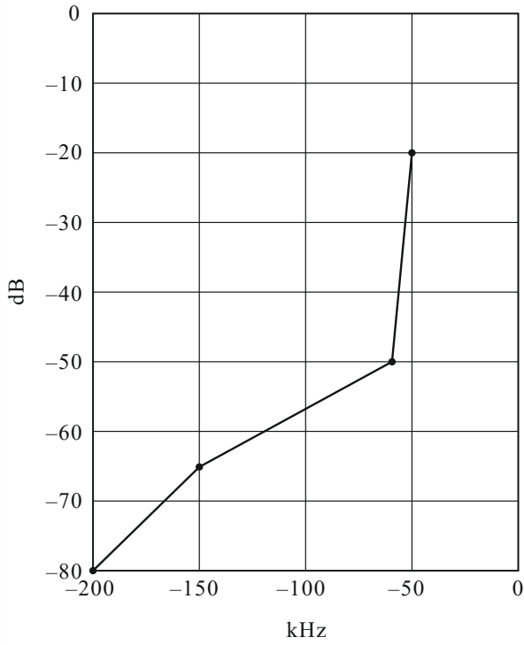
Curva espectral para el modo espectral A
