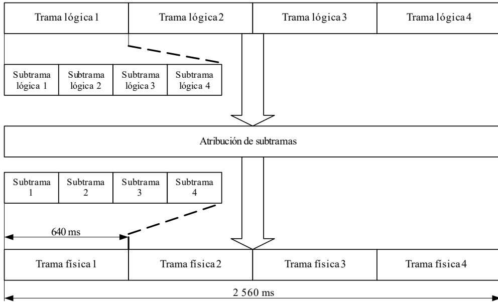
FIGURA 44 Trama lógica y atribución de subtrama
