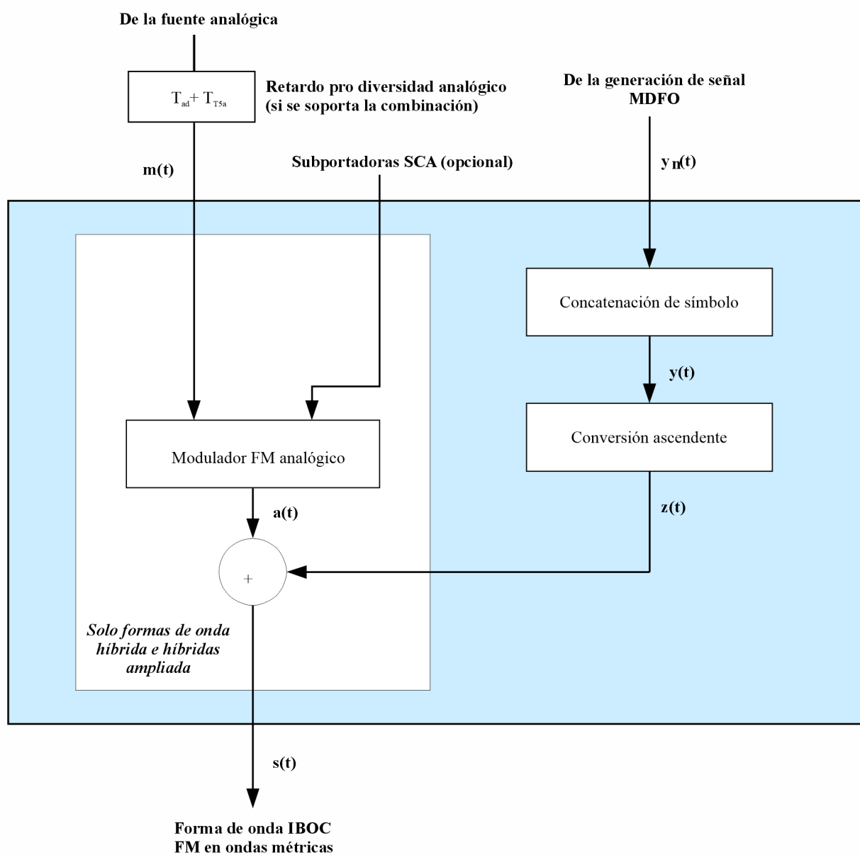
Diagrama de bloques funcional del subsistema de transmisión híbrido/híbrido ampliado
