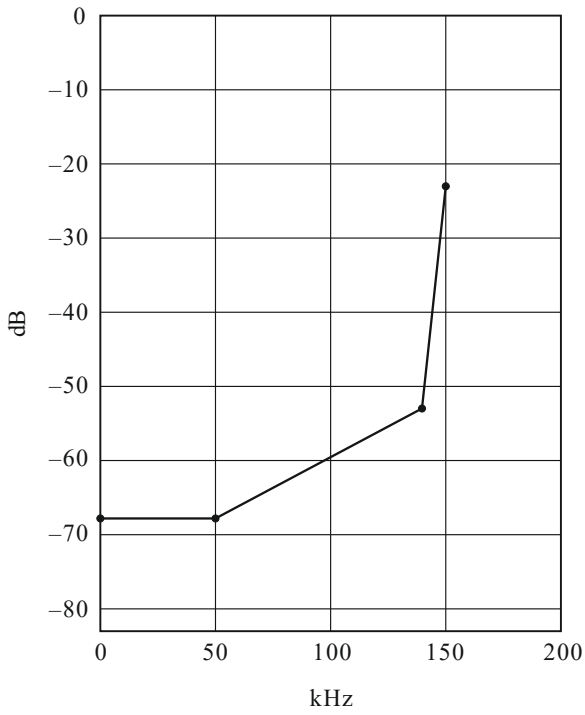
Curva espectral para el modo espectral D
