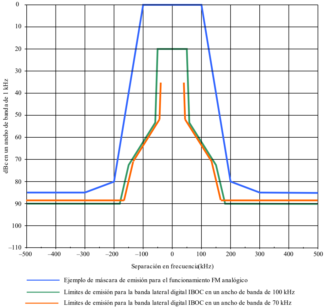
FIGURA 33 Límites de las emisiones en banda lateral IBOC*
