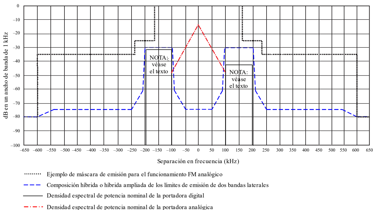
Límites de la emisión en modo híbrido IBOC*
