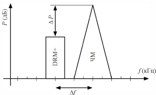
РИСУНОК 40 Пример конфигурации цифровой системы G (DRM, режим E, левая часть) и ЧМ-сигнала (правая часть)
