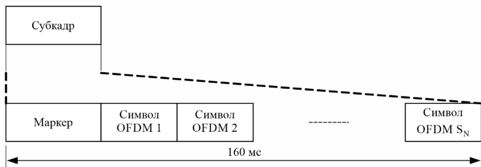
РИСУНОК 46 Структура субкадра
