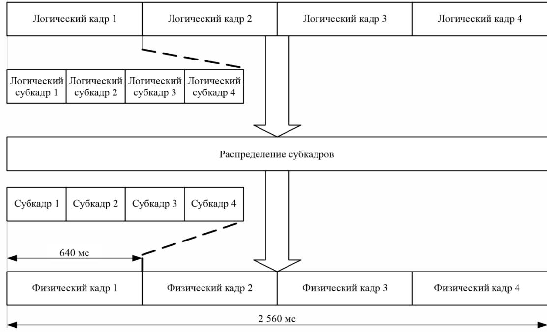
РИСУНОК 44 Логический кадр и распределение субкадров
