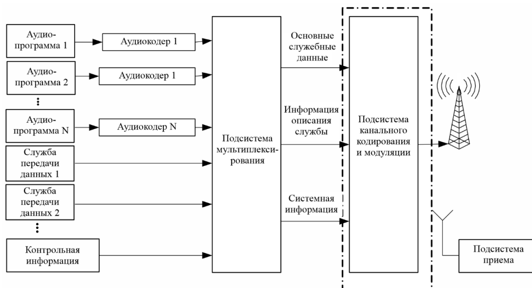
РИСУНОК 42 Обзор системы
