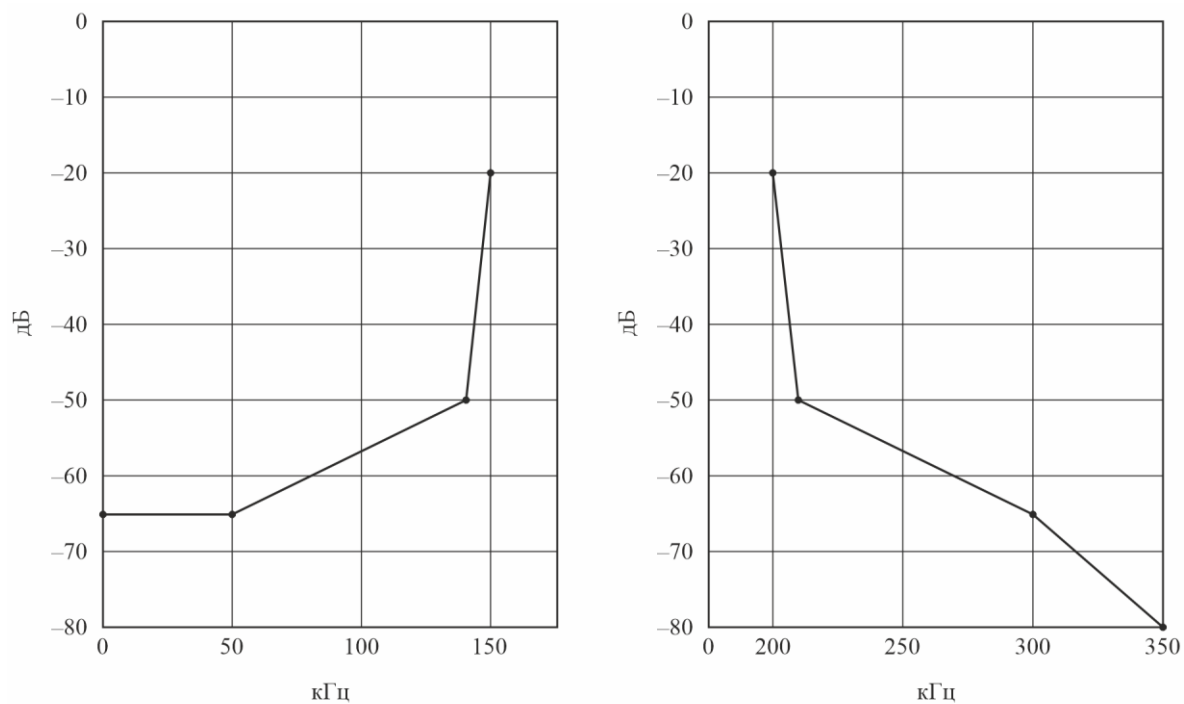
РИСУНОК 49 Спектральная маска режима спектра С
