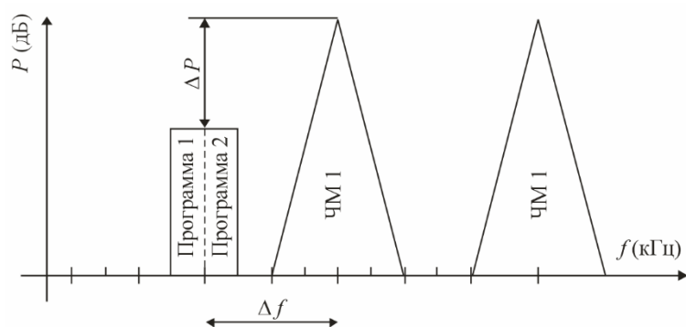
РИСУНОК 41 Пример конфигурации цифровой системы G (слева) и двух ЧМ-станций (справа)
