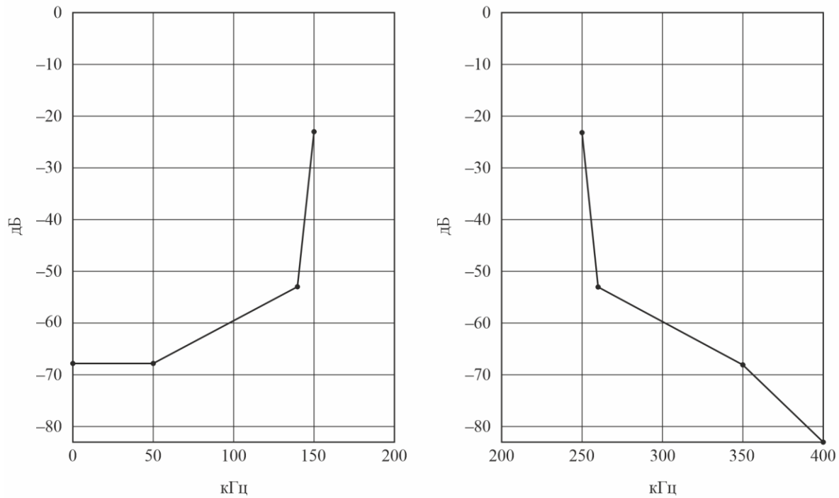
РИСУНОК 50 Спектральная маска режима спектра D
