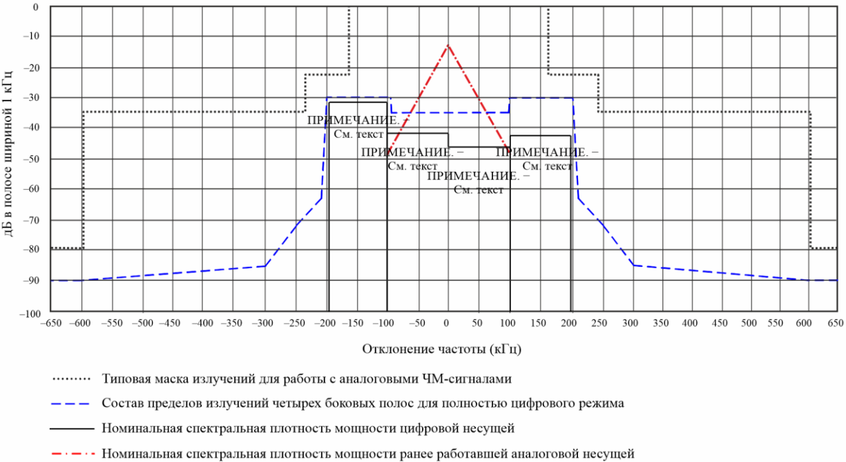
РИСУНОК 32 Пределы излучений в полностью цифровом режиме
