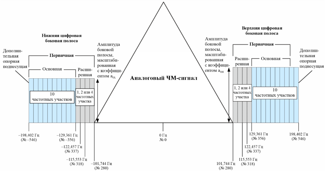
РИСУНОК 29 Спектр расширенной гибридной волны – режимы обслуживания MP2, MP3, MP11, MP12, MP5, MP6, MP1X, DSB1, MP1XOV, MP6OV и DSB1OV
