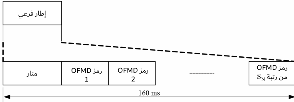
هيكل إطار فرعي واحد
