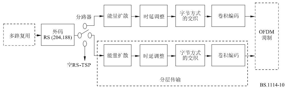
图10 信道编码图
