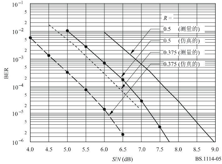
图5 系统A的BER对比S/N 高斯信道
