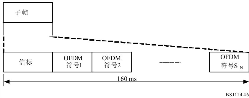
图46 子帧结构
