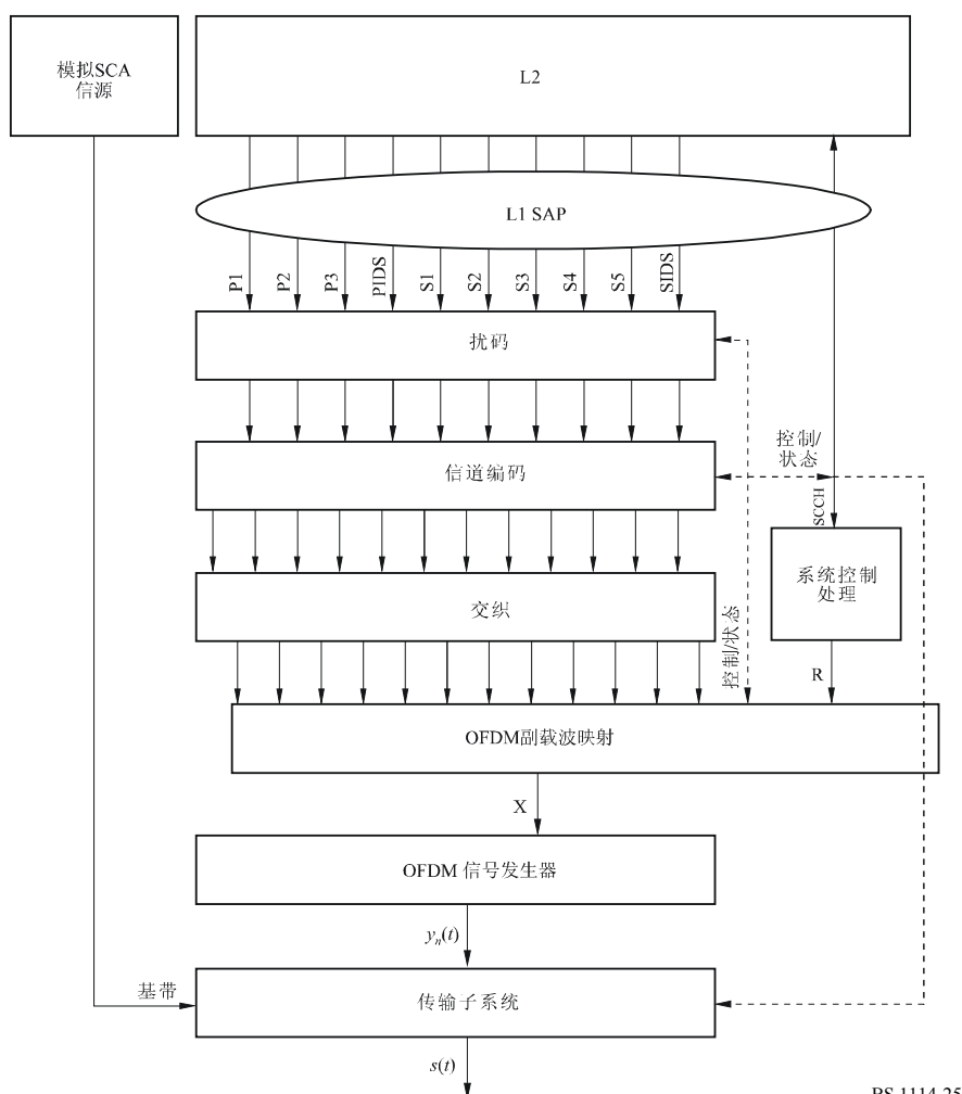
图25 FM空中接口L1功能框图
