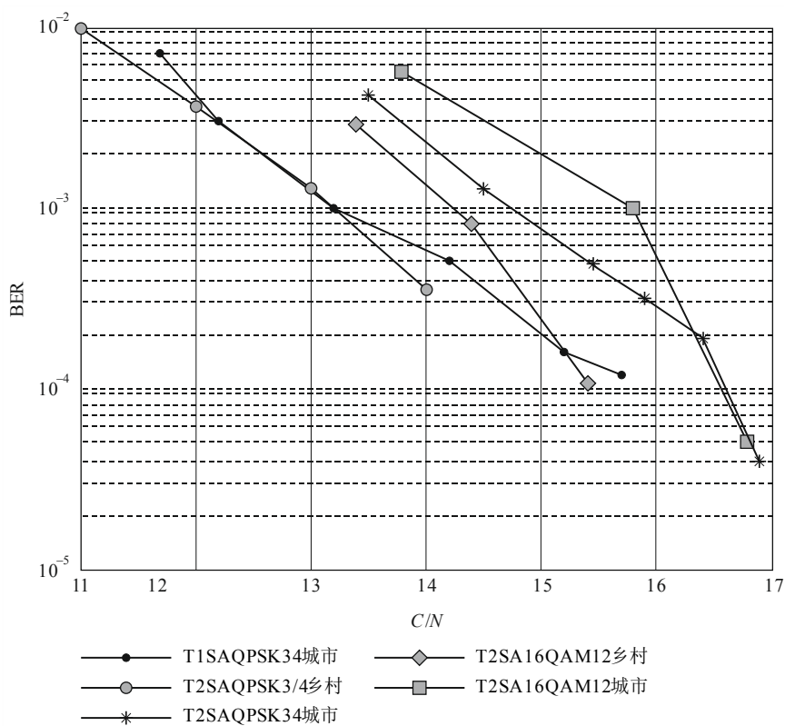
多径信道中的BER对比C/N
