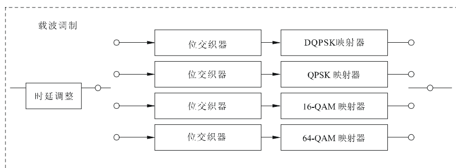
图13 载波调制单元的配置
