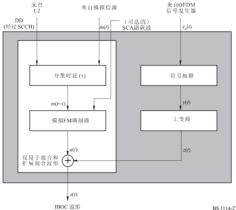
混合/扩展混合传输子系统功能框图
