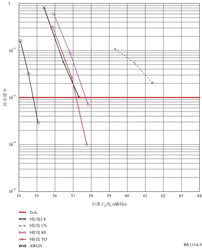
图34 混合系统在不同类型的9射线衰落和加性高斯白噪声（AWGN） 情况下的块错误率结果
