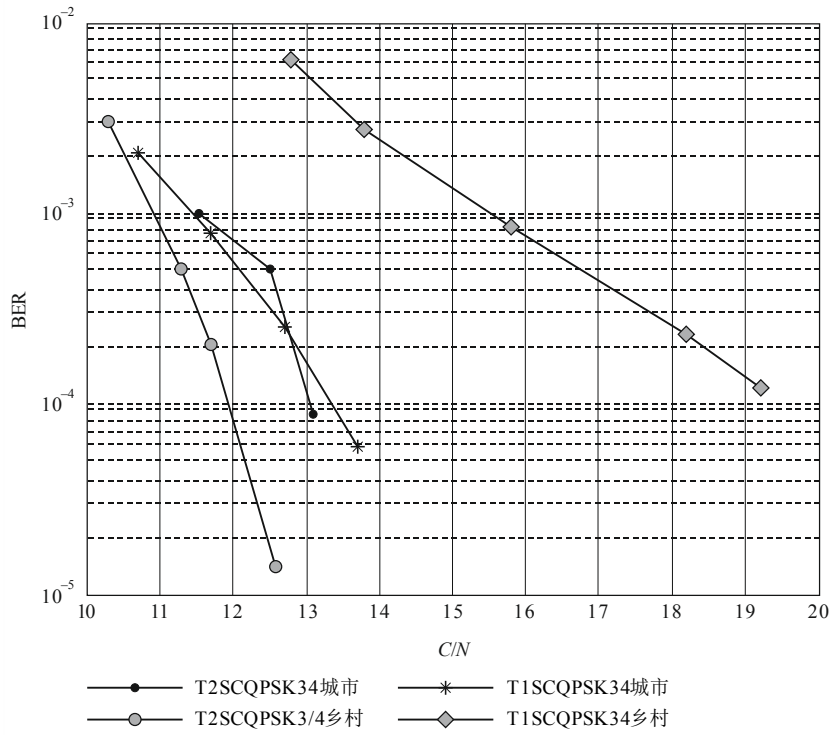
多径信道中的BER对比C/N
