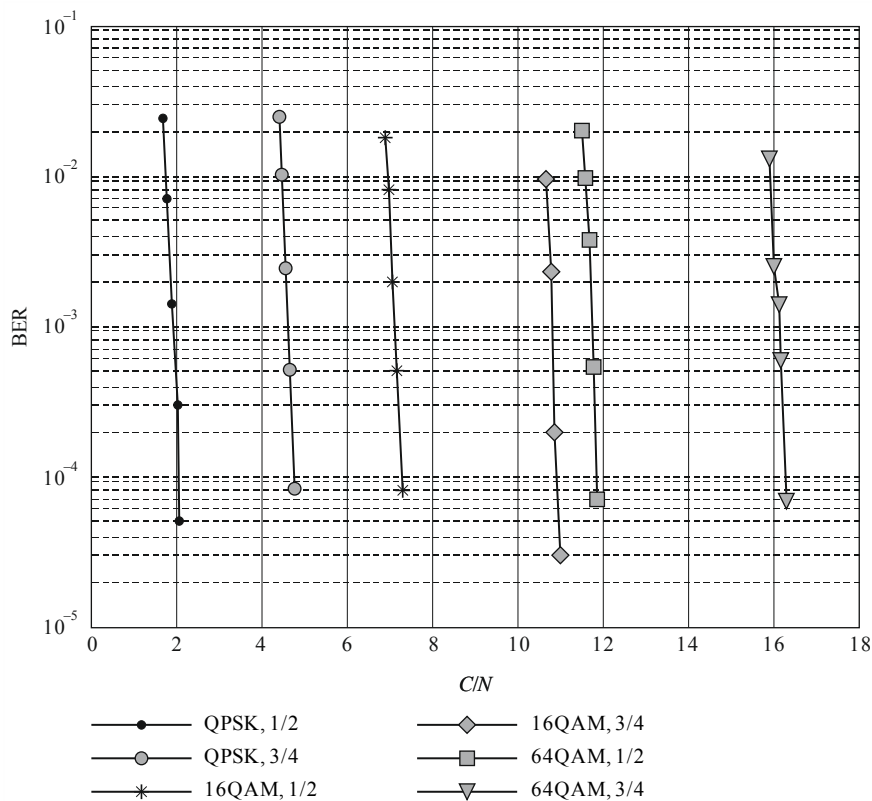
高斯信道中的BER对比 C/N
