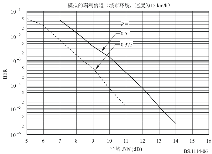
图6 系统A的BER对比S/N （传输模式I，266 MHz）
