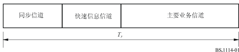
图1 多路复用帧结构
