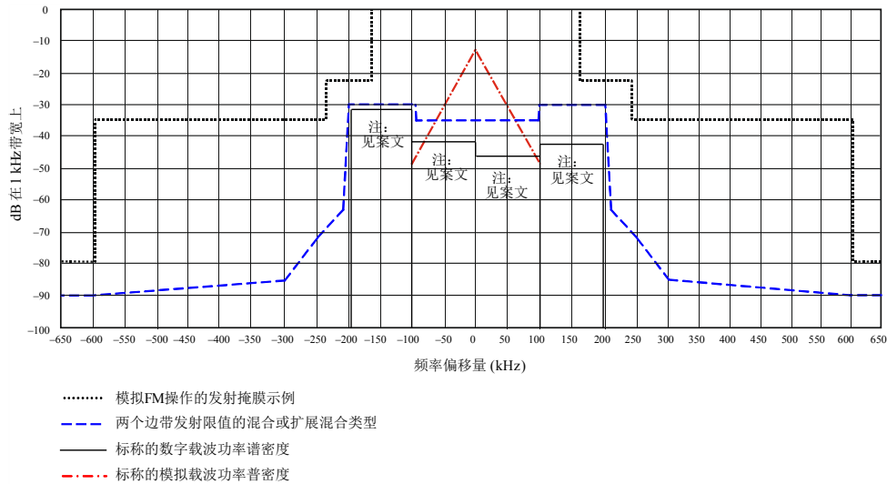
图32 全数字发射限制*
