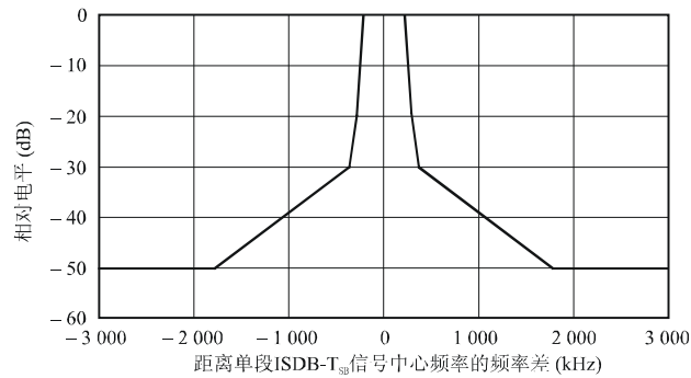
图14 单段ISDB-T SB 信号的频谱掩模 (段带宽=6/14 MHz)
