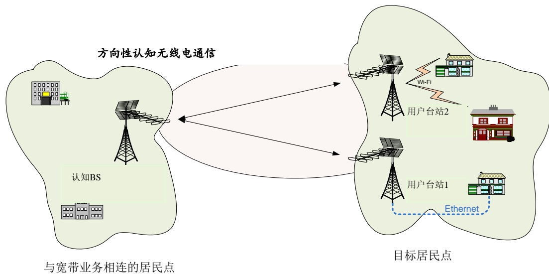
470-686 MHz频段使用方向性天线的居民点间P-MP链路
