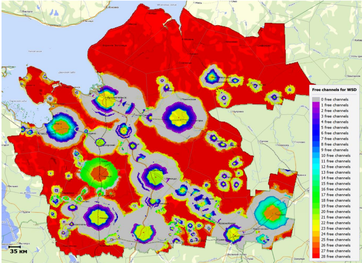
图 A5-2 Arkhangelsk区内功率为20 dBm (100 mW) 的WSD频谱可用性图示例
