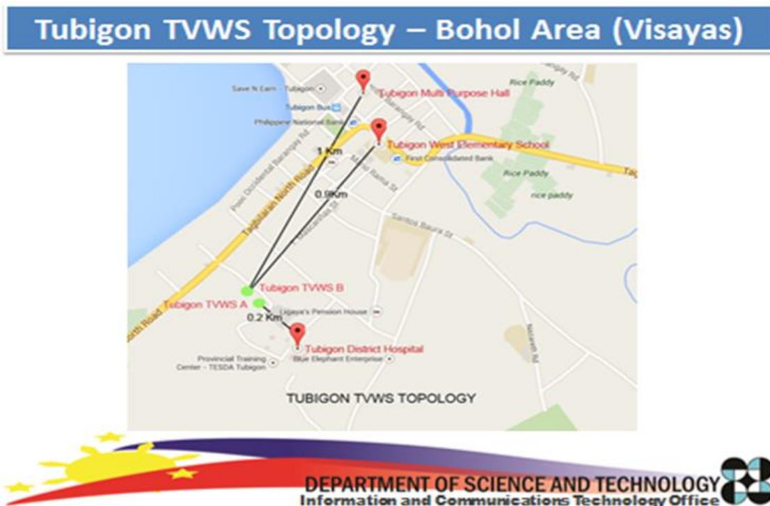
Tubigon市TVWS项目覆盖图
