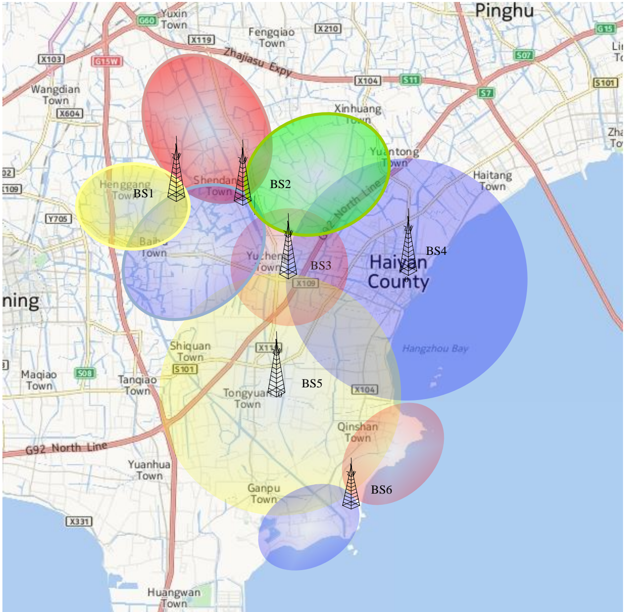
图 A6-2 海盐的试点网络部署
