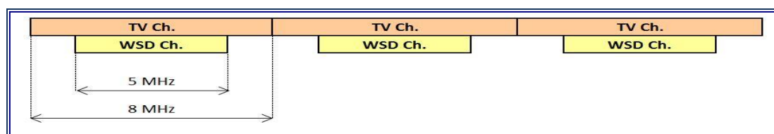
电视和WSD频道格栅
