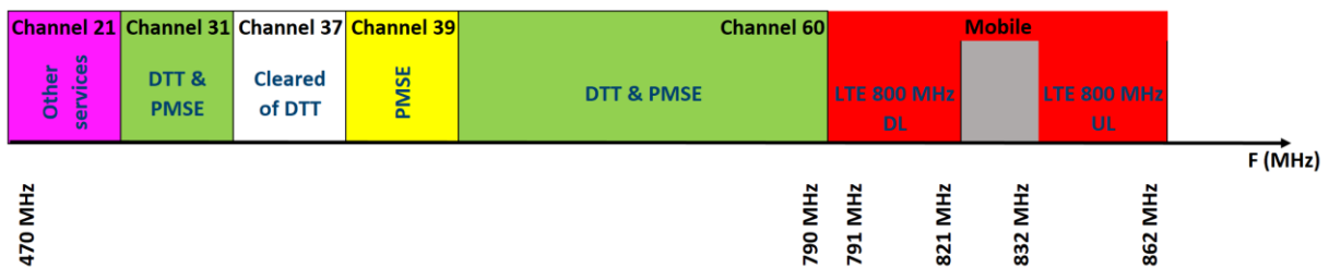
对UHF电视频段（470-790 MHz）及其欧洲用户的说明
