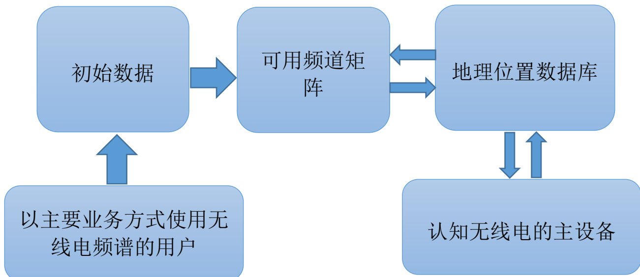
使用地理位置数据库的认知系统的原理
