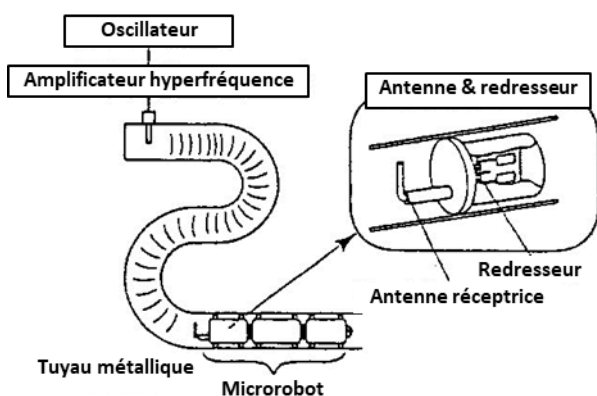
a) Concept de robot alimenté en MPT pour se déplacer dans un tuyau
