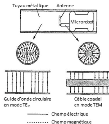
b) Méthode classique de conversion d'énergie provenant d'un guide d'onde circulaire et dirigée vers un câble coaxial [SHB 97]
