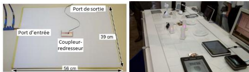
FIGURE 7 Système 2DWPT
