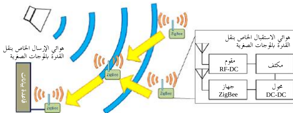
صورة لأجهزة الاستشعار ZibBee المزودة بالطاقة لاسلكياً [ICH12]
