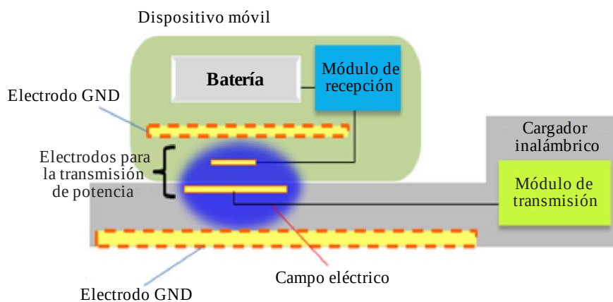
Estructura típica del sistema de acoplamiento capacitivo
