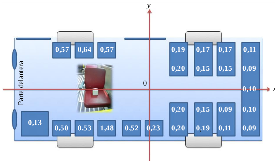
FIGURA A1-4 Distribución del campo magnético calculado según la distancia al OLEV
