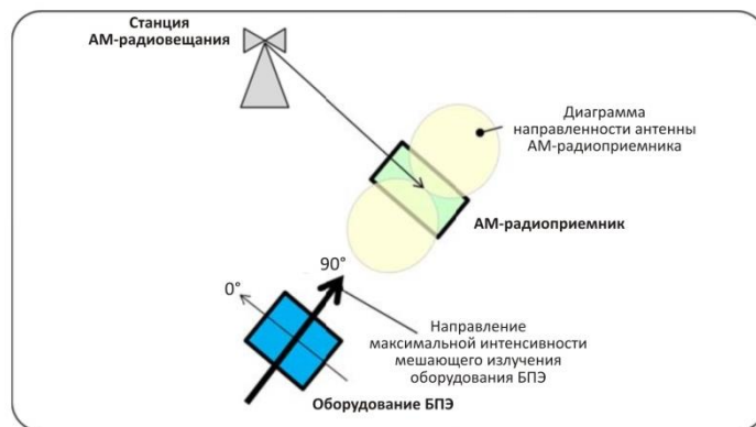
РИСУНОК 15 Условия измерений в ходе испытания на слышимость
