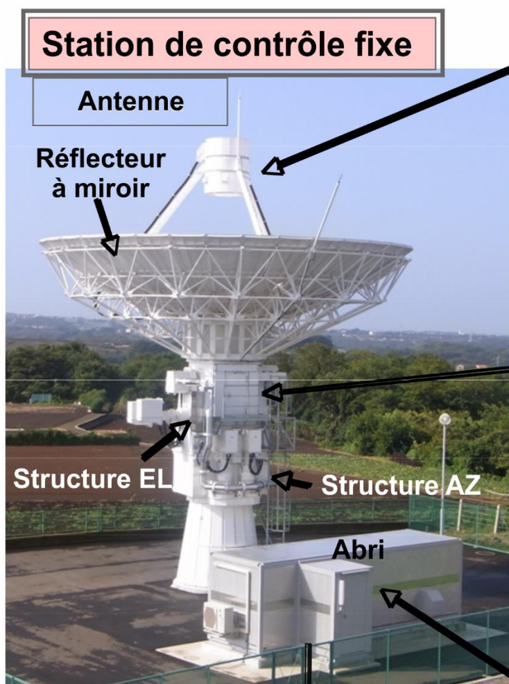
FIGURE 13 Configuration de l'antenne de 13 m
