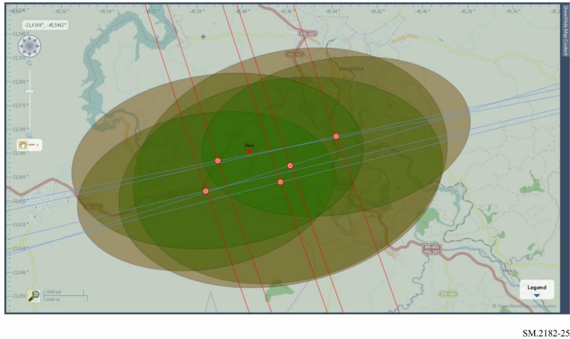
FIGURE 27 Résultats de la géolocalisation (ellipses de géolocalisation répétées cinq fois et convergeant vers la même région)
