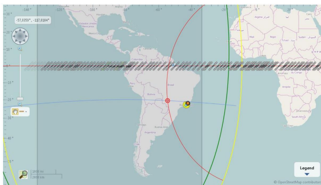
FIGURE 25 Résultats de la géolocalisation (lignes TDOA et FDOA et indication de la cible)
