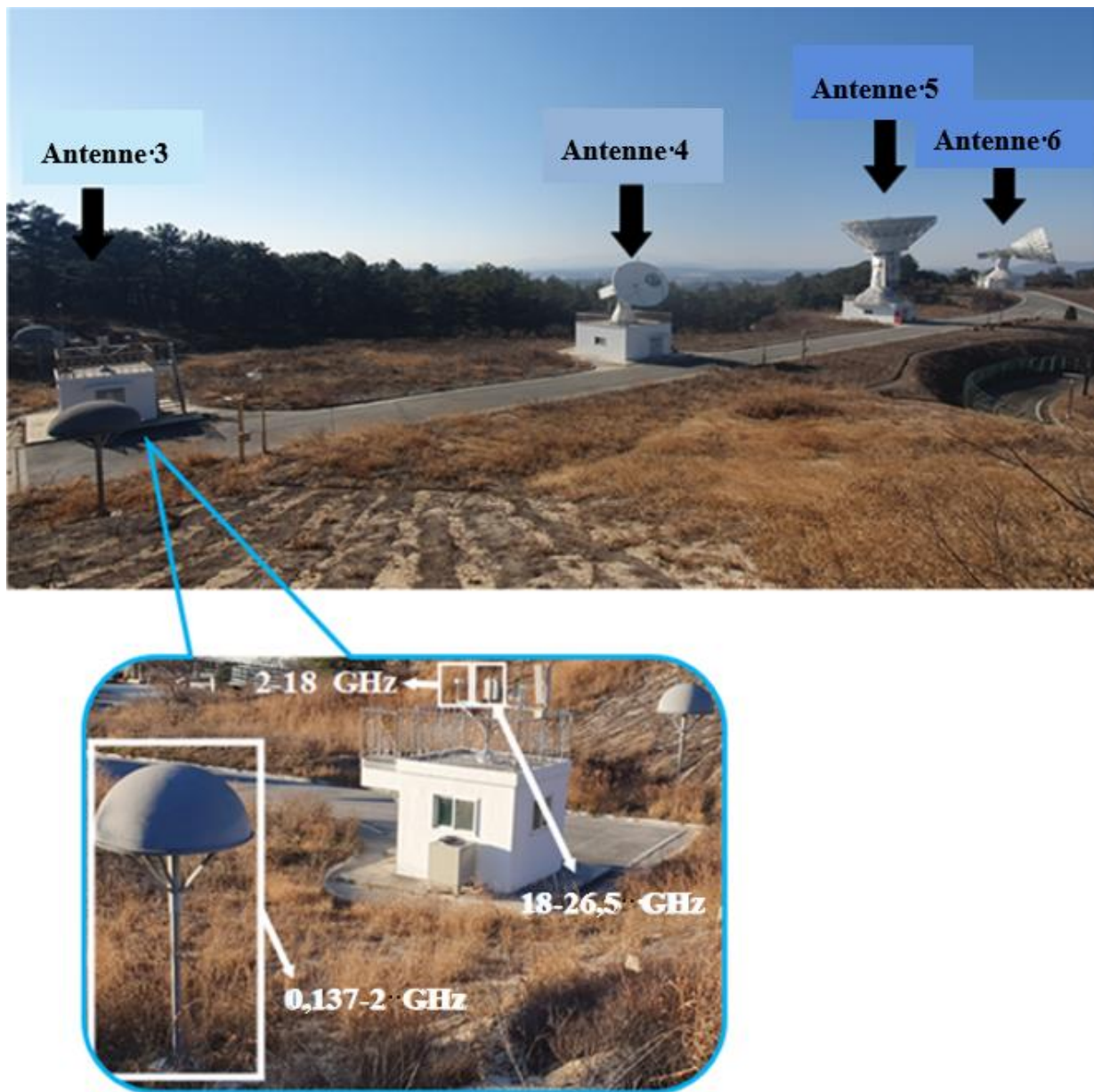
FIGURE 8 Antennes 3, 4, 5 et 6 du SRMC
