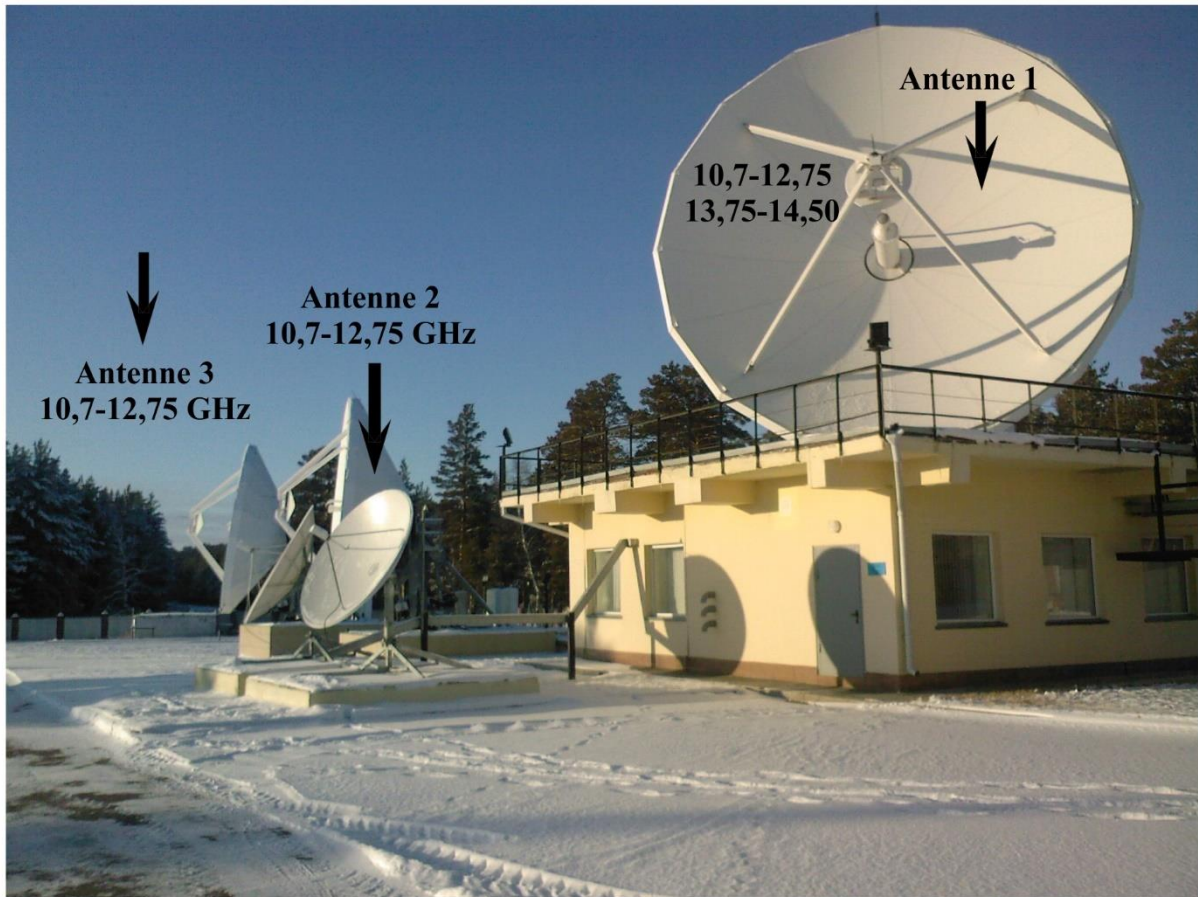
FIGURE 23 Vue d'ensemble des systèmes N° 1, 2 et 3
