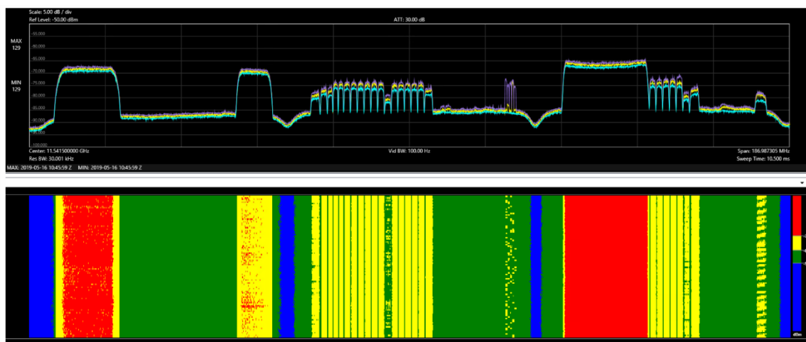
FIGURE 30 Spectrogramme des répéteurs reçus
