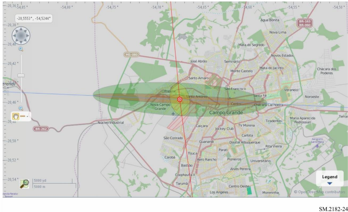
FIGURE 26 Résultats de la géolocalisation (ellipse de géolocalisation)
