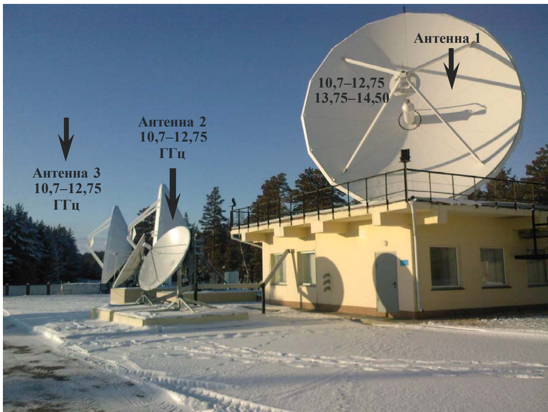
Общий вид антенных систем 1, 2 и 3
