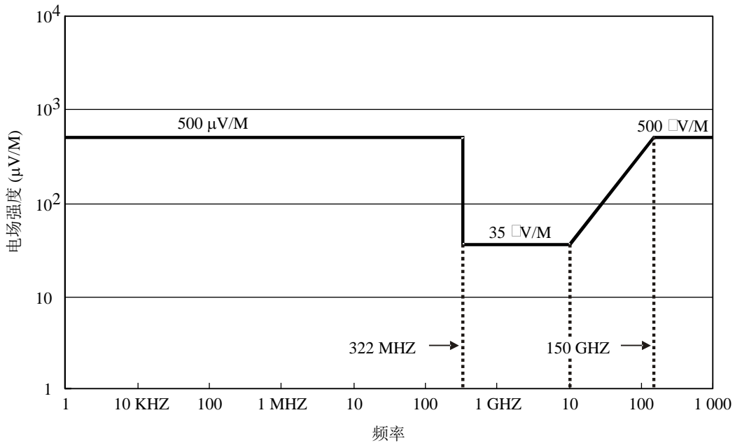
距发射极小功率无线电站3 m处电场强度的最大容限值*
