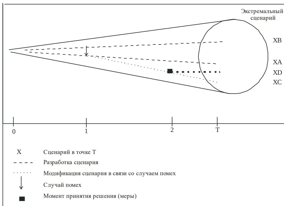
РИСУНОК 4 Разработка сценариев
