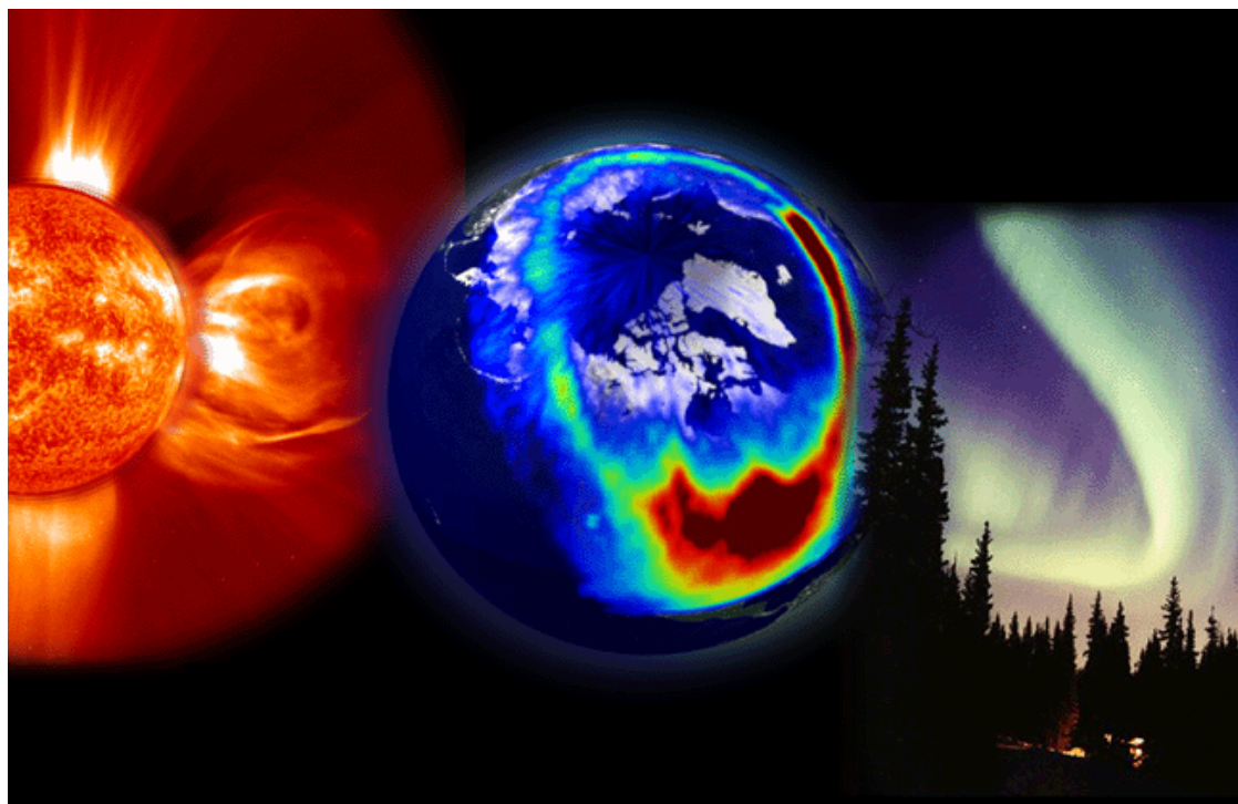
Figure 5: L'activité solaire vue depuis un satellite et depuis la Terre
