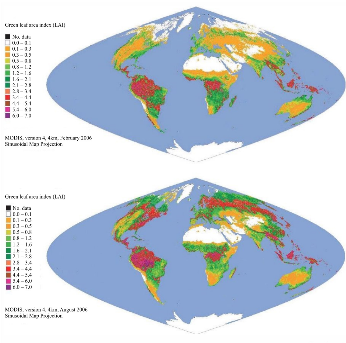
Figure 2: Indices de feuilles vertes fournis par MODIS montrant les variations saisonnières de la végétation
