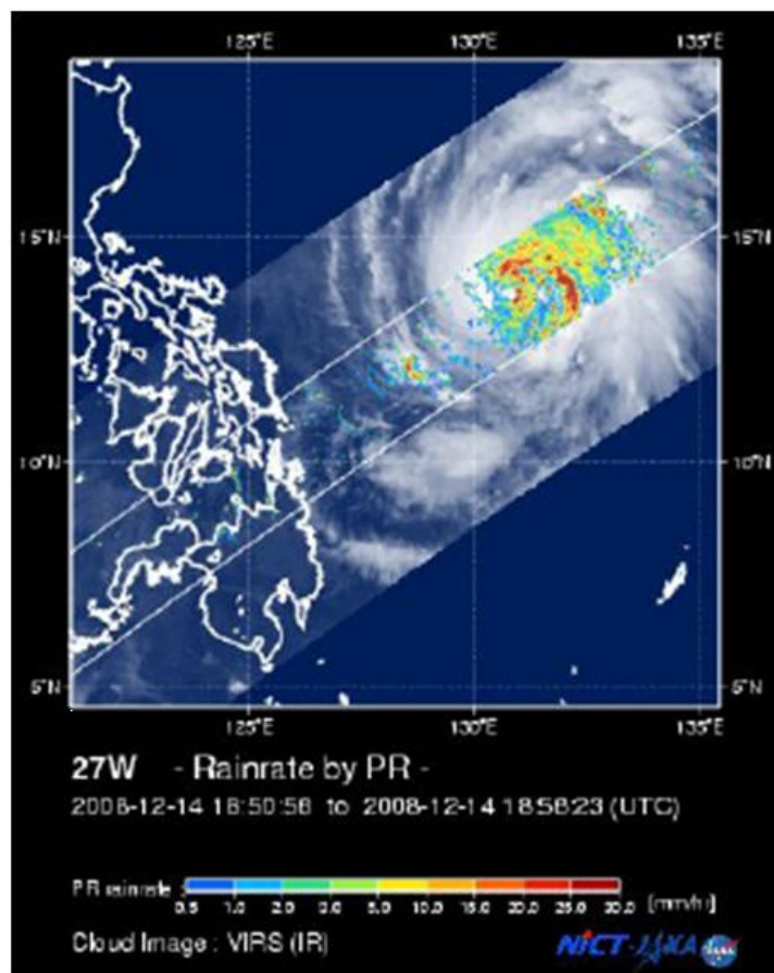
Figure 3: Répartition des taux de précipitation d'un typhon
