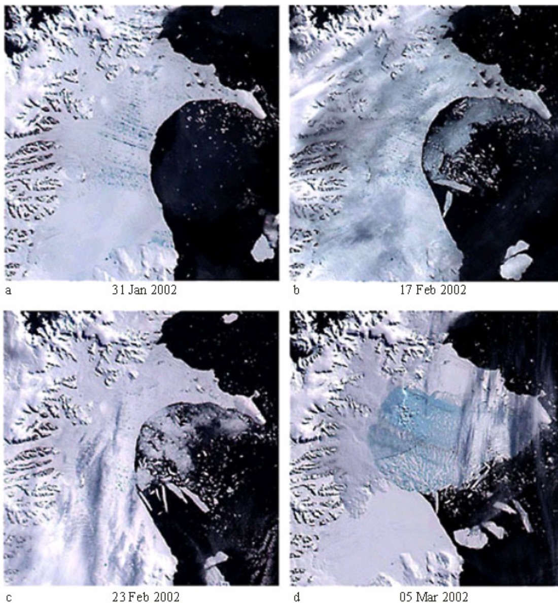
Figure 1: Effondrement de la plate-forme de glace Larsen B dans l'Antarctique ouest: 2 000 km 2 de glace continentale désintégrés en l'espace de deux mois
