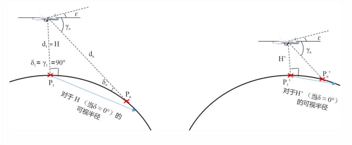
对两种不同A-ESIM高度的合规性审查的几何图形
