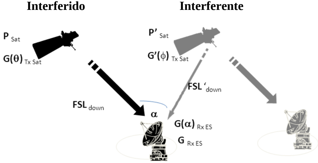
Fig. 3. Hipótesis de interferencia en el enlace descendente
