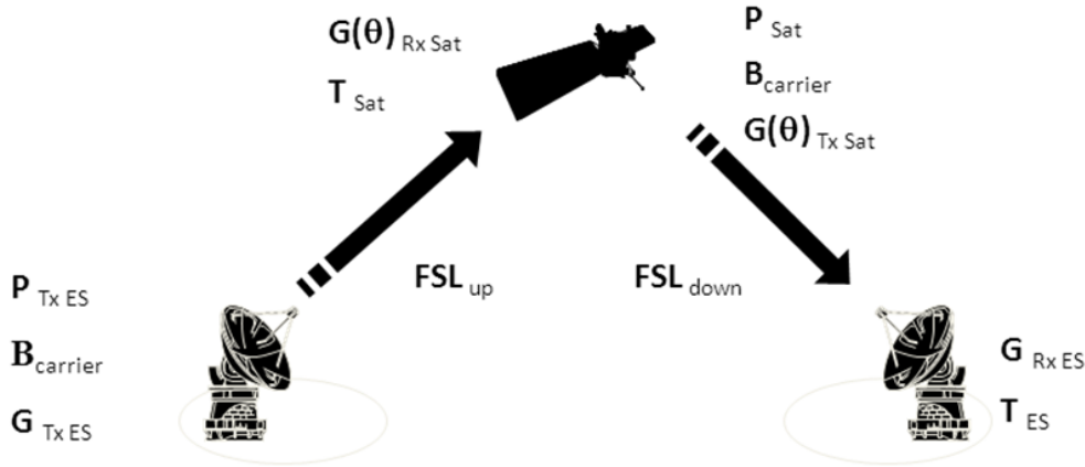
Fig. 1. Enlace de comunicaciones por satélite
