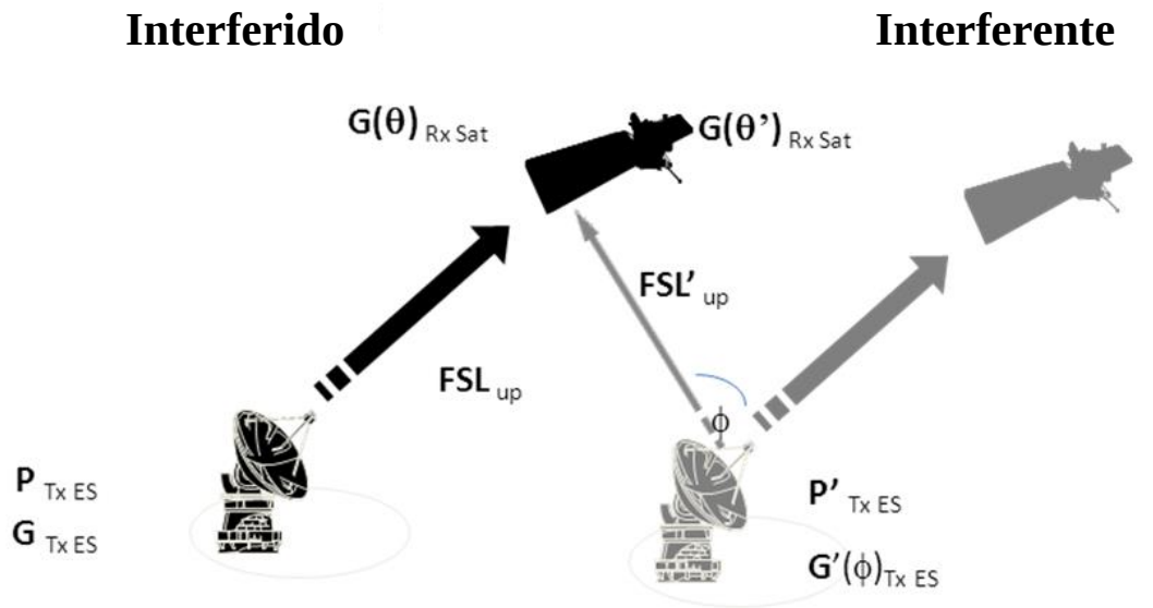
Fig. 2. Hipótesis de interferencia en el enlace ascendente
