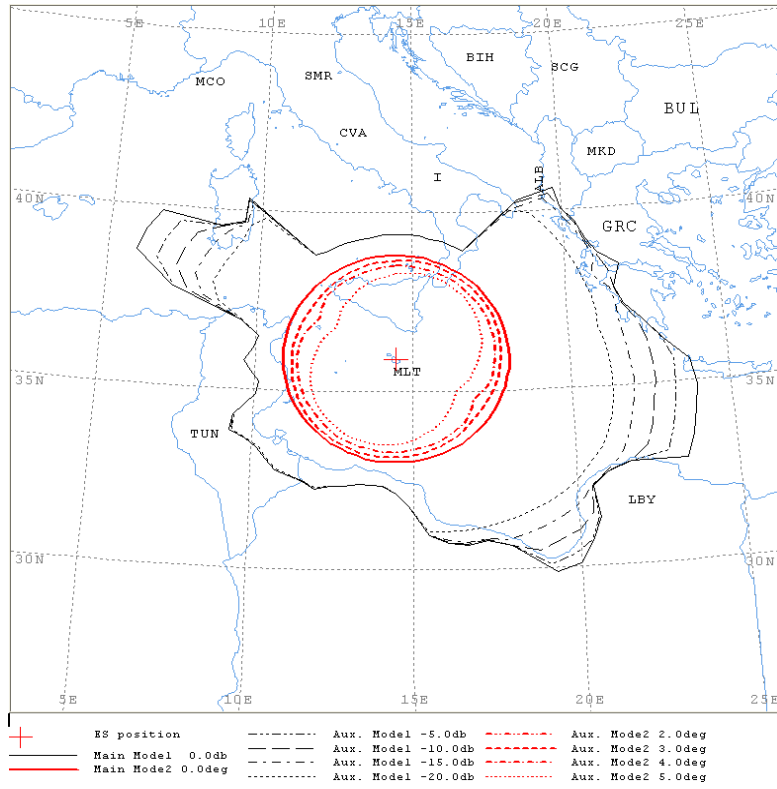
图3 针对发射地面台站的卫星固定业务接收GSO地球站
