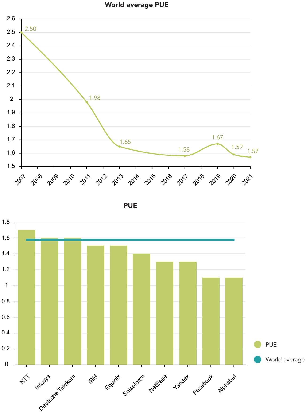
Figure 3.2: PUEs
