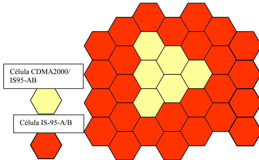
Figura F.4 – Superposición selectiva de células CDMA2000 e integración sin interfaces en una red IS-95 A/B
