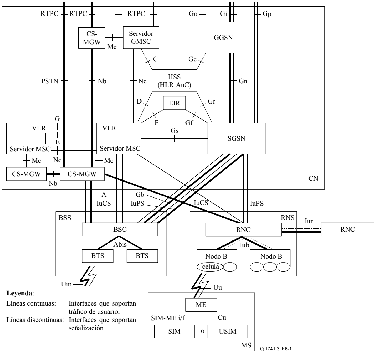
Figura 6-1/Q.1741.3 – Configuración básica de una RMTD que soporta servicios e interfaces con conmutación de circuitos y conmutación de paquetes
