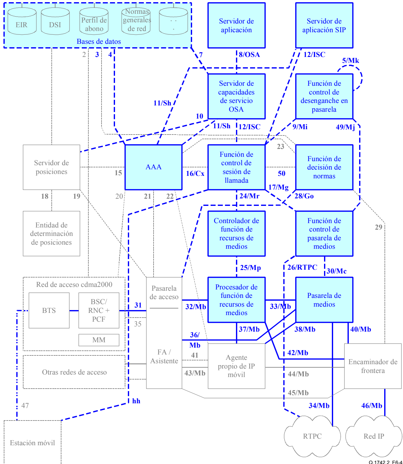
Figura 6-4/Q.1742.2 – Modelo de arquitectura del subsistema de sesión de multimedia IP de la red central desarrollada ANSI-41 con la red de acceso cdma2000
