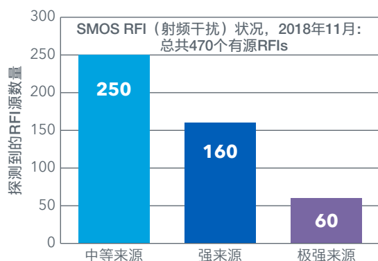
图2: SMOS辐射计在1400-1427 MHz无源频段探测到的RFI源数量的全球统计
