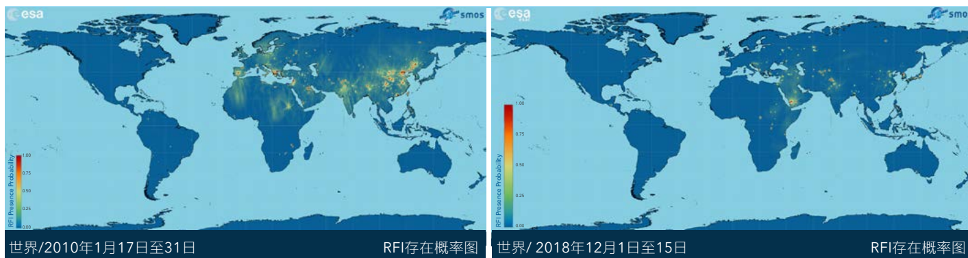
图1：SMOS RFI概率图，显示2010年至2018年间全球干扰源分布的改善
