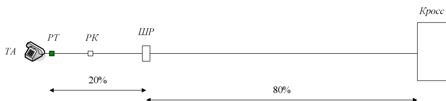
а) Модель эксплуатируемой сети доступа
