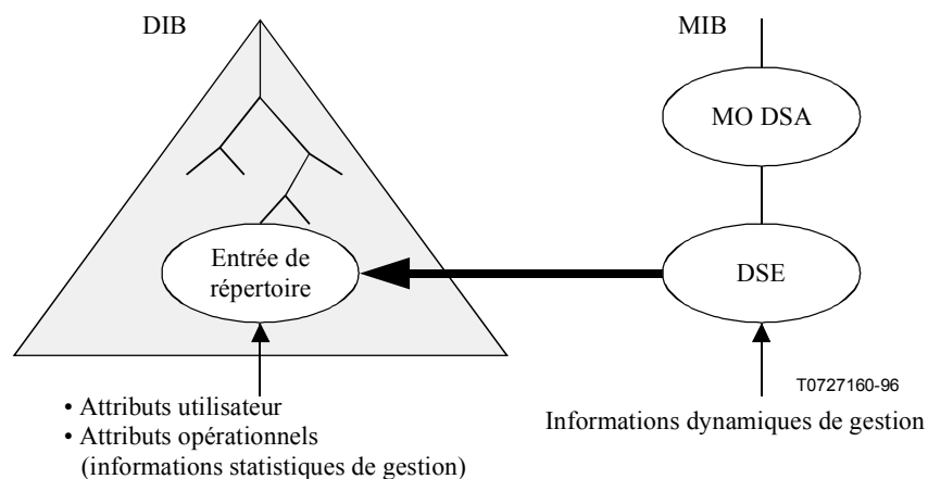
Figure 3 – Entrée gérée d'annuaire
