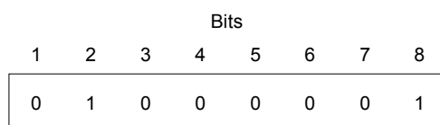
FIGURE 7/X.32 Sous-champ d'identificateur de format XID
