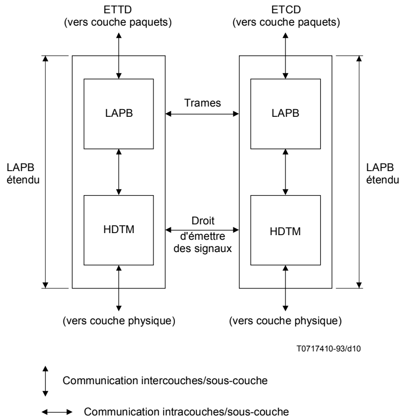
FIGURE 11/X.32 Couche liaison pour l'accès par RTPC basé sur le LAPB et le module de transmission en mode semi-duplex
