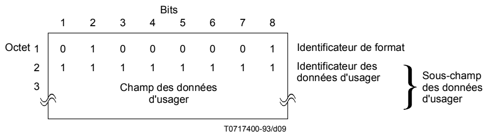
FIGURE 10/X.32 Format du champ d'information XID
