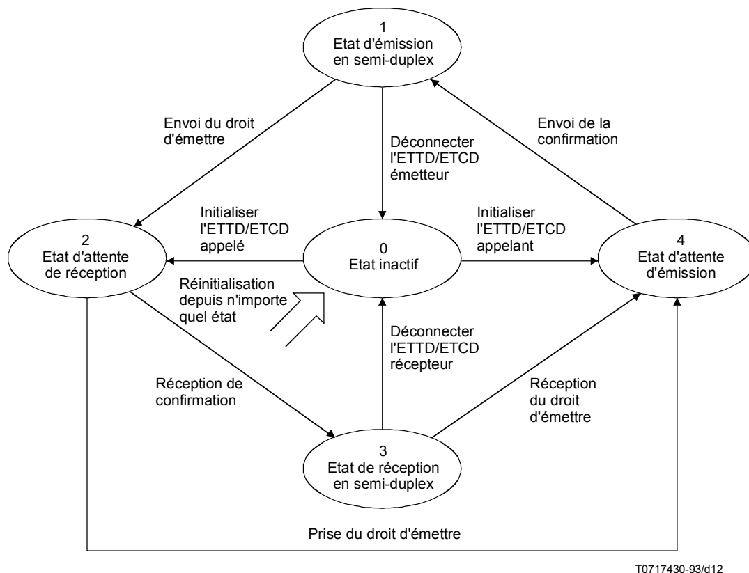
FIGURE 13/X.32 Diagramme d'états
