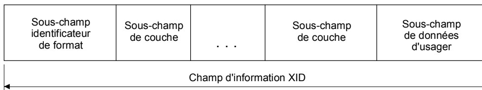
FIGURE 6/X.32 Structure générale du champ d'information XID
