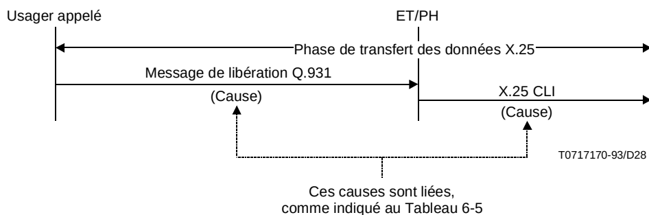
FIGURE III.13/X.31 Libération Q.931 pendant la phase de transfert des données X.25
