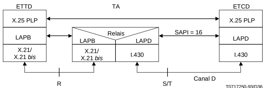
FIGURE IV.5/X.31 Exemple de configuration pendant la phase de transfert des données
