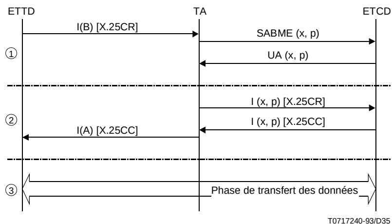
FIGURE IV.4/X.31 Séquence de messages Q.921 et X.25 pour un appel sortant déclenché par l'ETTD
