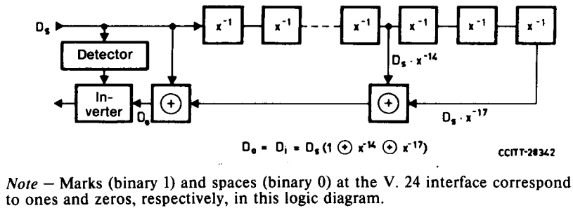
FIGURE 4/V.22 bis
