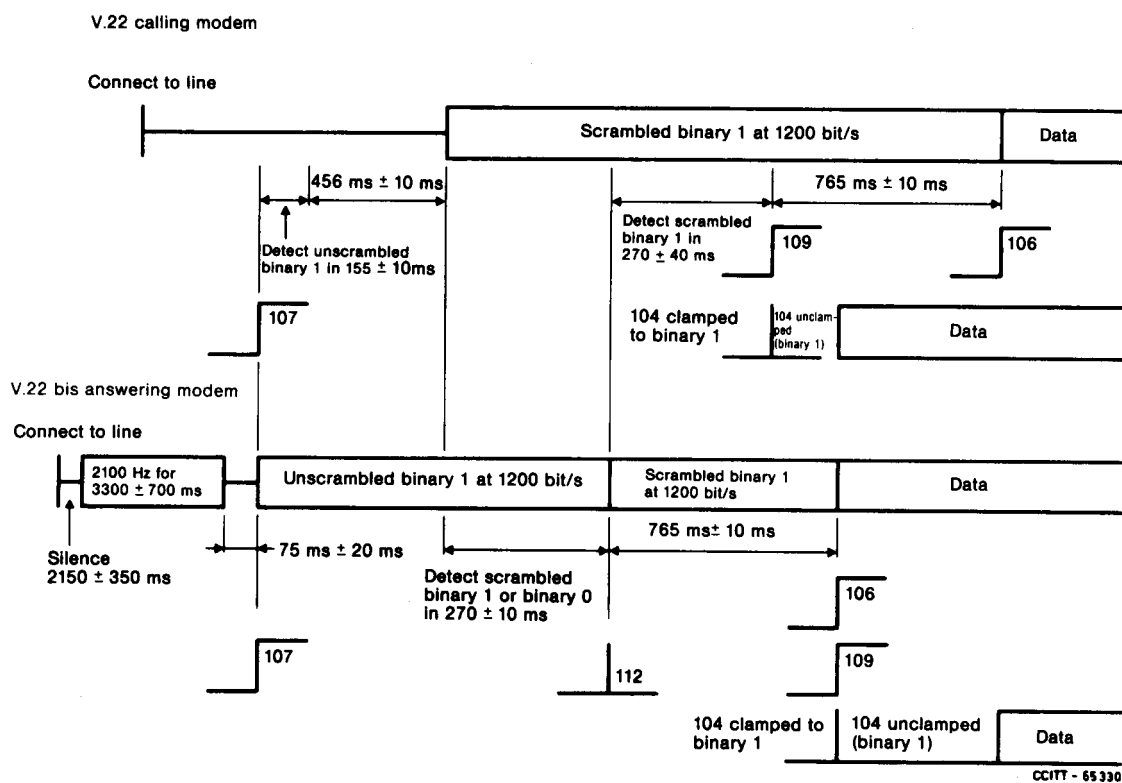
FIGURE 6/V.22 bis
