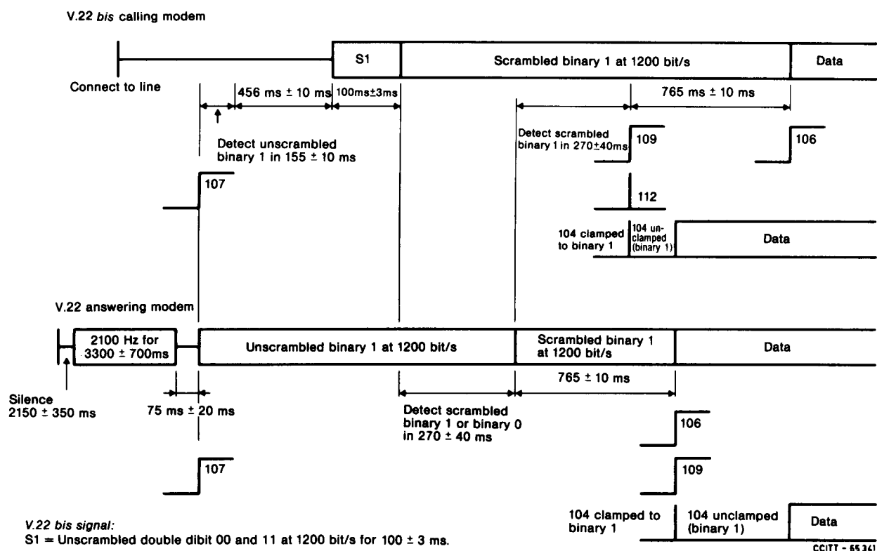
FIGURE 7/V.22 bis
