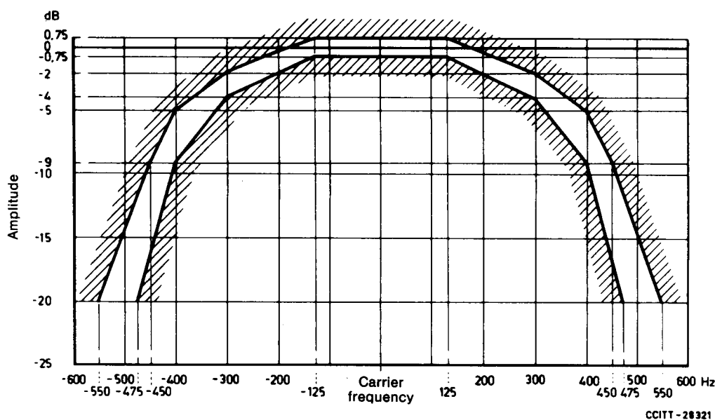
FIGURE 1/V.22 bis
