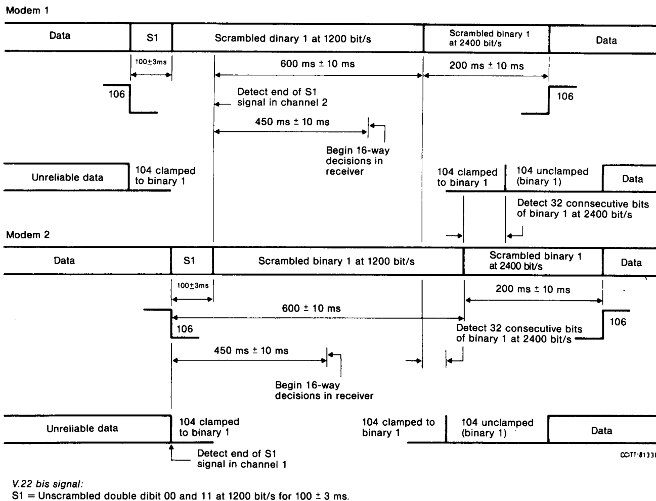
FIGURE 8/V.22 bis
