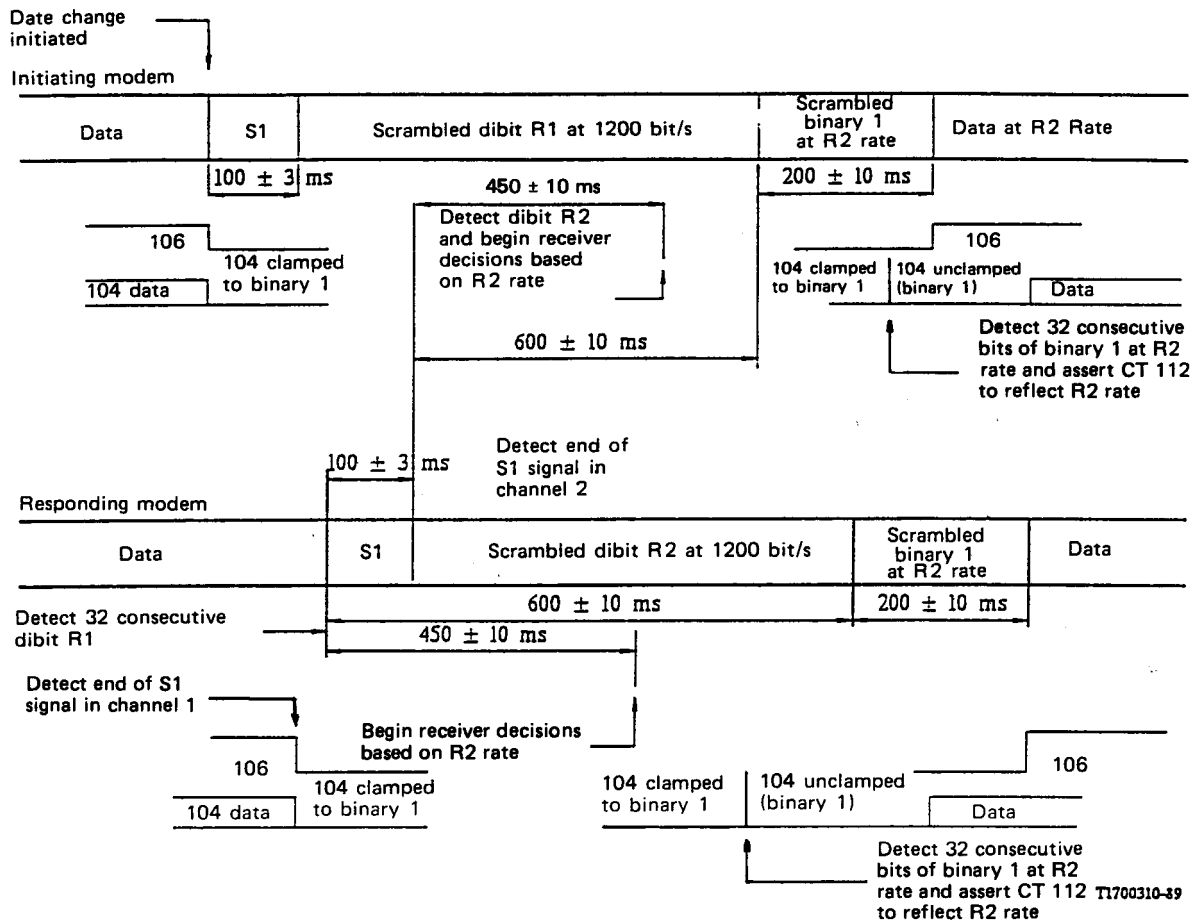
FIGURE 9/V.22 bis
