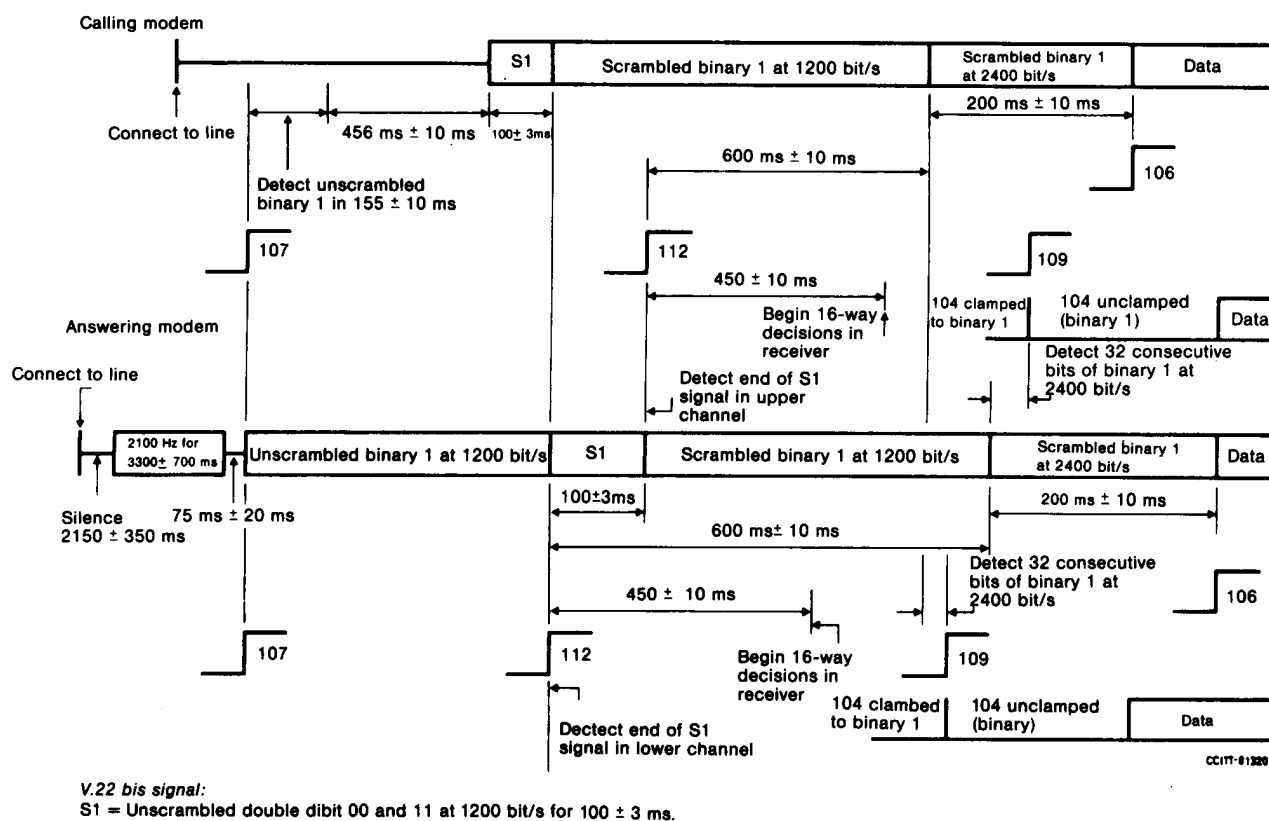
FIGURE 5/V.22 bis
