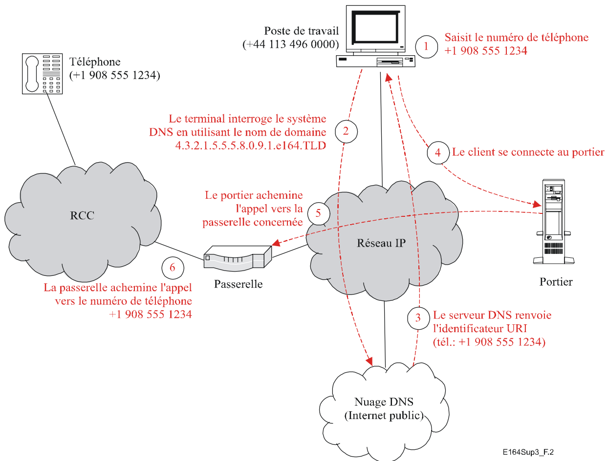
Figure 2 – Flux d'appel entre un réseau à commutation de circuits et un réseau basé IP – Exemple
