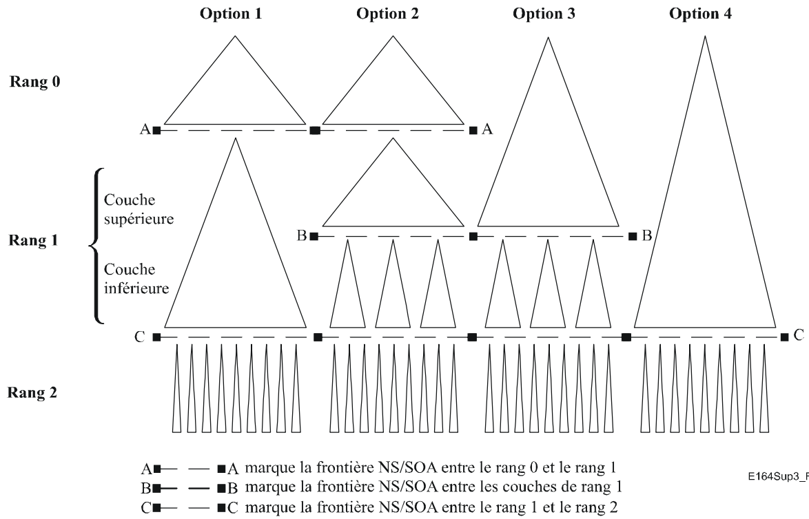
Figure B.2 – Exemples de variantes pour les délégations de zones faisant intervenir le rang 1 ENUM
