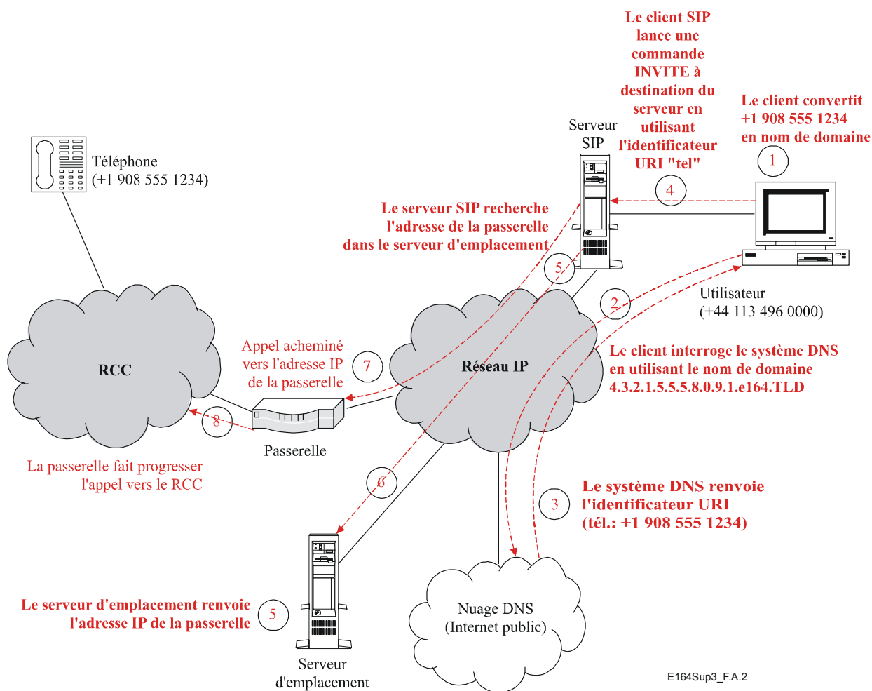
Figure A.2 – Flux d'appels types: IP vers RTPC
