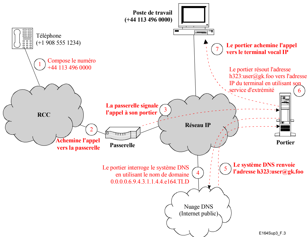
Figure 3 – Flux d'appel entre un réseau basé IP et un réseau à commutation de circuits – Exemple
