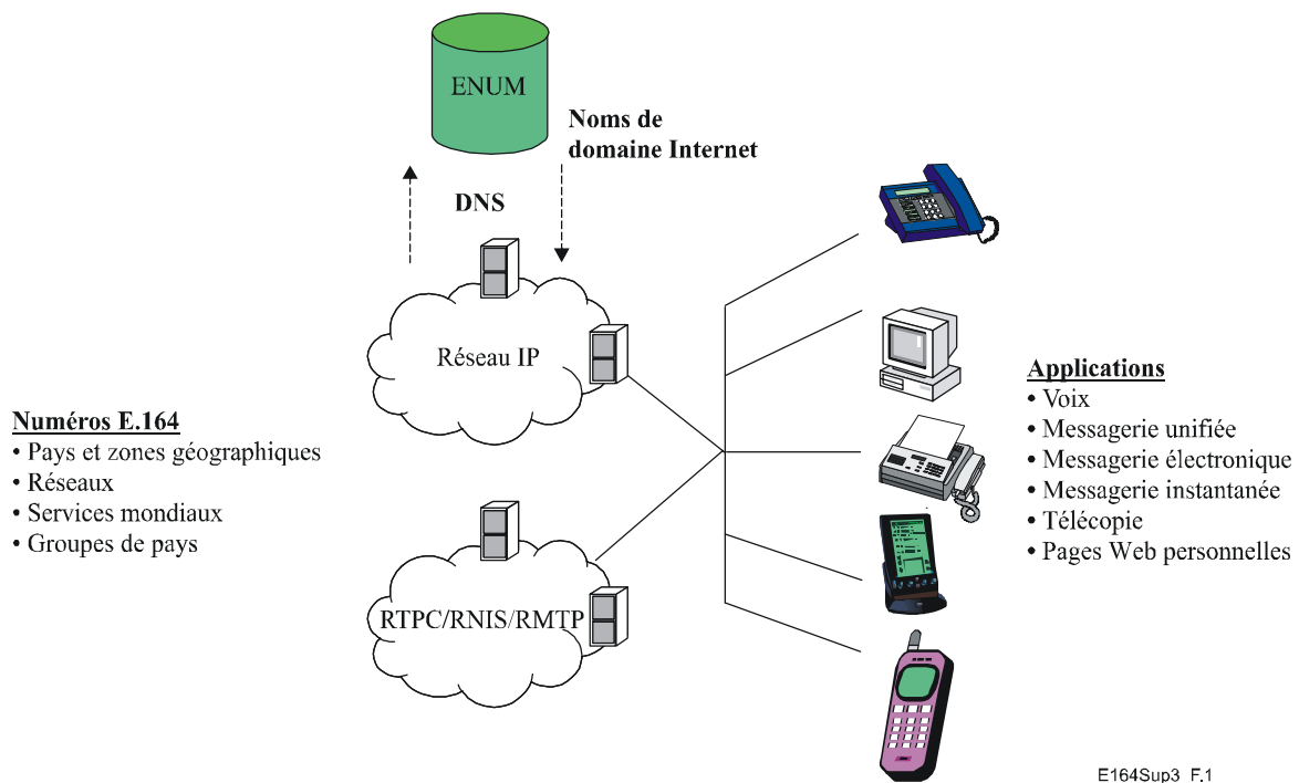
Figure 1 – Applications pouvant être associées à des numéros E.164
