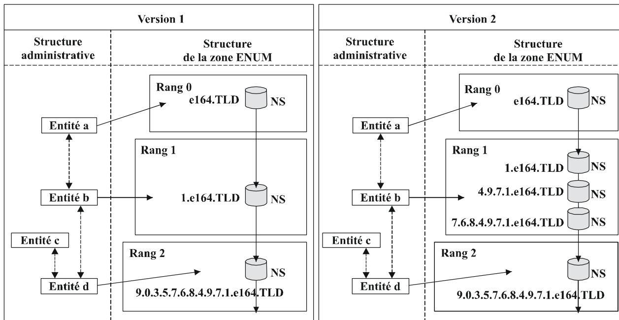
Figure 5 – Exemples de relations possibles entre une structure administrative et des structures de zone ENUM
