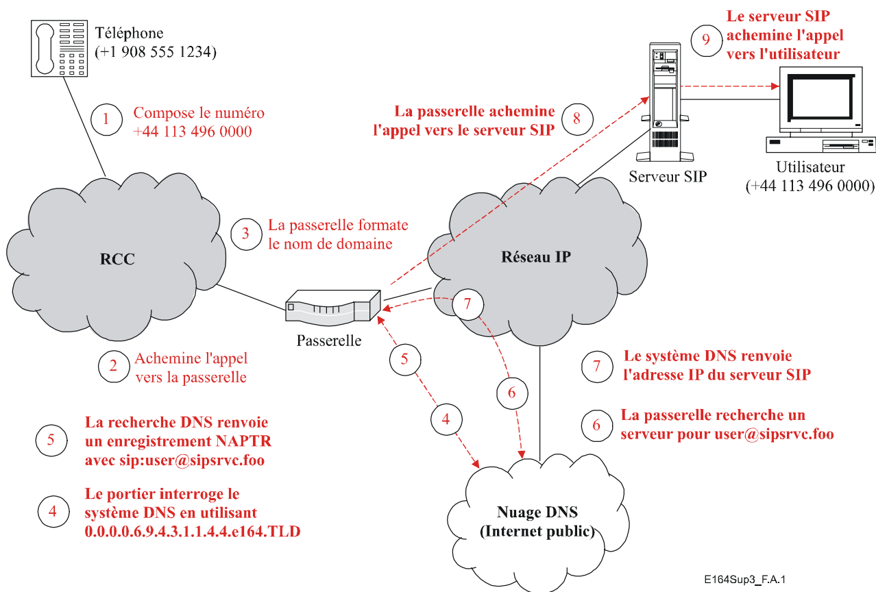
Figure A.1 – Flux d'appels types: RTPC vers IP
