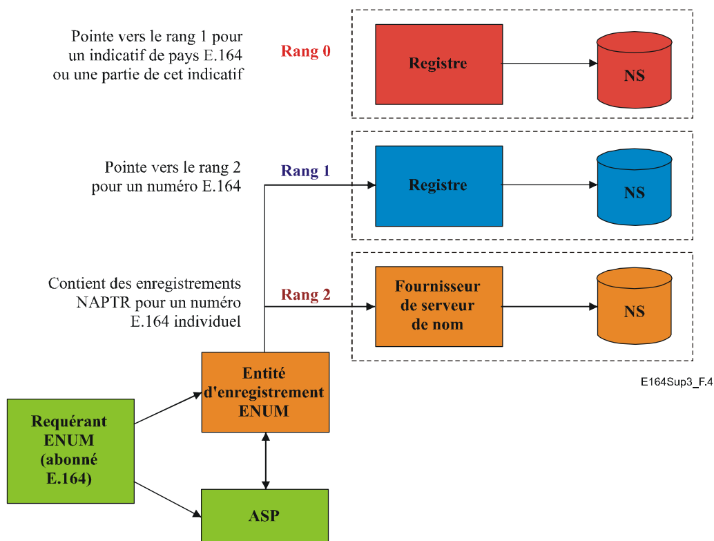
Figure 4 – Insertion de numéros E.164 dans le système DNS
