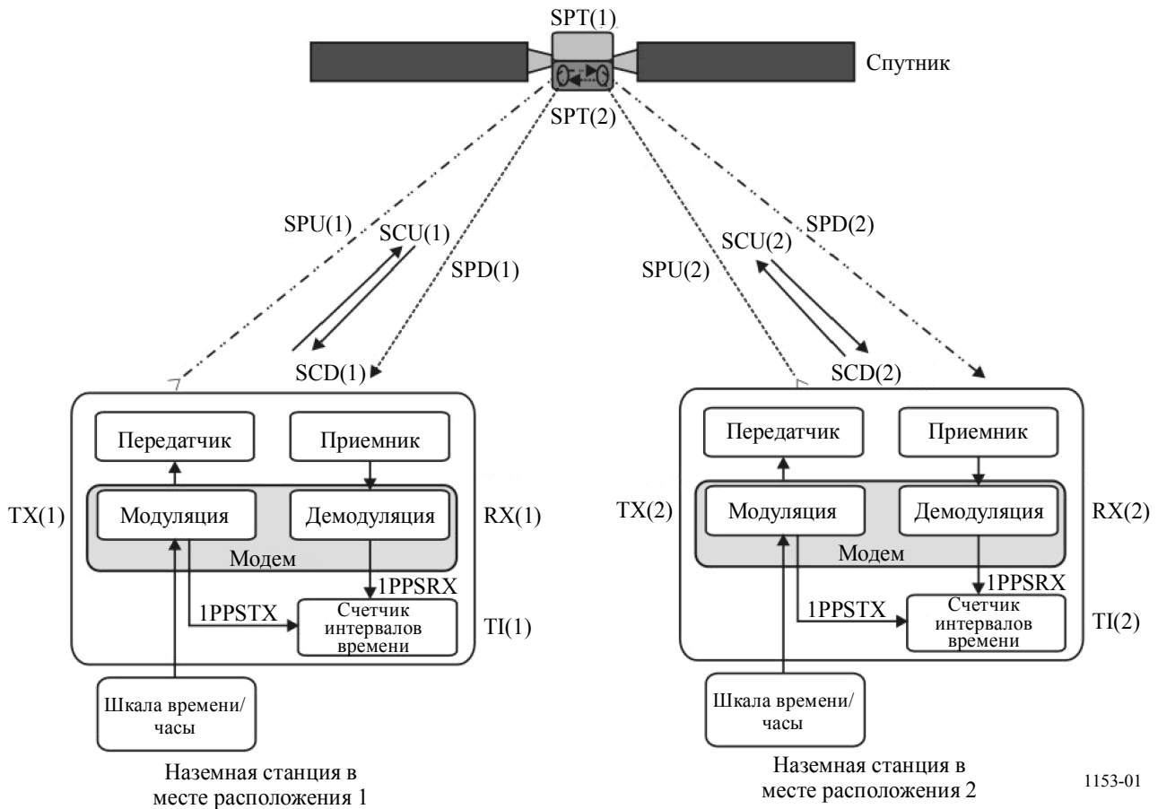
РИСУНОК 1 Принцип TWSTFT
