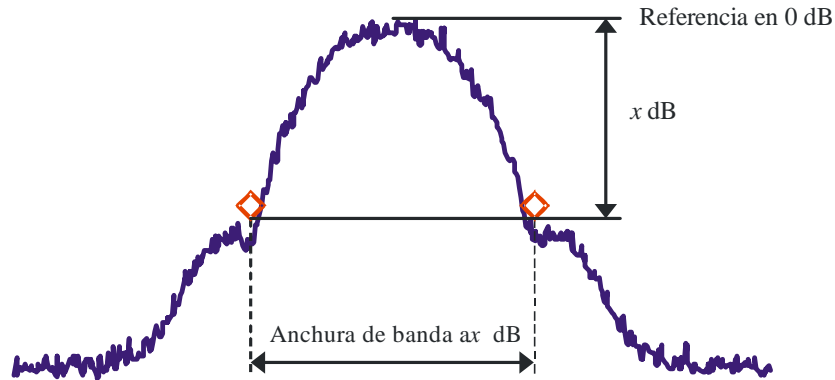
FIGURA 3 Anchura de banda entre puntos a x dB
