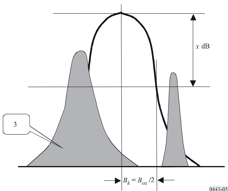
РИСУНОК 5 Измерение ширины полосы по половинному спектру
