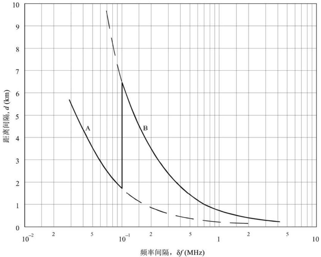
两信号三阶接收机互调干扰分析的 FD 规则
