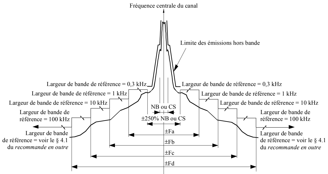
Gabarit générique des rayonnements non essentiels pour des stations du service fixe relevant de la catégorie B (voir le Tableau 11)
