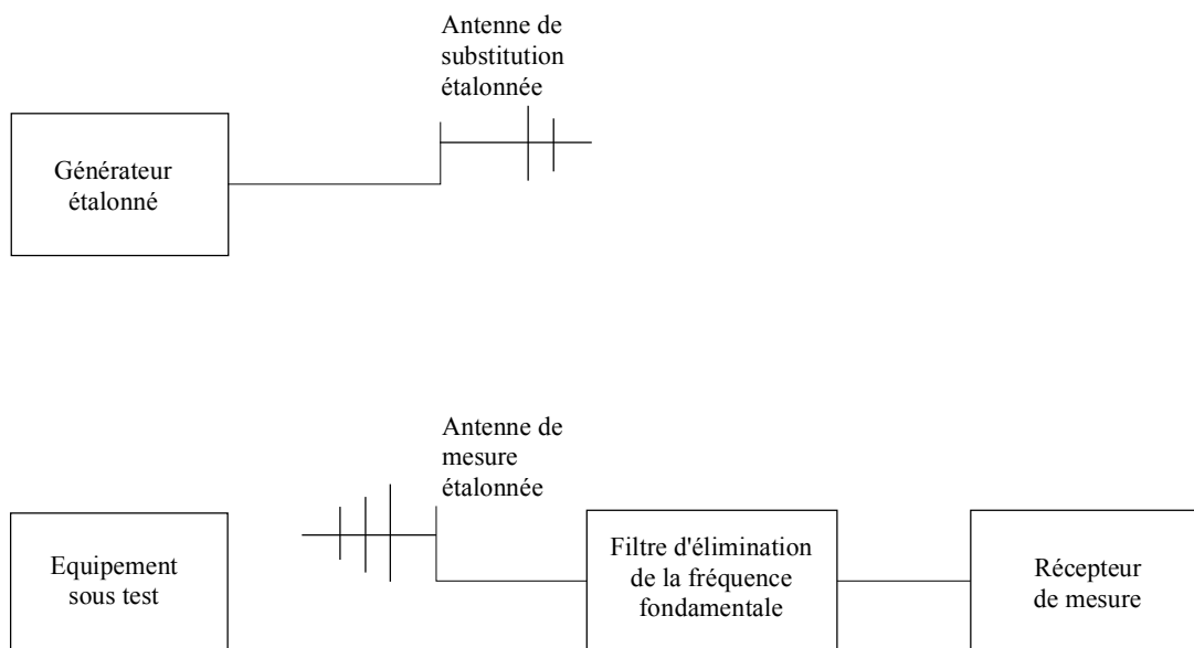
FIGURE 2 Montage pour la mesure de la p.i.r.e. des rayonnements non essentiels
