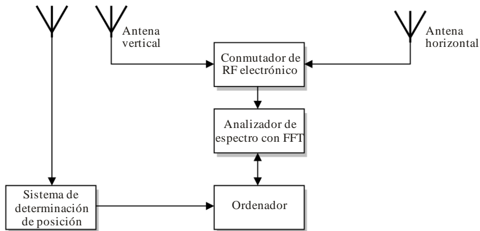
FIGURA 9 Montaje de medición (recepción portátil en las SFN)
