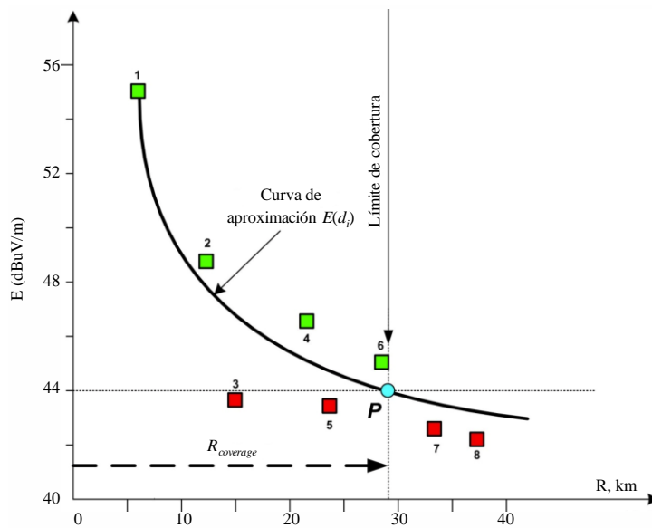
FIGURA 19 Ejemplo de procesamiento de los resultados de medición en una única dirección radial
