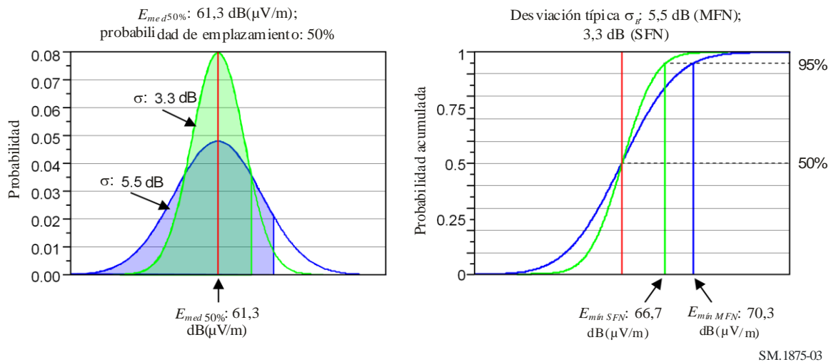
FIGURA 3 Ganancia de red
