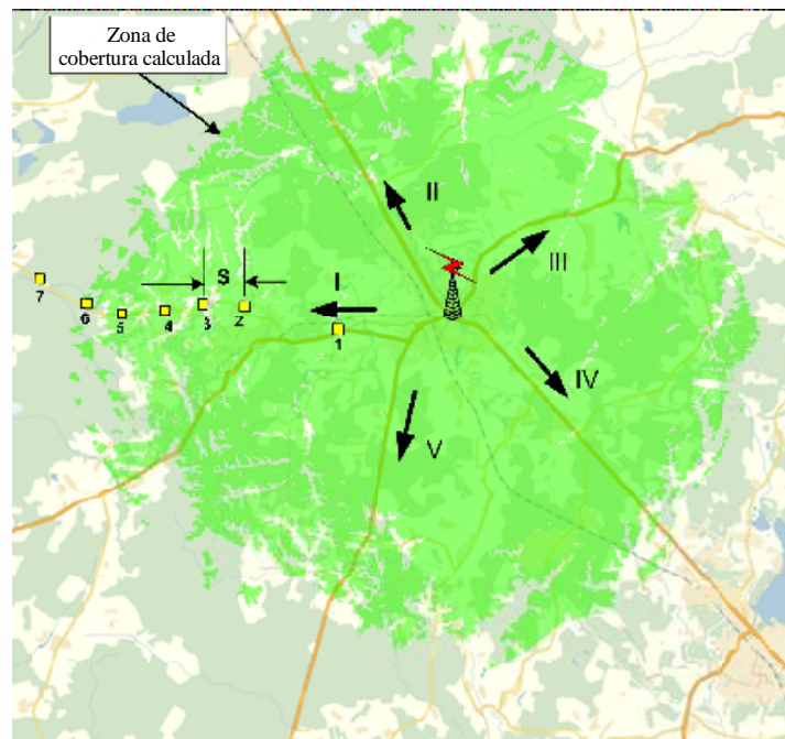
FIGURA 16 Ejemplo de planificación de la medición
