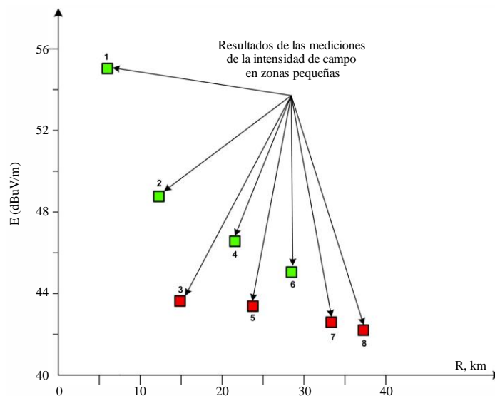
Ejemplo de los resultados de medición obtenidos en una única dirección radial
