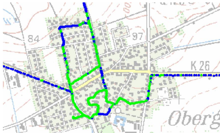
FIGURA 13 Resultados de la medición (recepción portátil)
