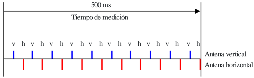
FIGURA 11 Temporización de las mediciones para SFN con polarización mixta (recepción portátil)
