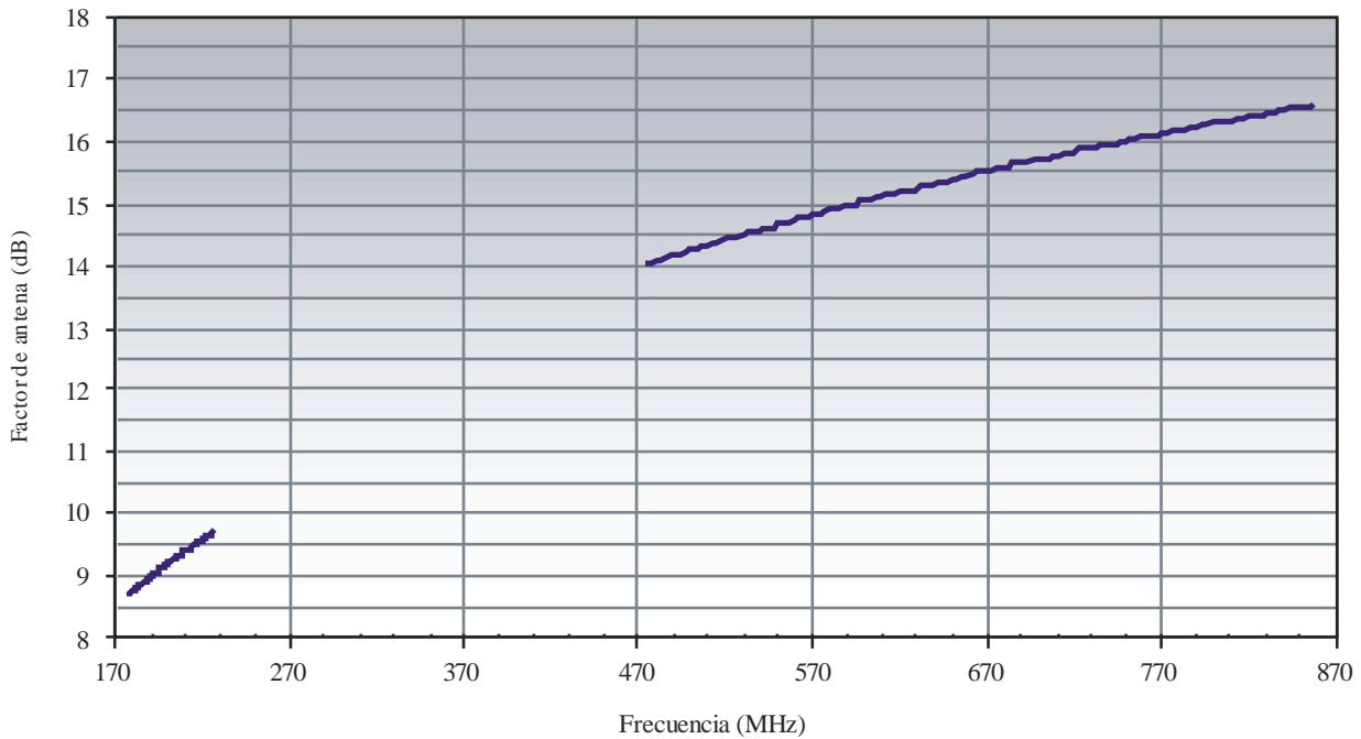
FIGURA 2 Factor de antena para la recepción de radiodifusión fija
