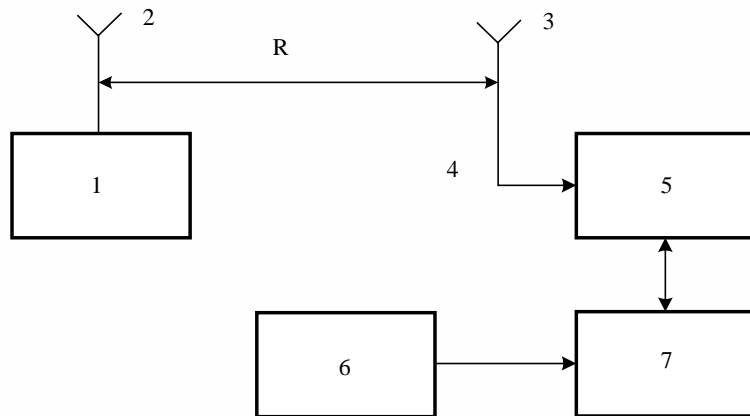
FIGURA 15 Diagrama de conexión de los equipos
