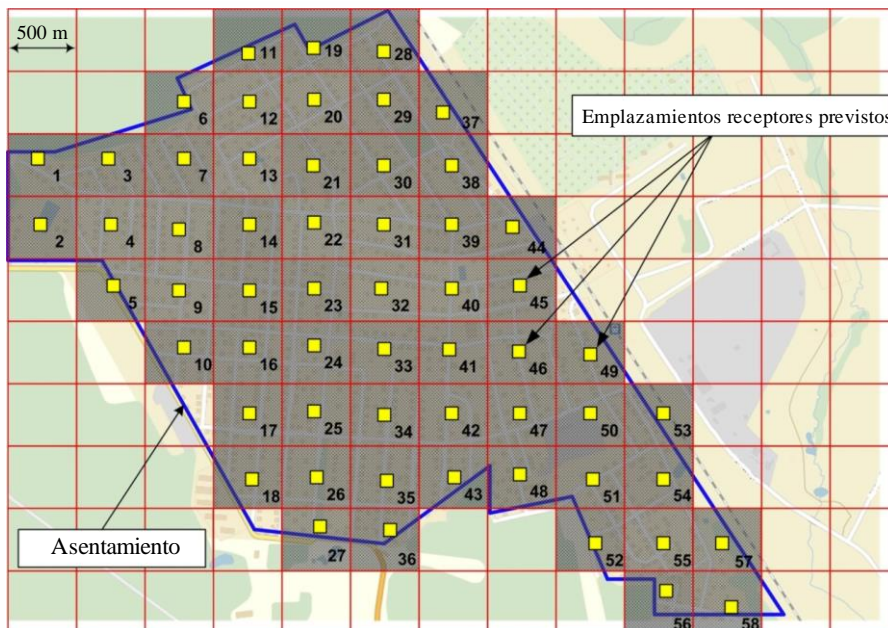
FIGURA 23 Ejemplo de proyección de retícula de prueba
