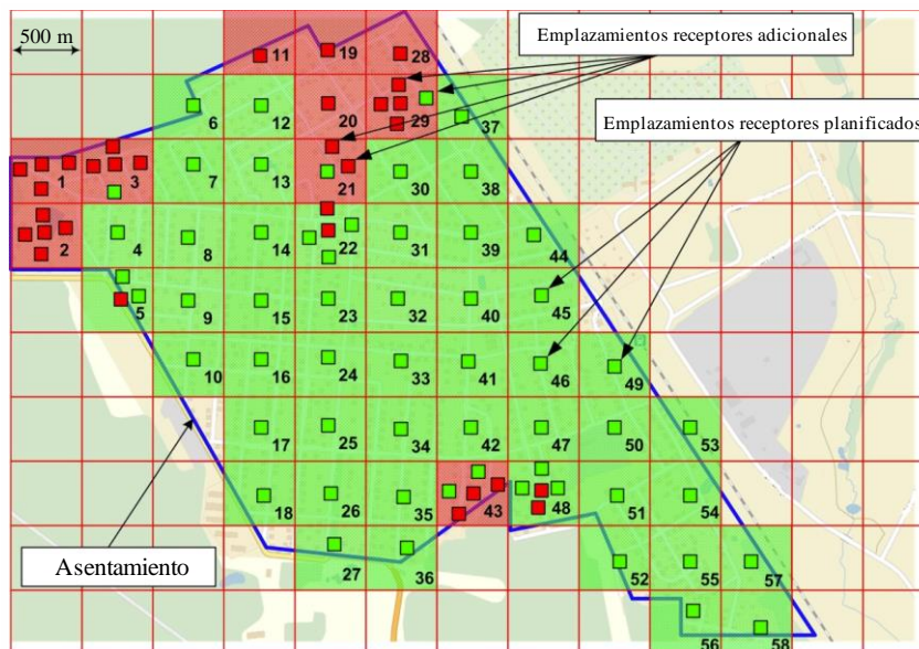
FIGURA 24 Ejemplo de visualización de los resultados de la medición
