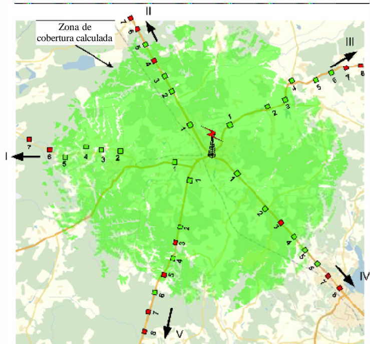
Ejemplo de resultados de medición en zonas pequeñas
